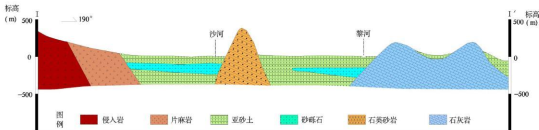
图 5.5-2 区域水文地质剖面图
