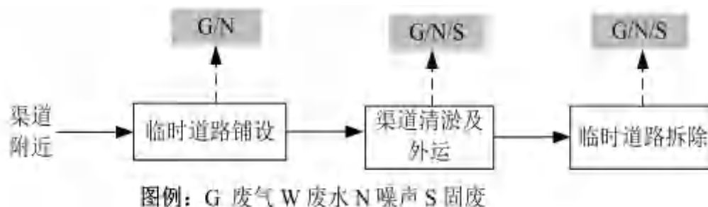
图3.11-2 渠道清淤施工工艺流程及产排污节点图
