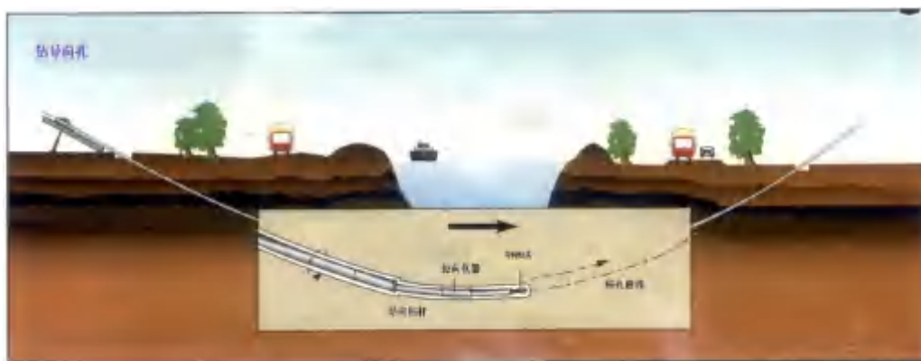
钻导向孔示意图
