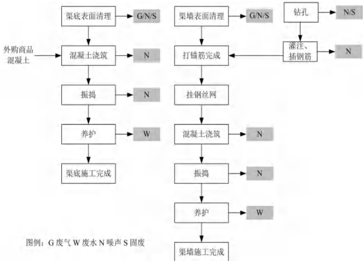
图 3.11-4 渠道挂网混凝土衬砌施工工艺流程及产排污节点图
