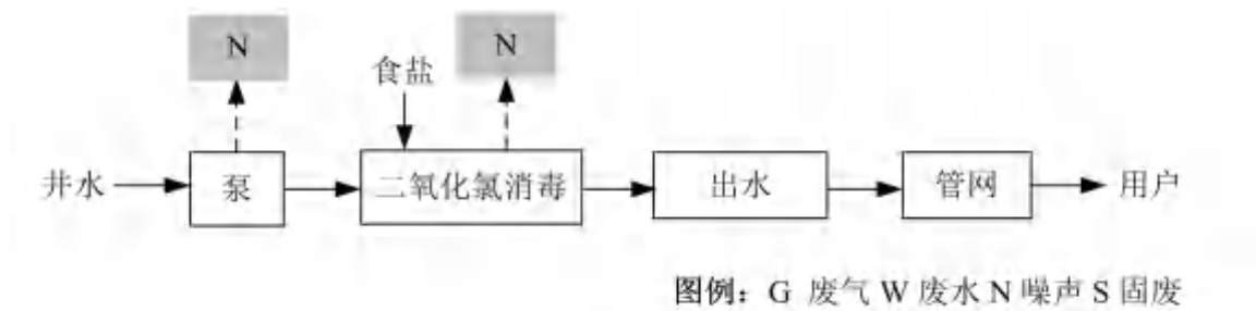
图3.12-1 导流施工工艺流程及产排污节点图
