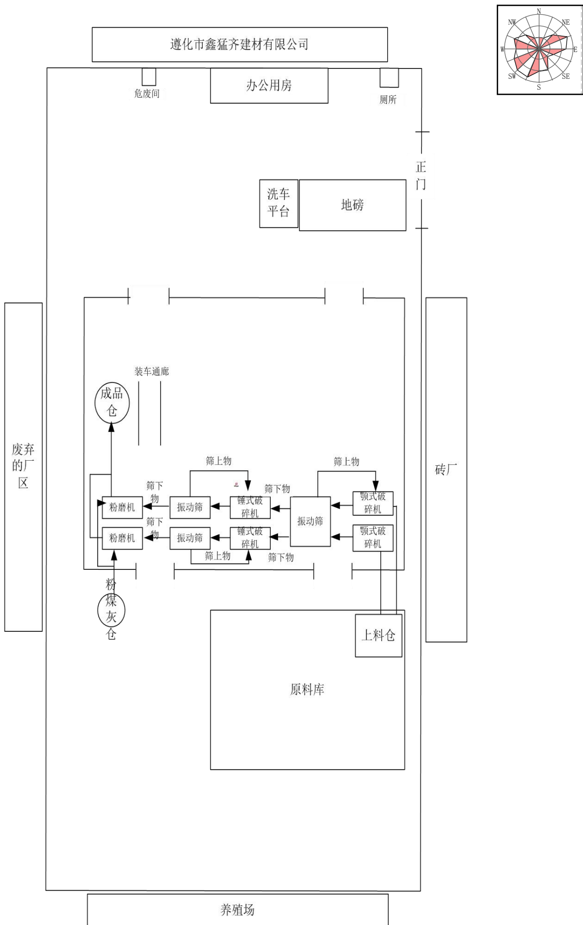
附图 2 平面布置及周边关系图 比例尺 1:700
