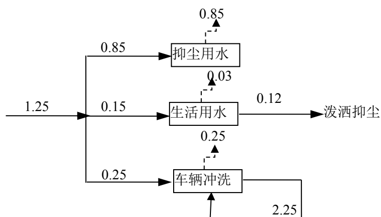
图2 本项目给排水平衡图
