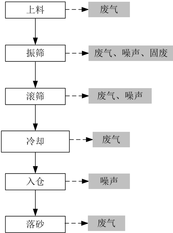
图 2-3 砂处理工艺流程及排污节点图
