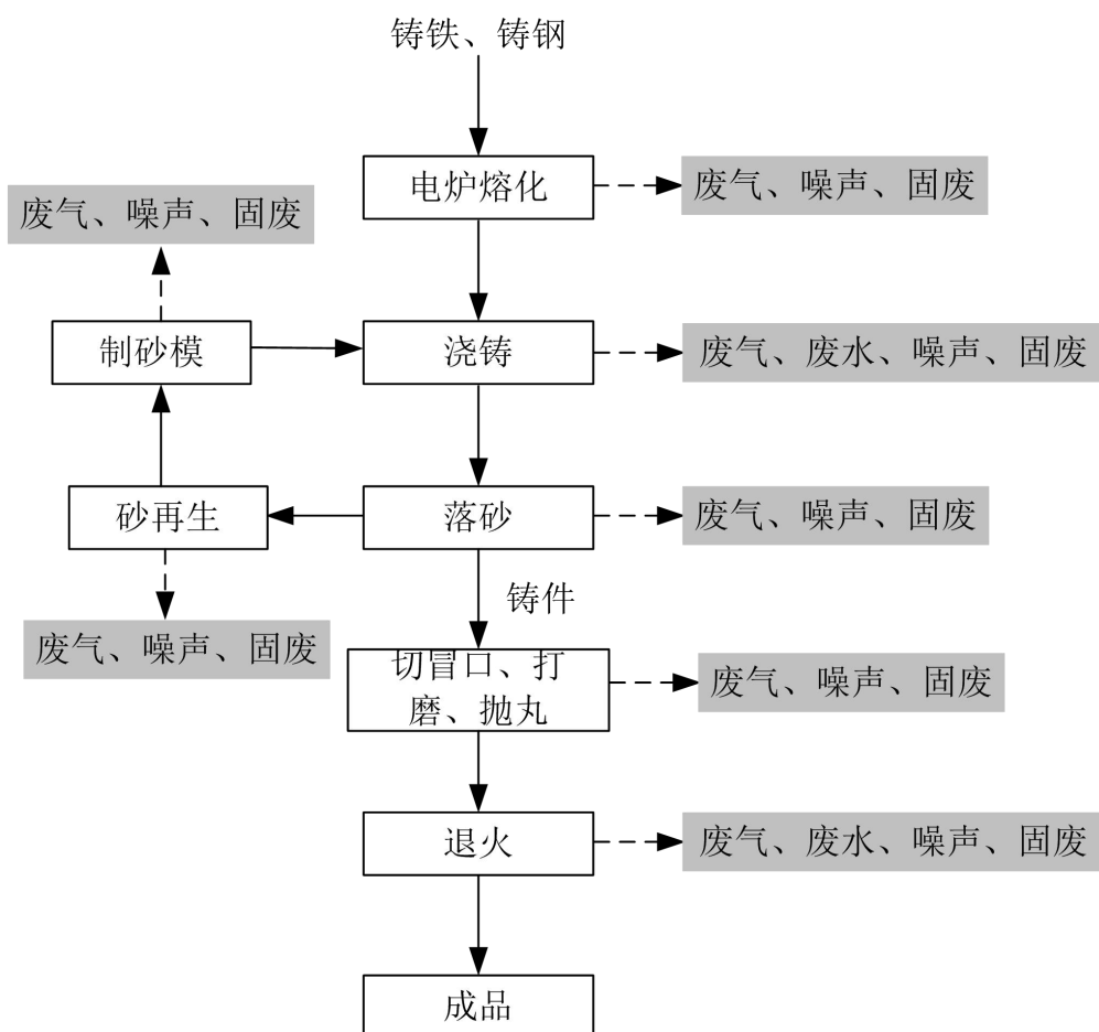
图 2-2 生产工艺流程及排污节点图
