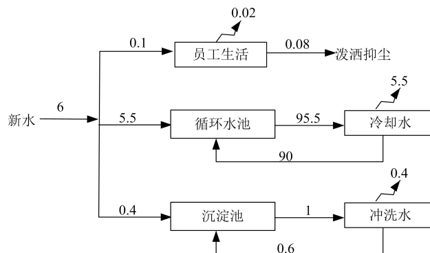
图 2-1 本项目给排水平衡图 单位: \text{m}^3/\text{d} 表 2-6 本项目水量平衡表 单位: \text{m}^3/\text{d}
