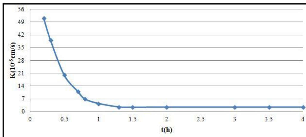
图 5.2-8 厂区北侧试验点渗透系数与时间关系曲线图
