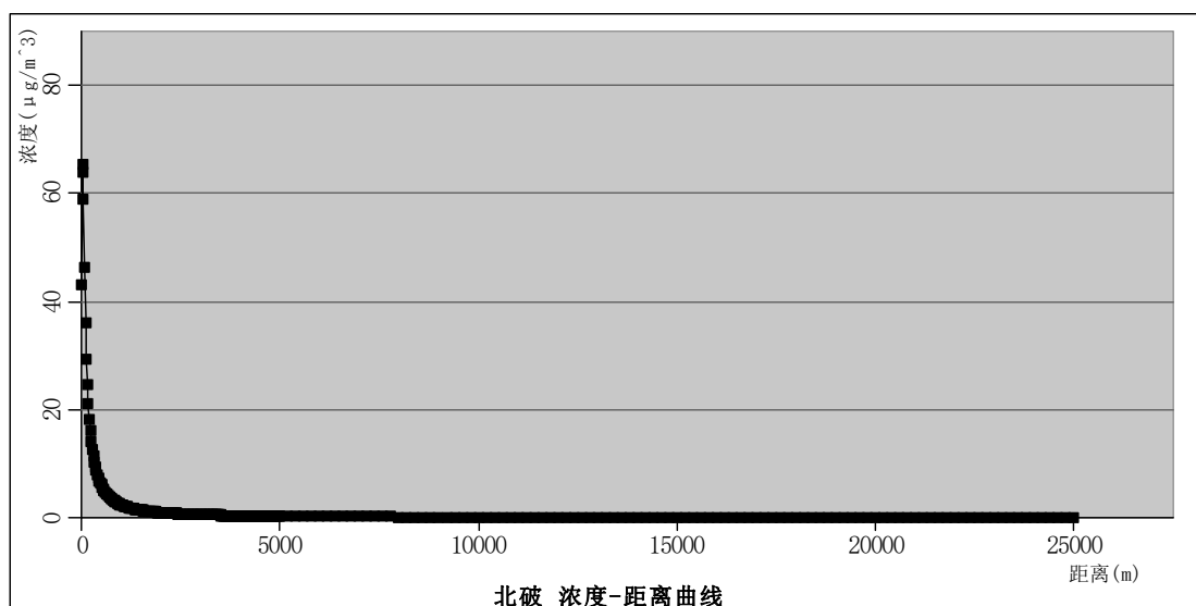
图 5.2-5 南厂区破碎车间无组织废气浓度距离曲线图 \mu\text{g}/\text{m}^3
