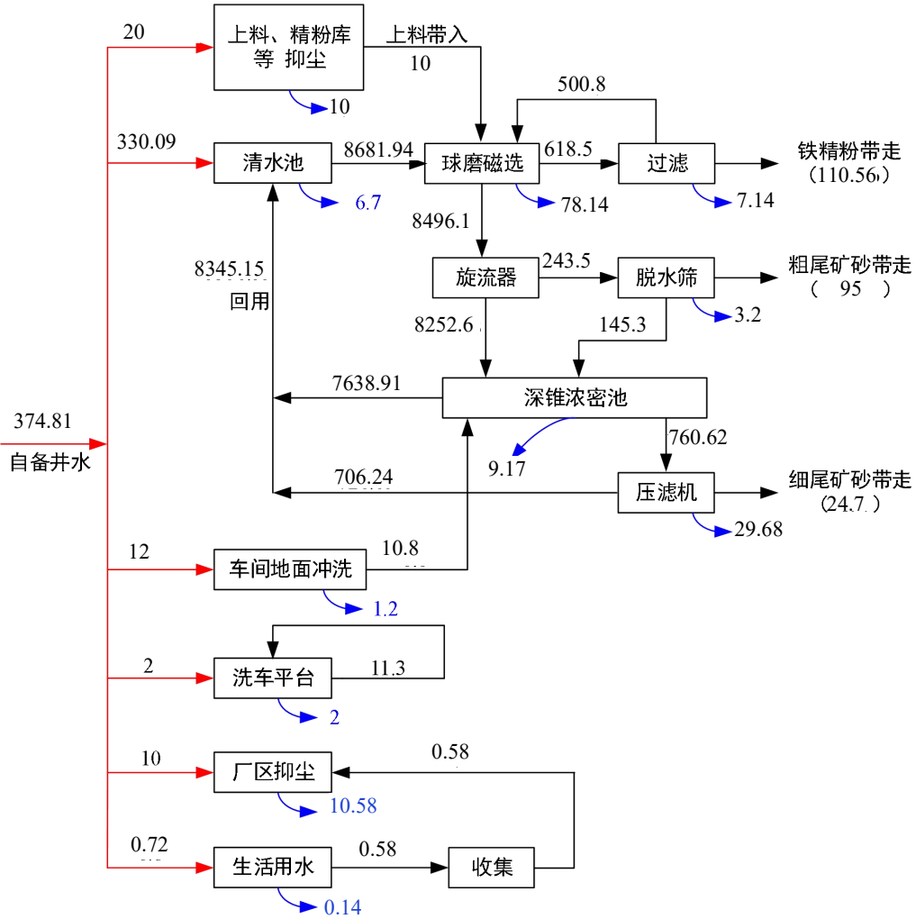
图 3.2-1 改扩建实施后全厂水平衡图
