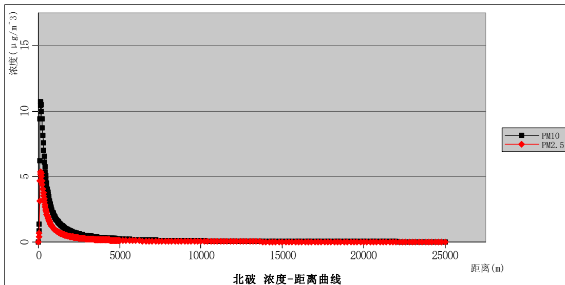
图 5.2-2 北厂区破碎线有组织废气浓度距离曲线图 \mu\text{g}/\text{m}^3
