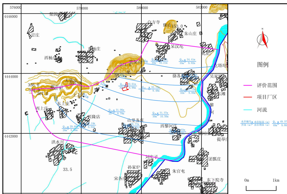
图 5.2-9 项目区域等水位线图
