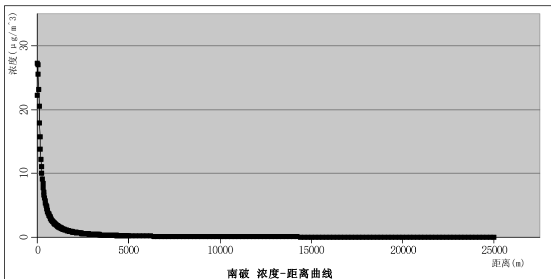
图 5.2-4 北厂区原料库无组织废气浓度距离曲线图 \mu\text{g}/\text{m}^3
