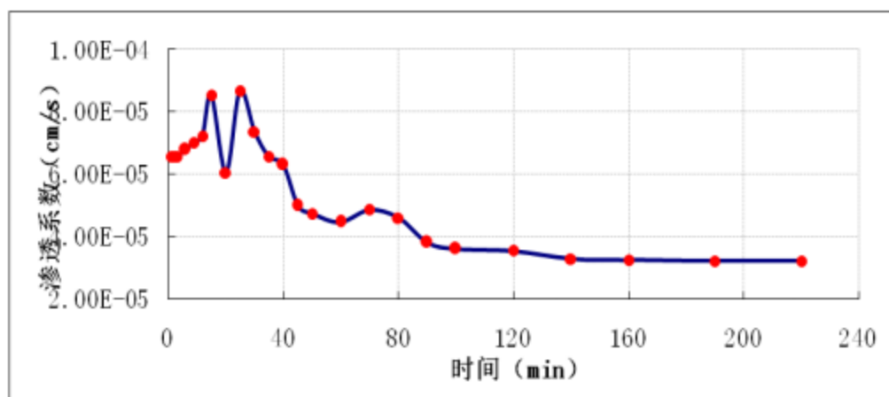
图 5.2-18 S-1 渗水试验成果图
