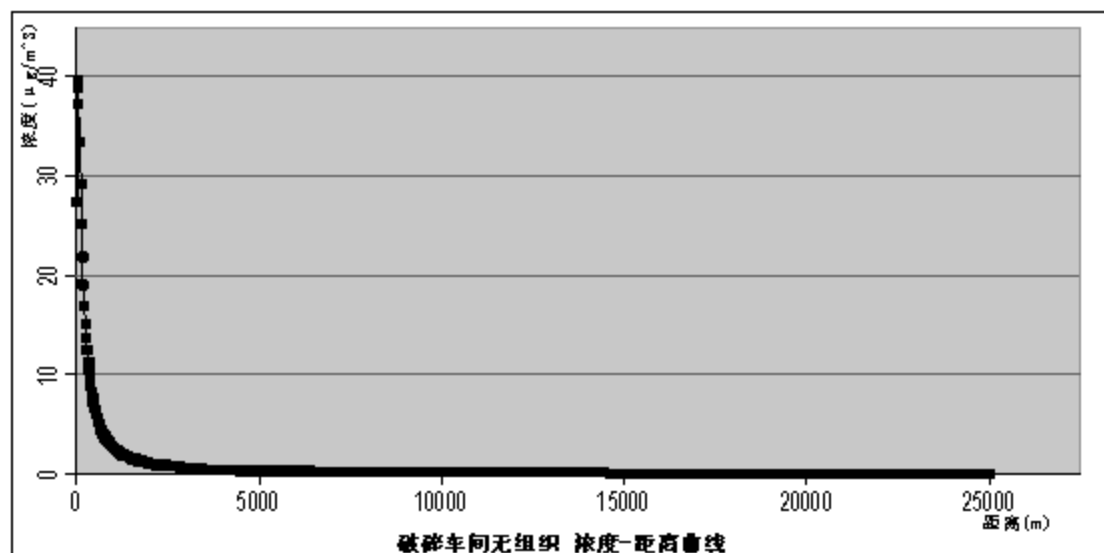
图 5.2-3 破碎车间无组织废气浓度距离曲线图 \mu\text{g}/\text{m}^3
