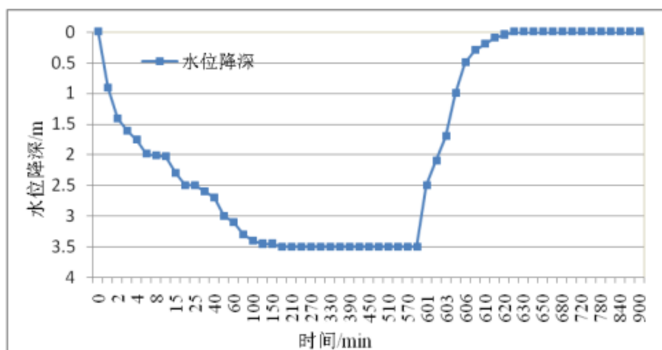
图5.2-11 般若院村抽水试验降深-时间曲线
