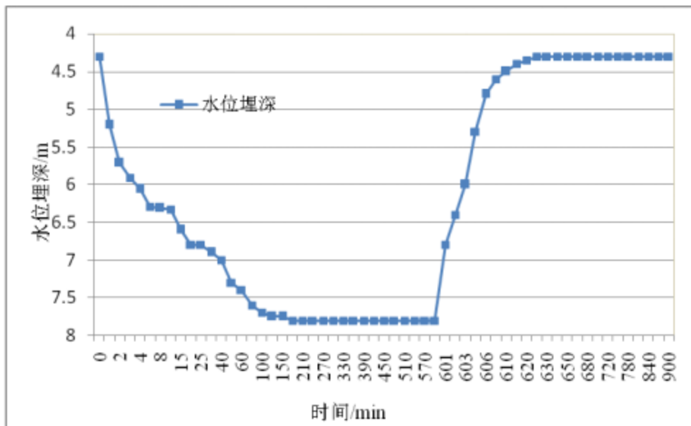
图5.2-12 般若院村抽水试验水位埋深-时间曲线
