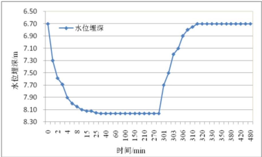
图5.2-15 上石河村抽水试验水位降深-时间曲线
