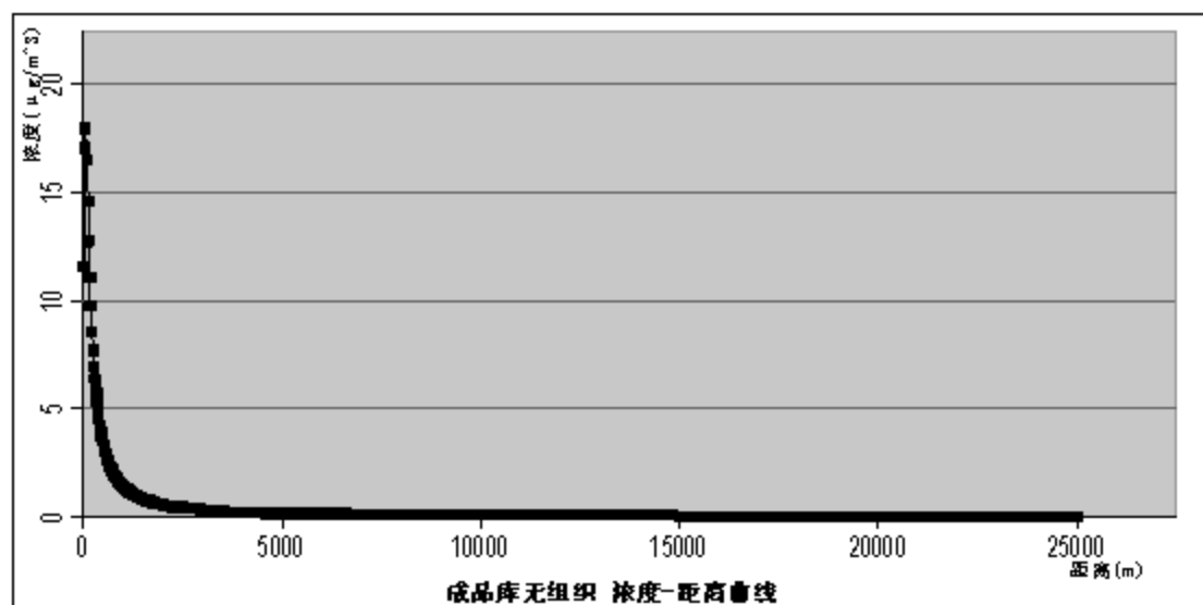
图 5.2-2 成品库无组织废气浓度距离曲线图 \mu\text{g}/\text{m}^3
