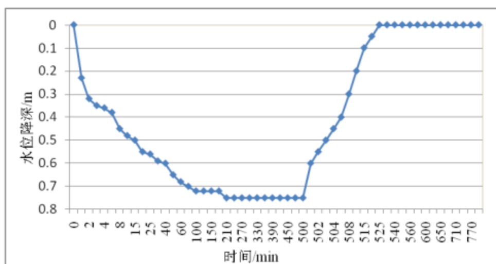
图 5.2-13 东桃园村东抽水试验水位降深-时间曲线
