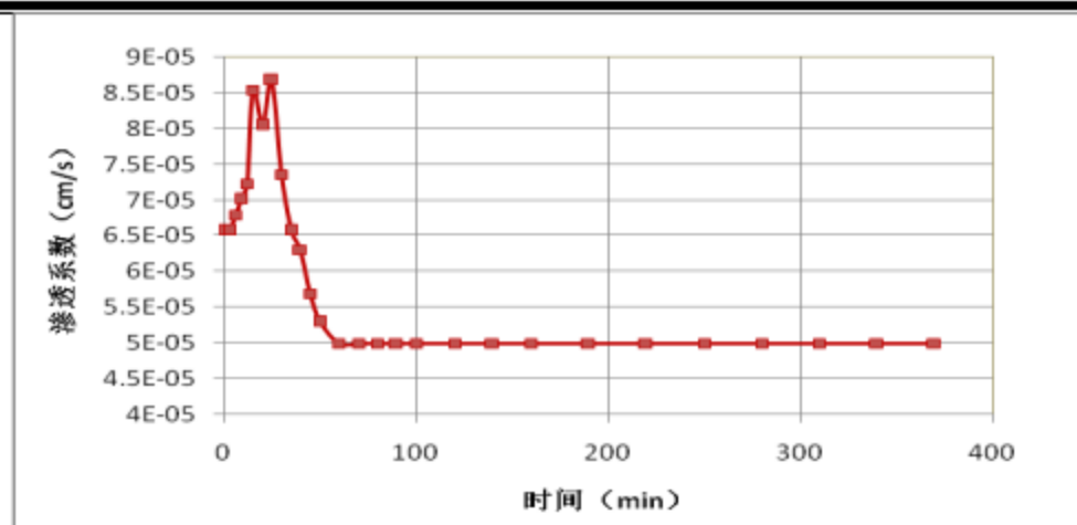
图 5.2-20 S-3 渗水试验成果图
