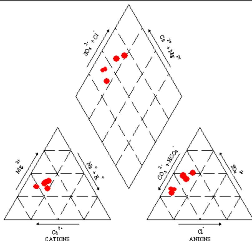
图 5.2-8 评价区水化学类型 piper 图
