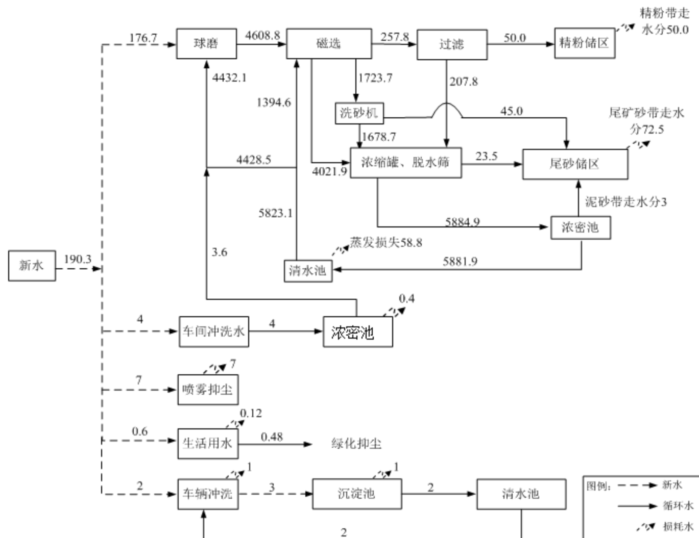
图 3.2-1 项目给排水平衡图 单位: \text{m}^3/\text{d}
