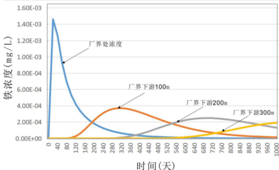
图 5.2-21 厂界、距厂界 100 米、200 米、300 米处铁浓度随时间变化过程线
