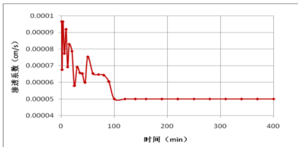
图 5.2-19 S-2 渗水试验成果图
