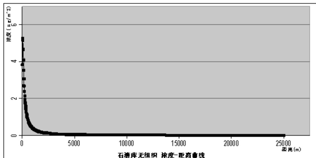
图 5.2-4 石渣库无组织废气浓度距离曲线图 \mu\text{g}/\text{m}^3
