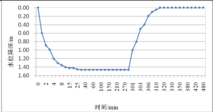
图5.2-15 上石河村抽水试验水位降深-时间曲线
