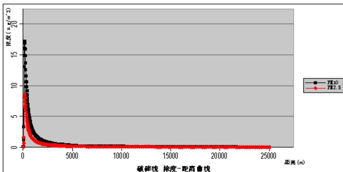
图 5.2-1 破碎线有组织废气浓度距离曲线图 \mu\text{g}/\text{m}^3
