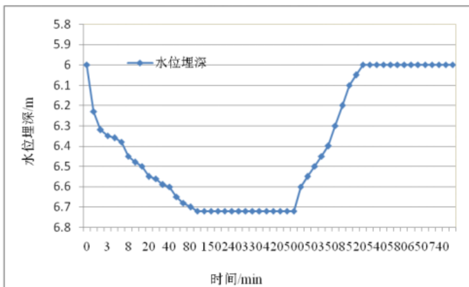
图 5.2-14 东桃园村东抽水试验水位埋深-时间曲线
