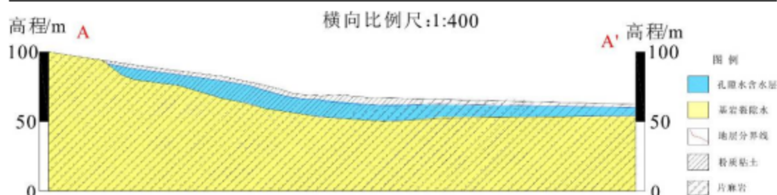
图 5.2-6 区域地质剖面图
