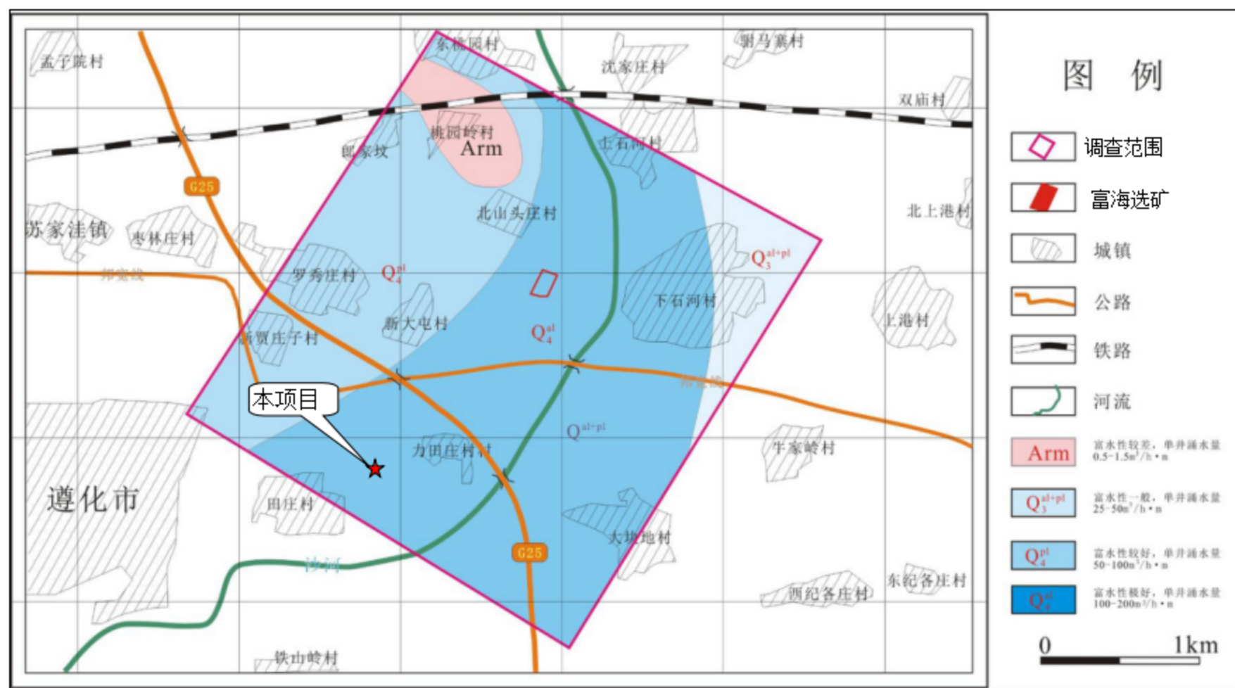
图 5.2-7 区域水文地质图
