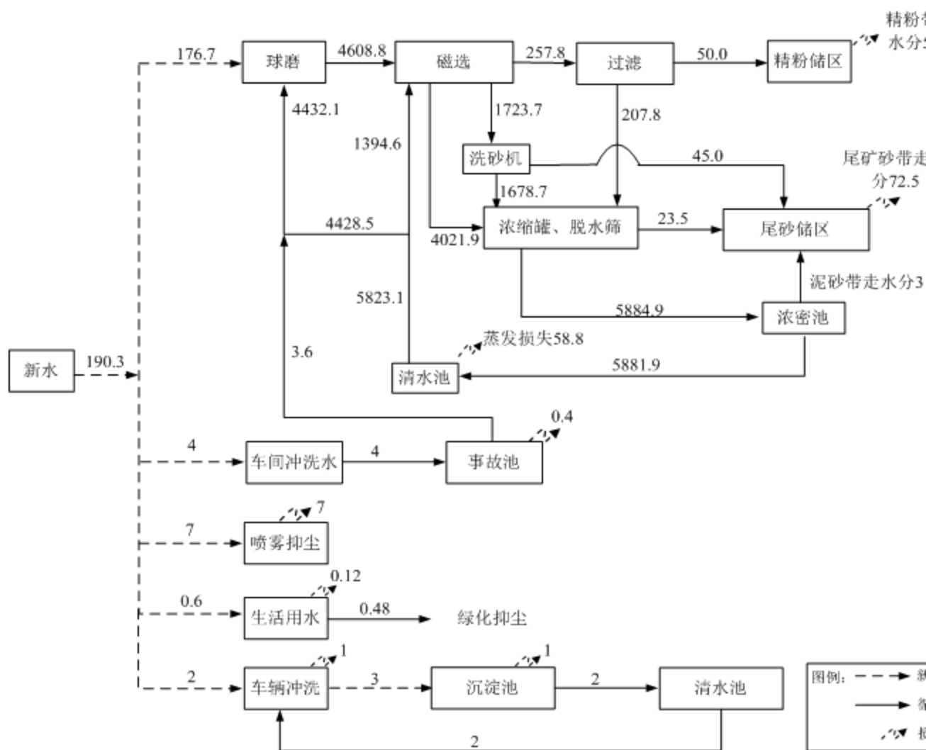
图 3.2-1 项目给排水平衡图 单位: \text{m}^3/\text{d}
