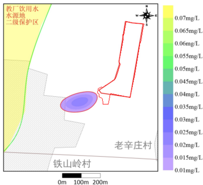
B. 300 天影响预测图
