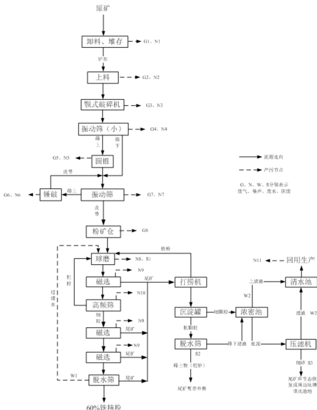
图 3.2-1 现有工程生产工艺流程及产排污节点图
