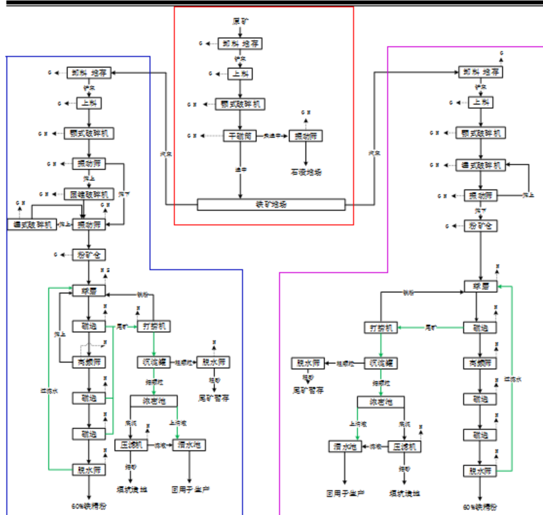
1#生产线，现有工程（厂区南侧） 2#生产线，扩建工程（厂区中部） 3#生产线，扩建工程（厂区北侧）
