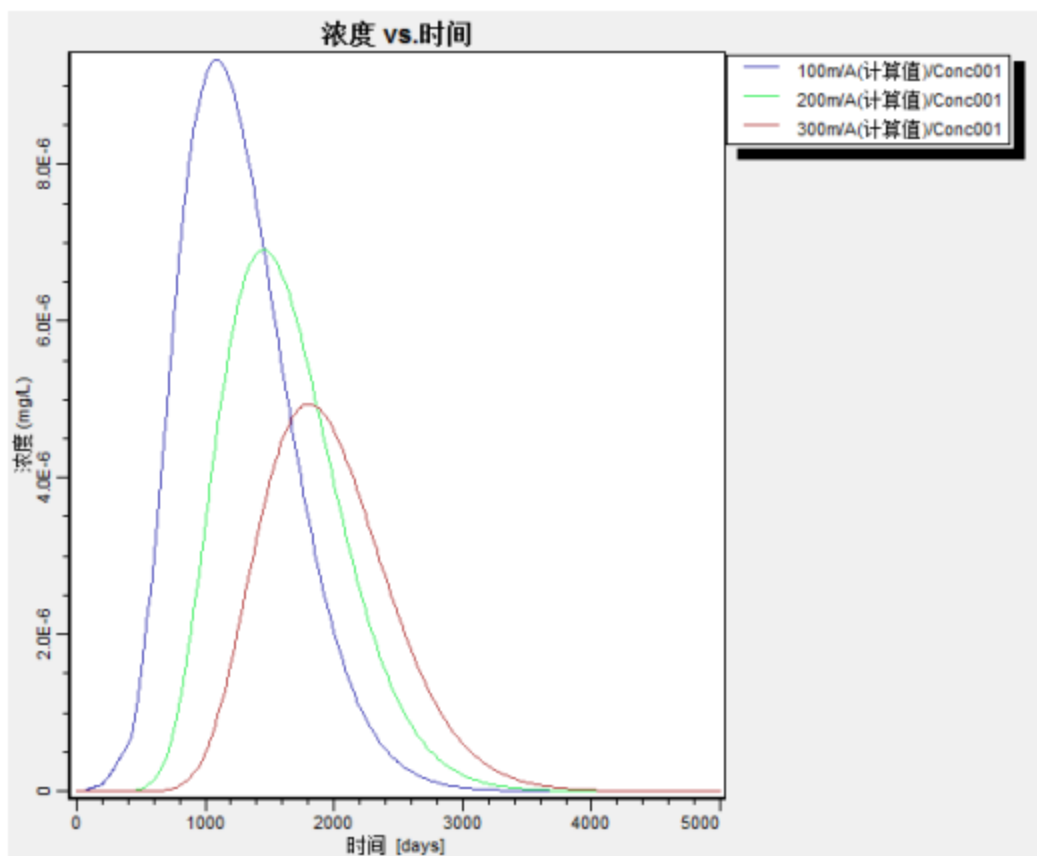
图 5.2-18 距离污染泄漏点 100 米，200 米和 300 米处铁浓度随时间变化过程线
