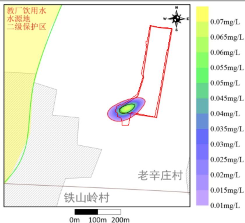
A. 100 天影响预测图
