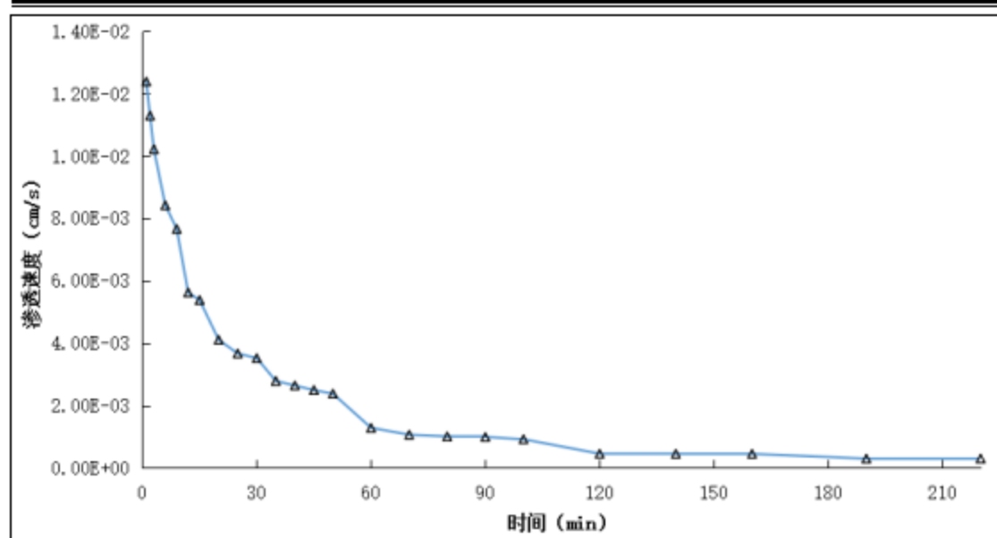
图 5.2-9 S1 渗水试验成果图
