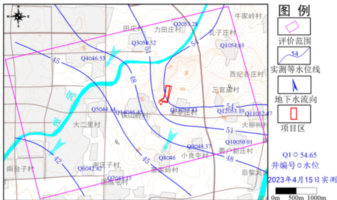
图 5.2-7 2023 年 4 月 15 日实测地下水流场
