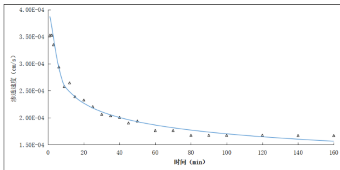
图 5.2-10 S2 渗水试验成果图
