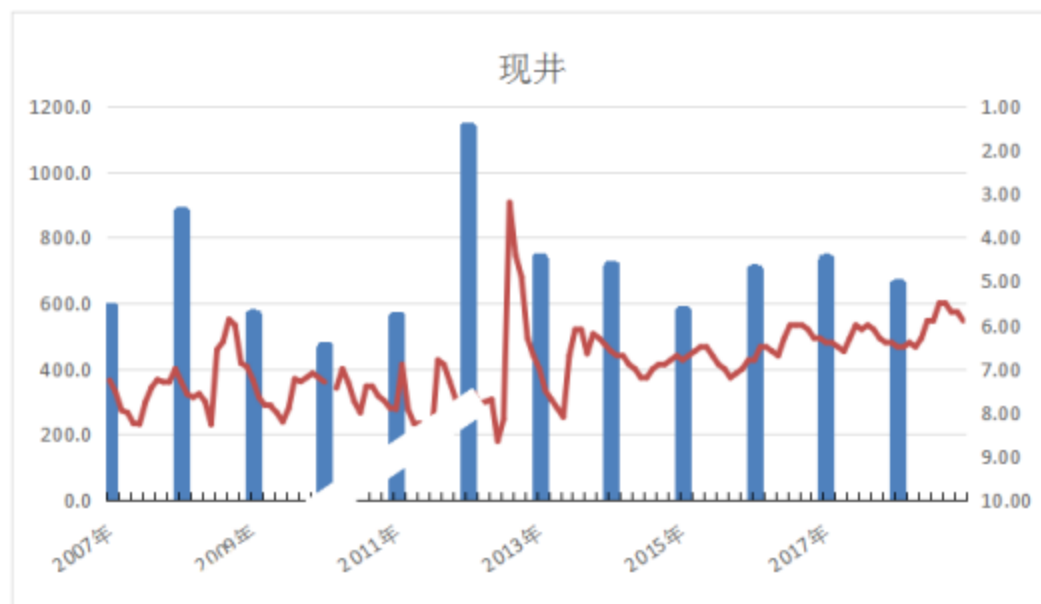
图 4.1-6 现井村地下水动态曲线
