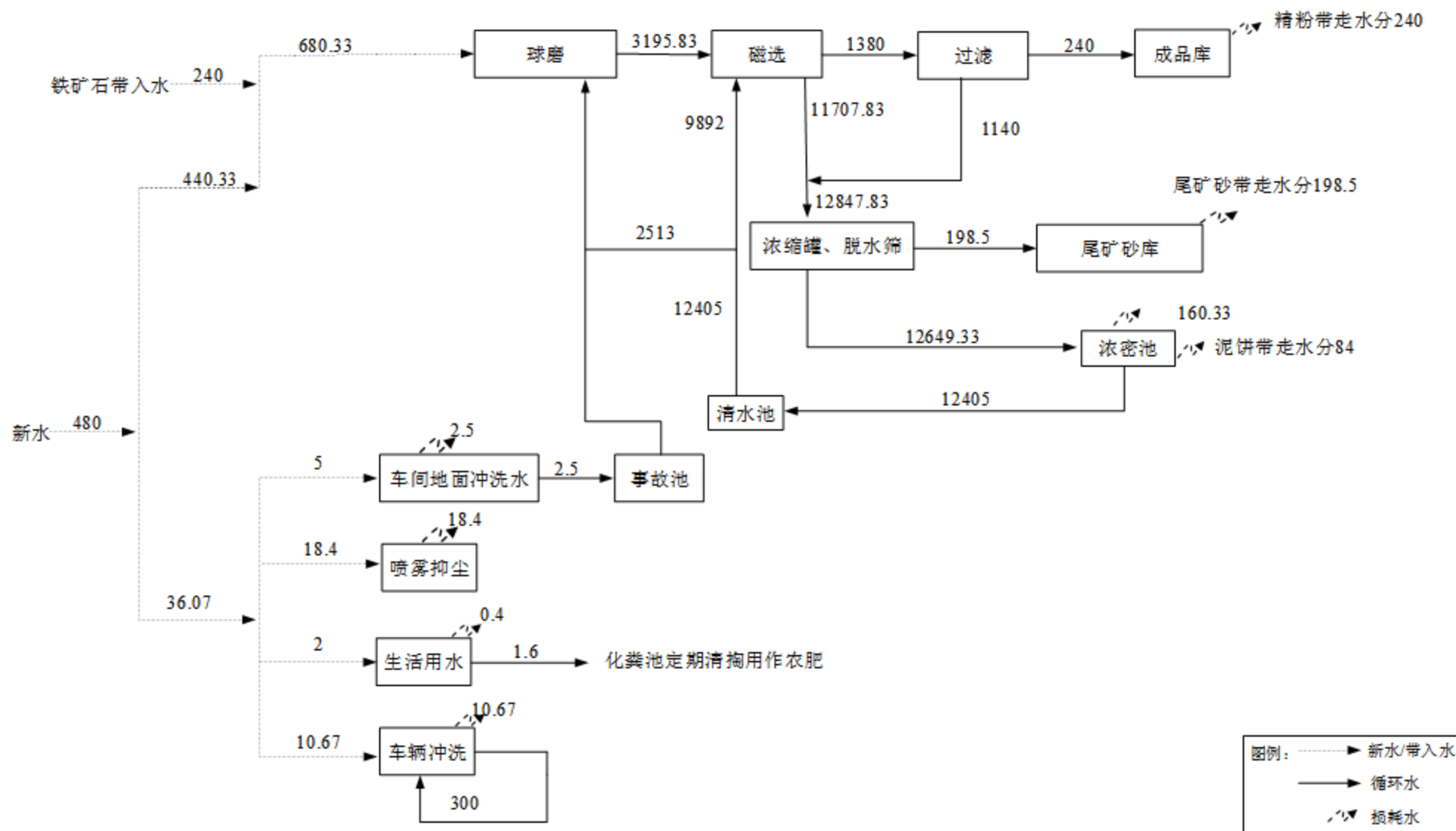
图 3.3-1 项目给排水平衡图 单位: \text{m}^3/\text{d}
