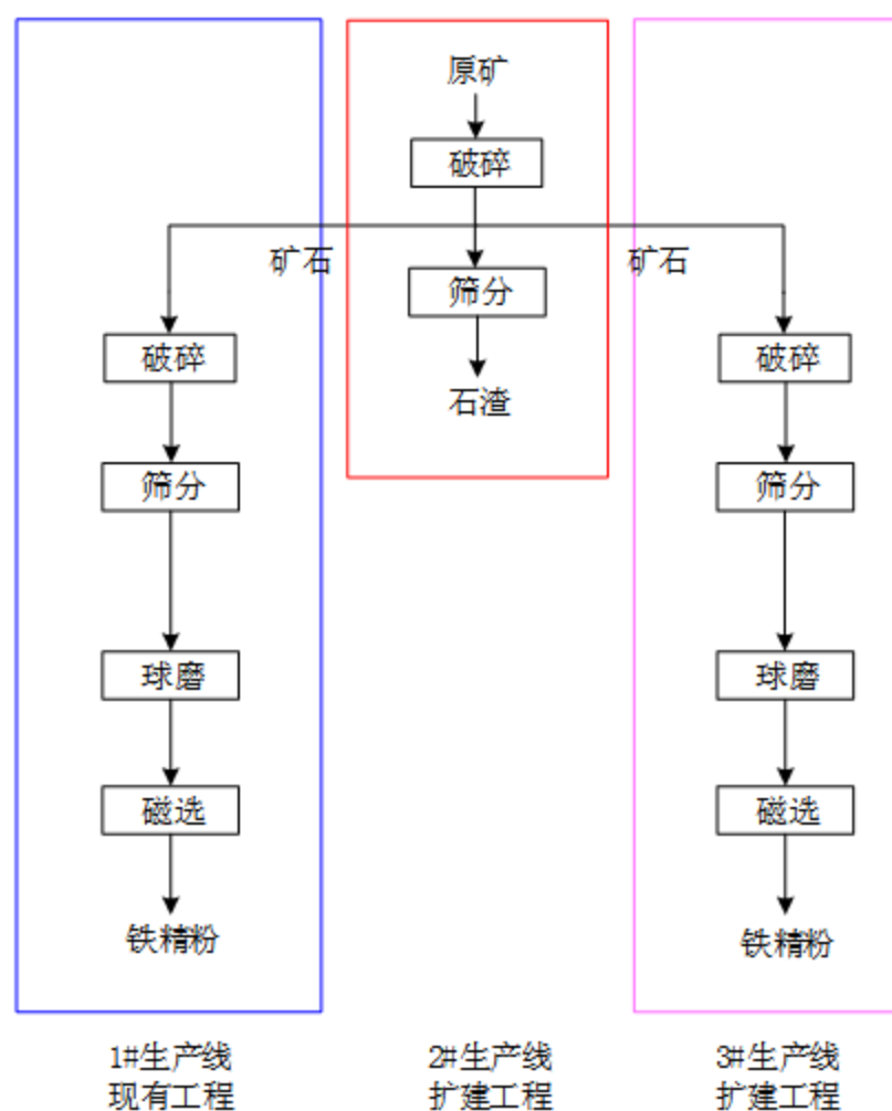
图 3.2-1 项目建成后全厂生产方案
