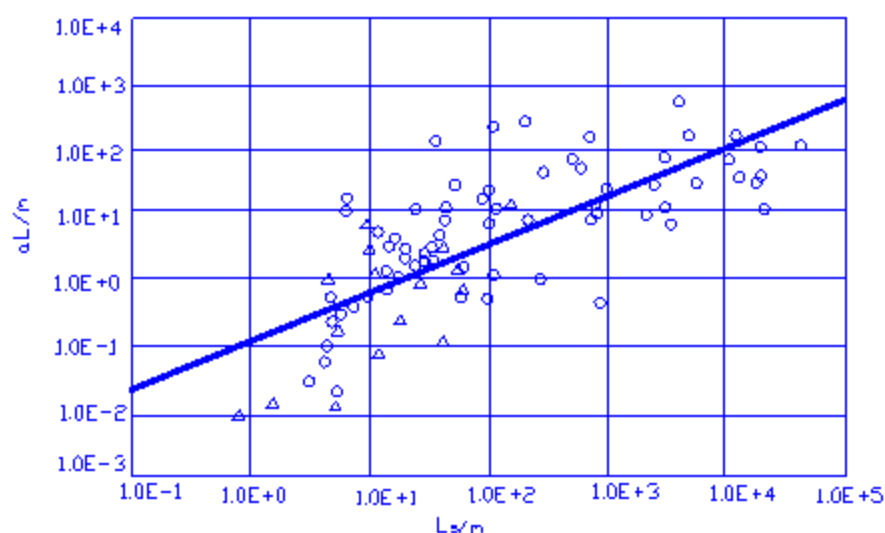
图 5.2-16 孔隙介质 2 维数值模型的 lg a_L - lg L 图
