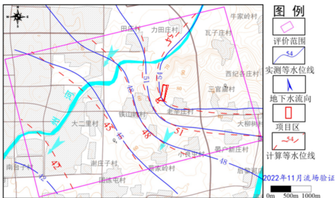
图 5.2-13 2022 年 11 月潜水等水位线识别图
