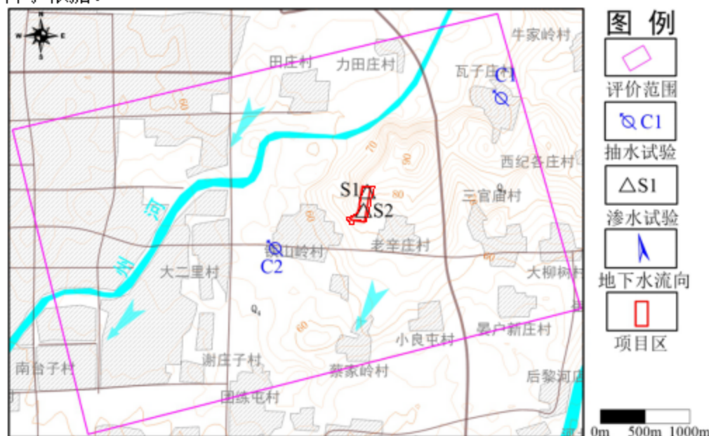
图 5.2-8 项目区抽水试验和渗水试验位置图
