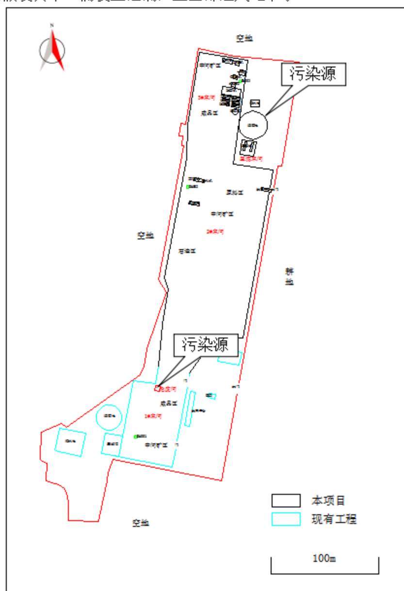
图 5.2-17 地下水污染源设定位置图
