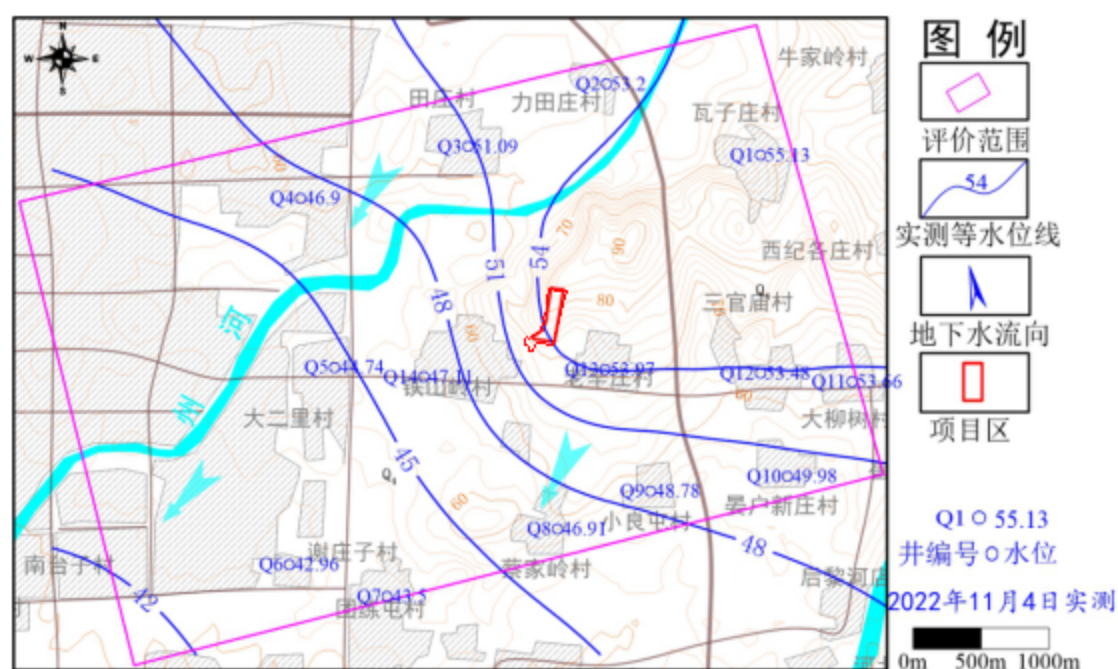
图 5.2-6 2022 年 11 月 4 日实测地下水流场
