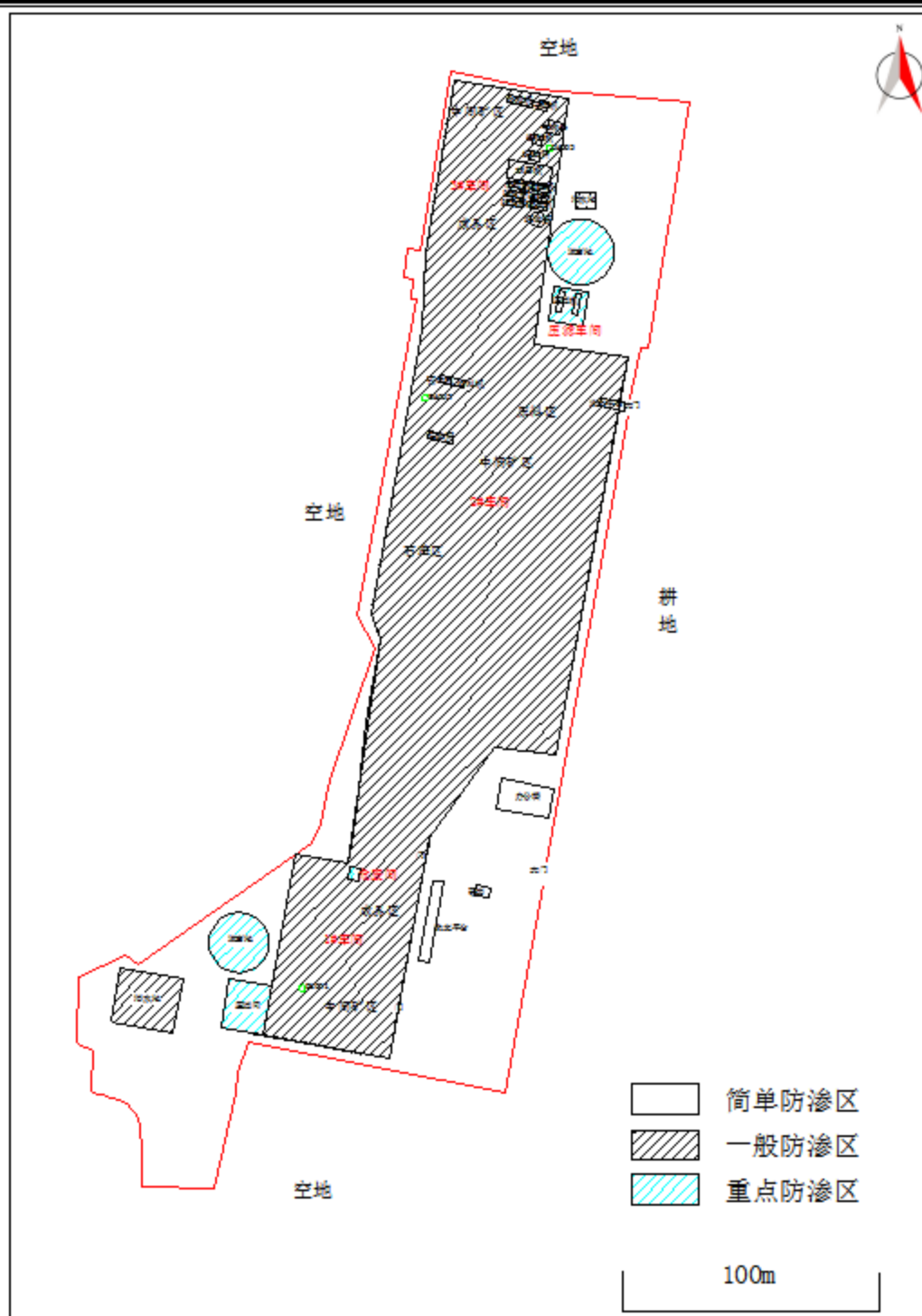
图 5.2-21 厂区防渗分区图
