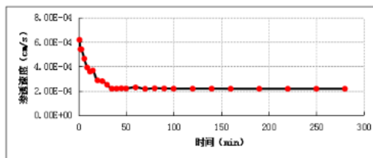
图 5.2-13 S-2 渗水试验成果图
