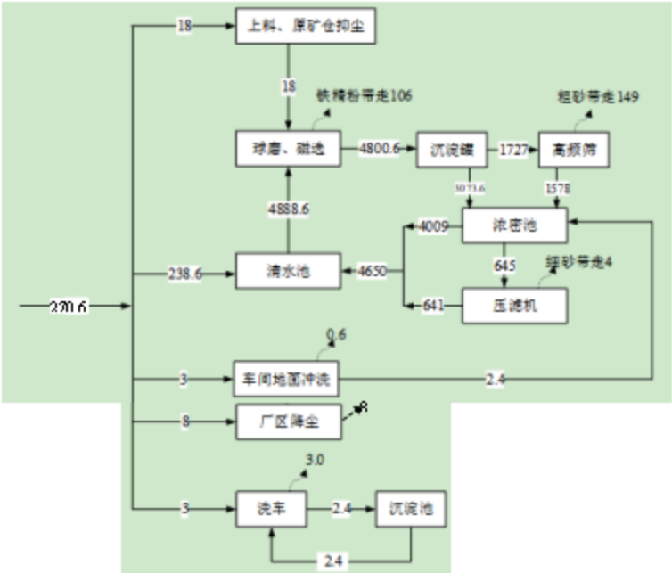
图 3.2-1 水平衡图 (单位: m³/d)
