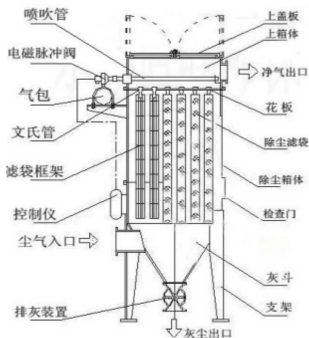
图 6.2-1 脉冲布袋式除尘器工作原理
