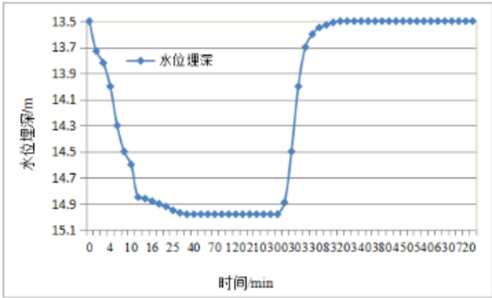
图 5.2-8 义井铺村抽水试验水位降深-时间曲线
