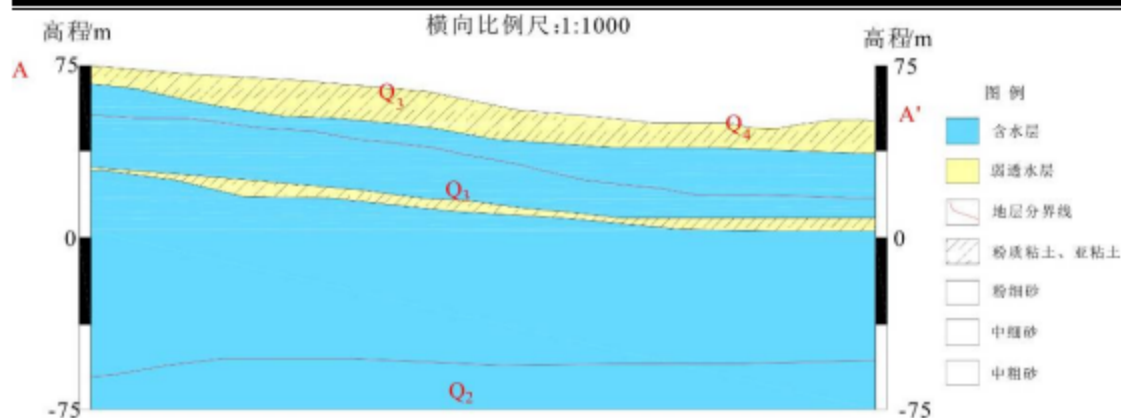
图 5.2-2 A-A'剖面图
