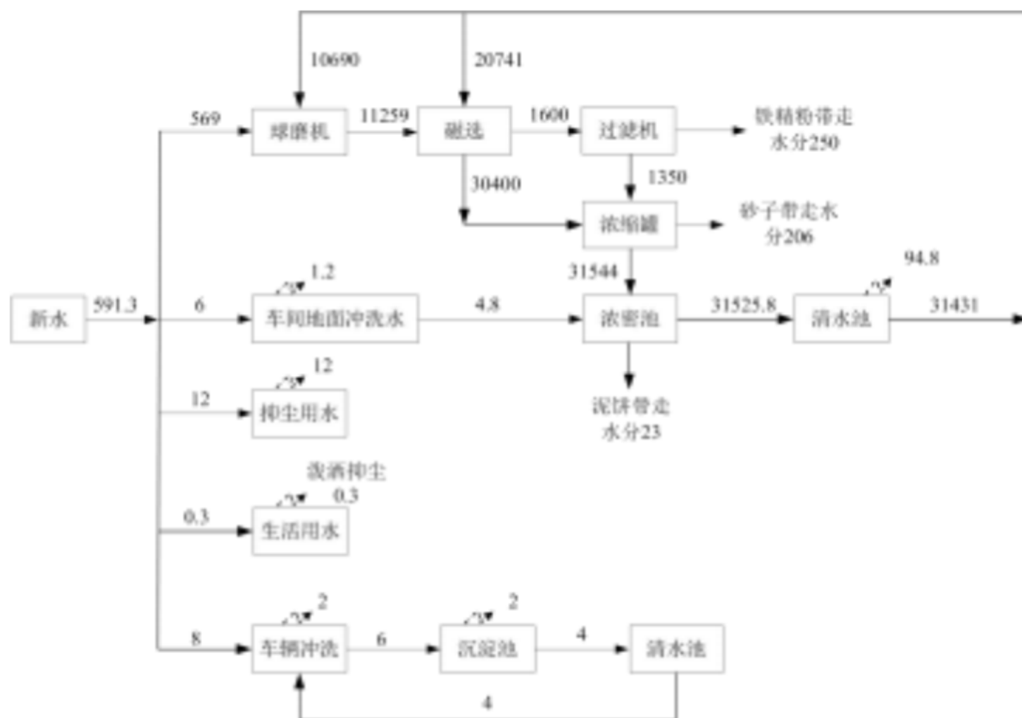
图 3.2-1 项目给排水平衡图 单位: \text{m}^3/\text{d}
