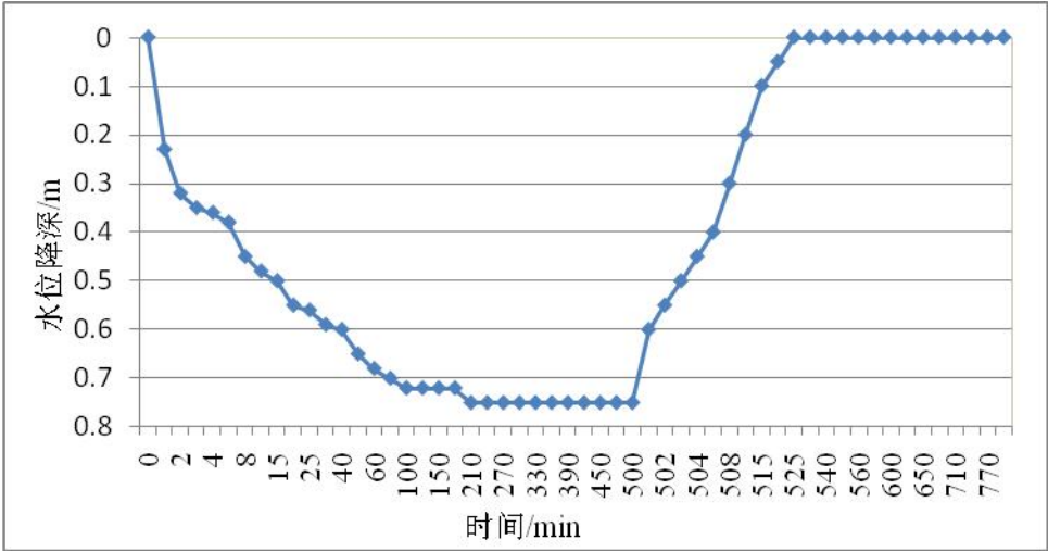
图5.2-7 东桃园村东抽水试验水位降深-时间曲线
