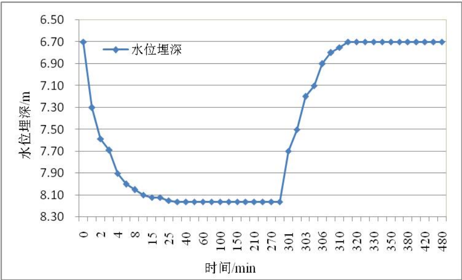
图5.2-10 上石河村抽水试验水位埋深-时间曲线
