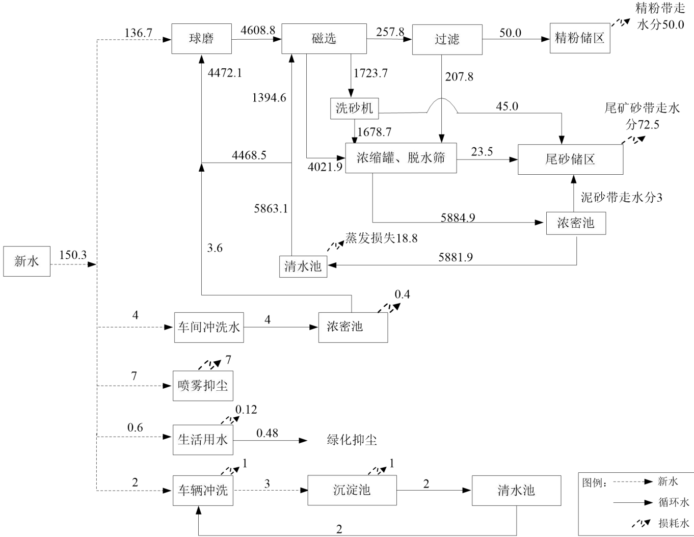
图 3.2-1 项目给排水平衡图 单位: m³/d
