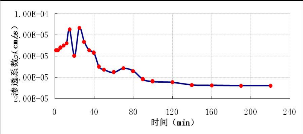
图 5.2-12 S-1 渗水试验成果图
