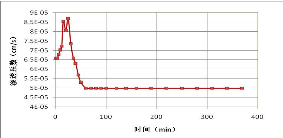
图 5.2-14 S-3 渗水试验成果图
