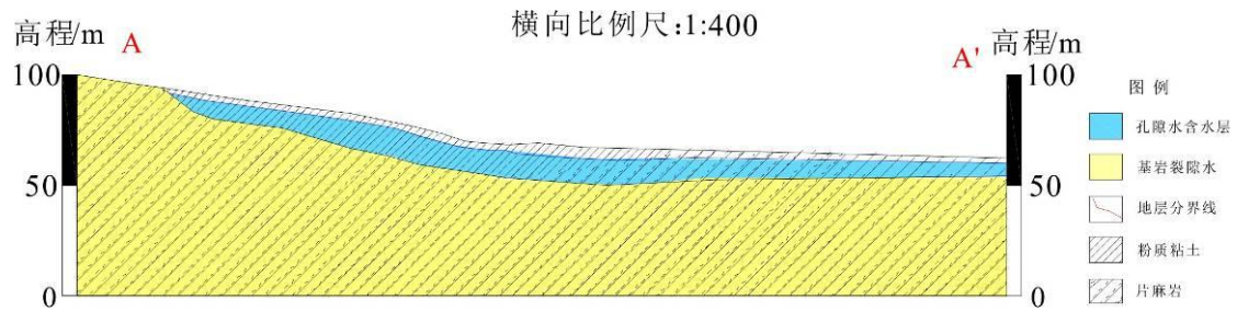
图 5.2-2 评价区地质图及剖面图
