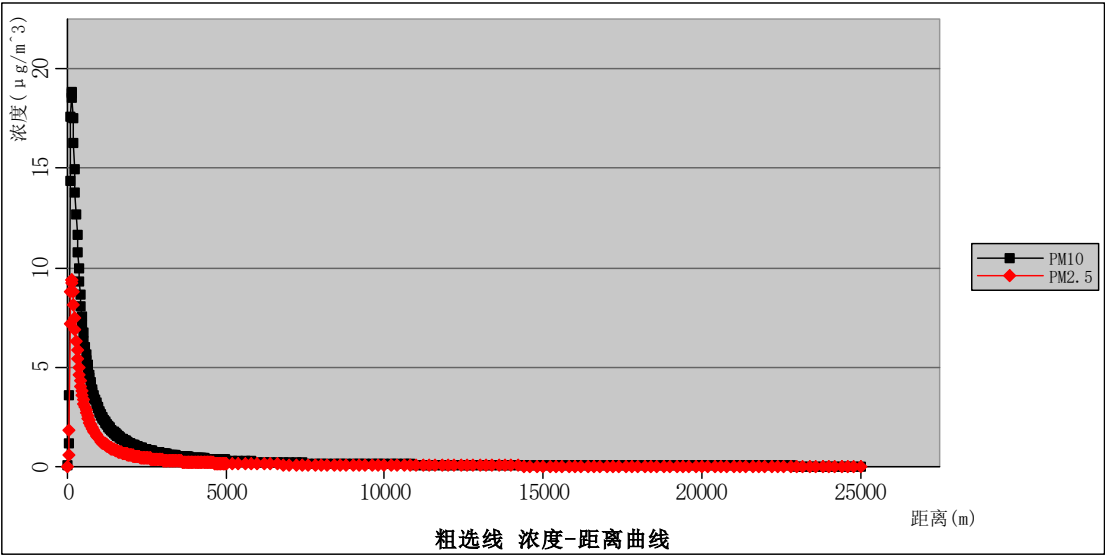
图 5.2-1 粗选线有组织废气浓度距离曲线图 \mu\text{g}/\text{m}^3
