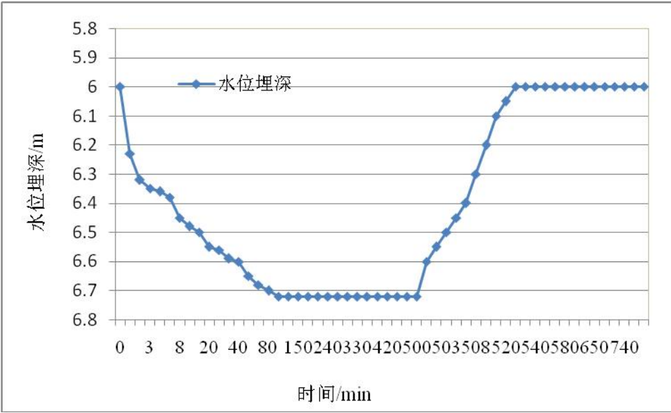
图5.2-8 东桃园村东抽水试验水位埋深-时间曲线
