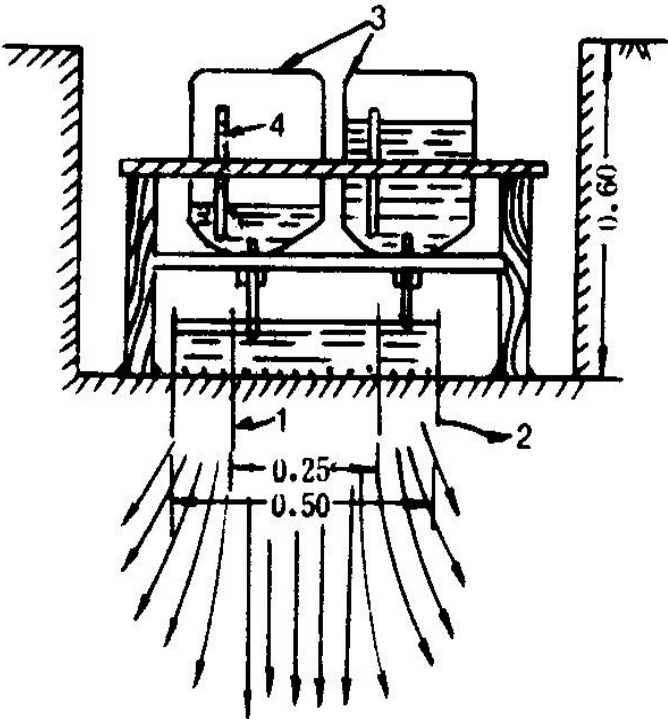
图5.2-11 双环渗水试验原理图
