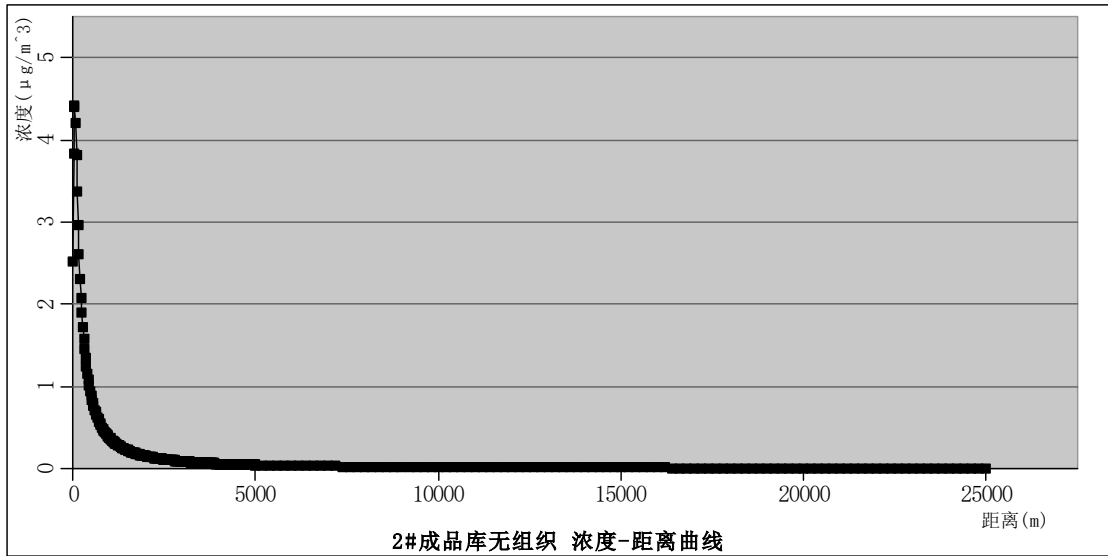
图 5.2-3 2#成品库无组织废气浓度距离曲线图 \mu\text{g}/\text{m}^3
