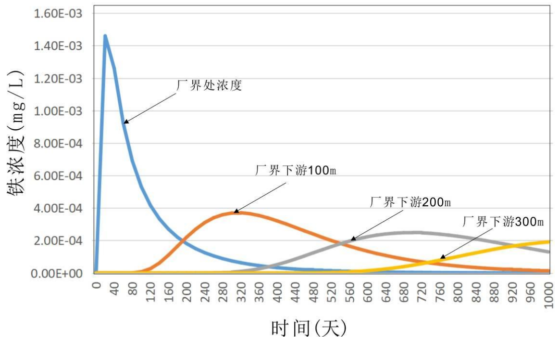
图 5.2-15 厂界、距厂界 100 米、200 米、300 米处铁浓度随时间变化过程线
