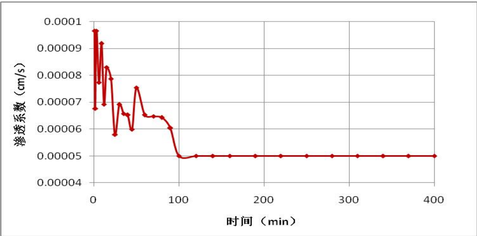
图 5.2-13 S-2 渗水试验成果图
