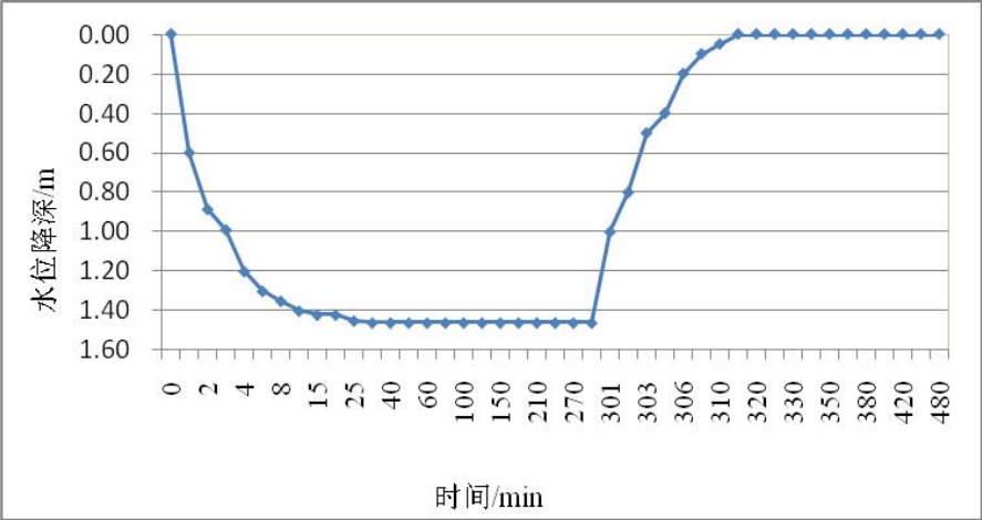
图5.2-9 上石河村抽水试验水位降深-时间曲线
