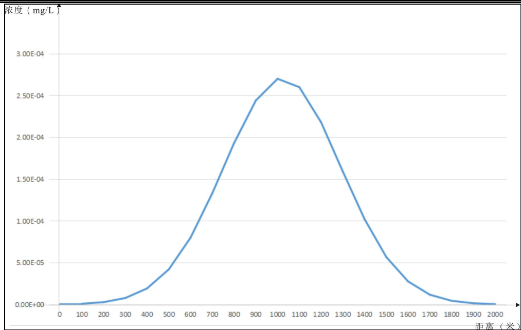
图 5.2-23 泄漏 3650d 后厂区下游铁浓度时间变化
