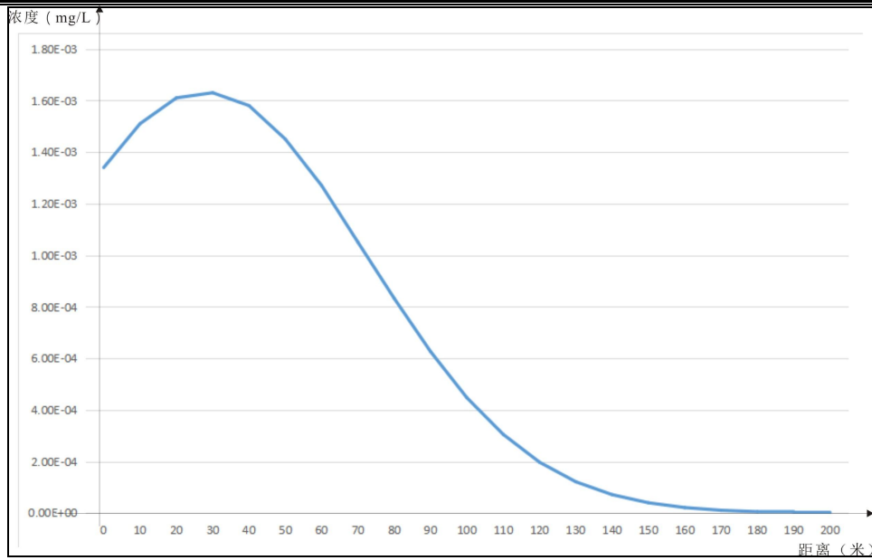
图 5.2-21 泄漏 100d 后厂区下游铁浓度时间变化
