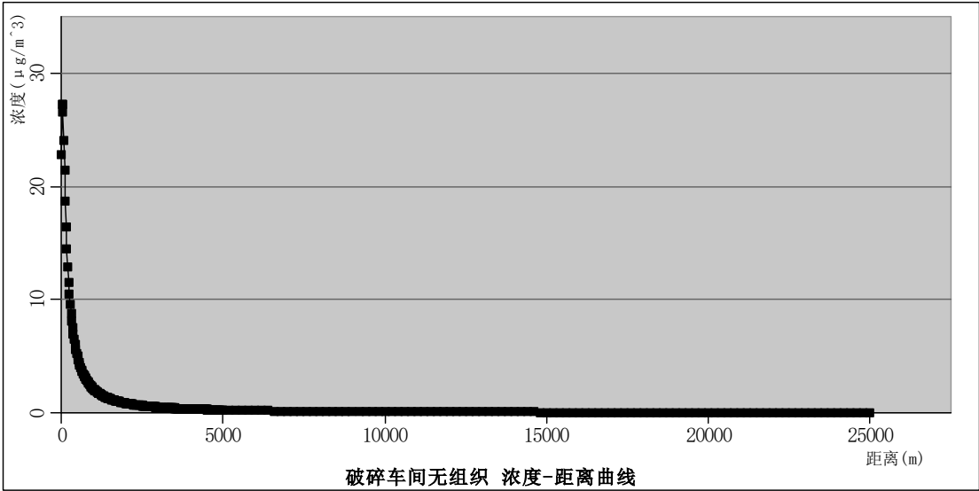
图 5.2-5 破碎车间无组织废气浓度距离曲线图 \mu\text{g}/\text{m}^3
