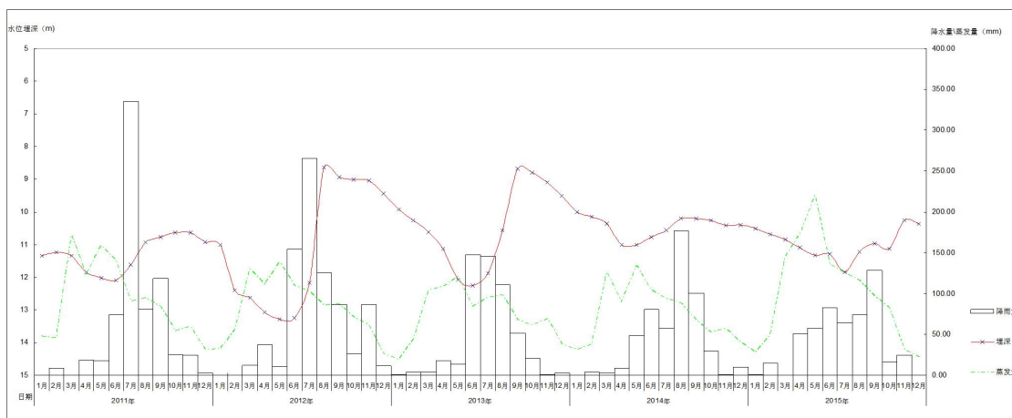
图 5.2-8 第四系浅层地下水水位 5 年变化与降水关系曲线
