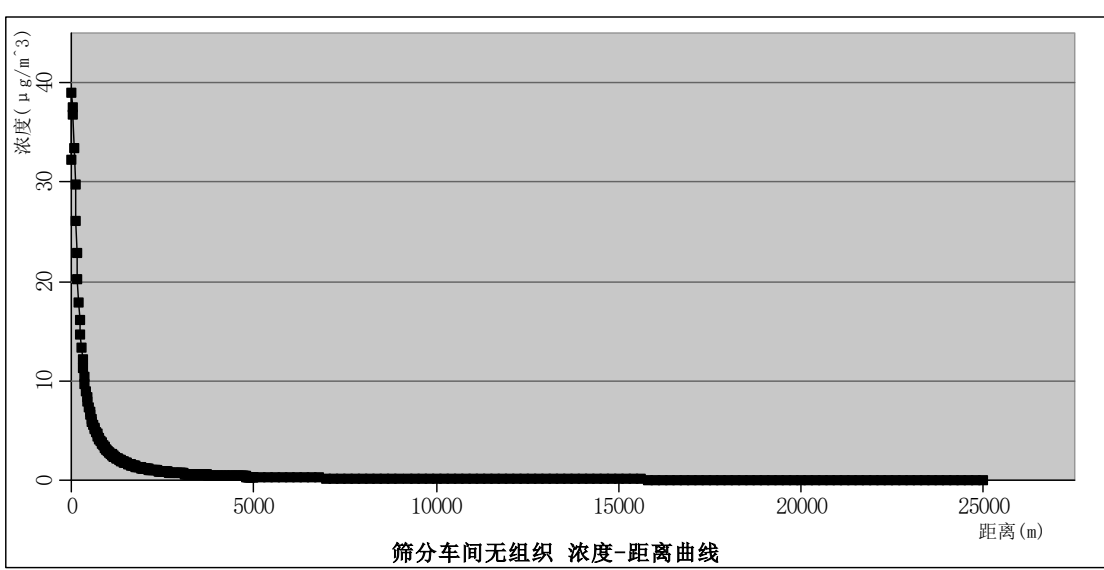
图 5.2-6 筛分车间无组织废气浓度距离曲线图 \mu\text{g}/\text{m}^3
