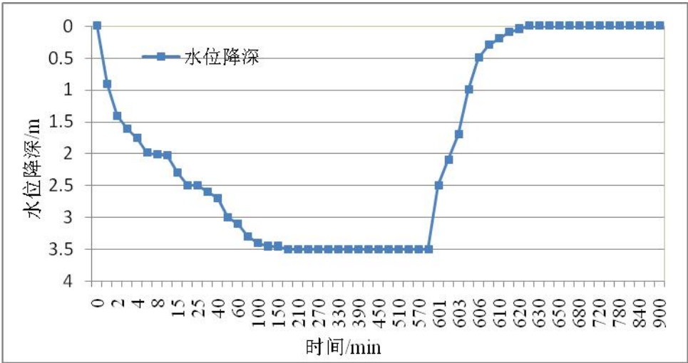
图5.2-7 般若院村抽水试验降深-时间曲线
