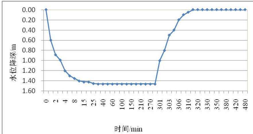
图5.2-11 上石河村抽水试验水位降深-时间曲线
