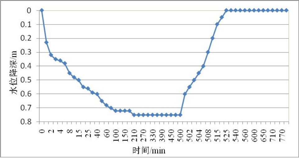
图5.2-9 东桃园村东抽水试验水位降深-时间曲线
