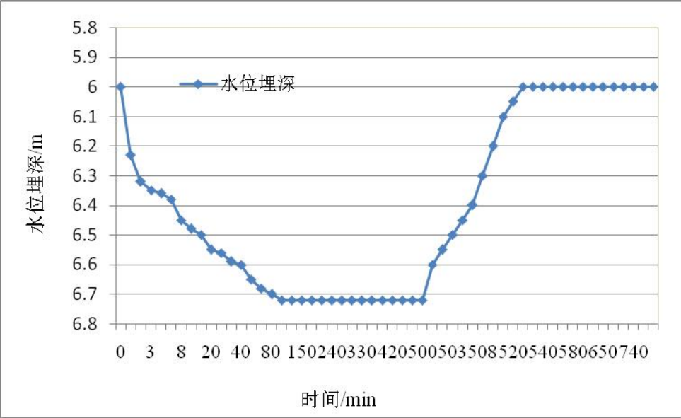
图5.2-10 东桃园村东抽水试验水位埋深-时间曲线
