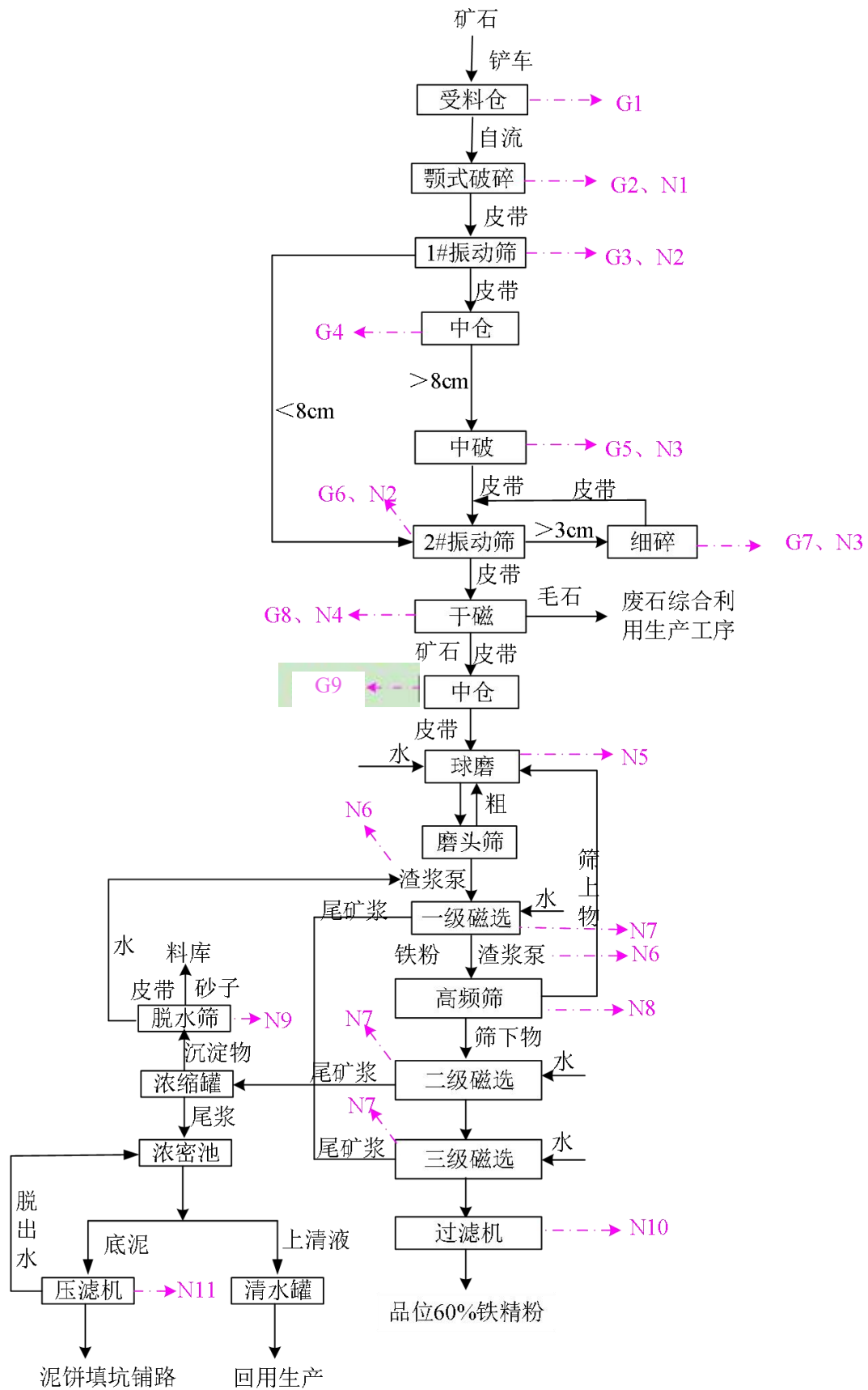
图 3.4-1 项目生产工艺流程及排污节点图
