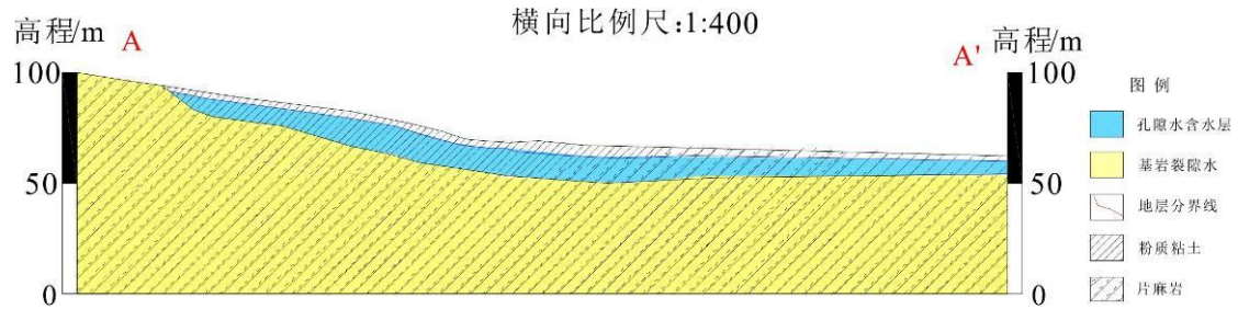
图 5.2-2 评价区地质图及剖面图
