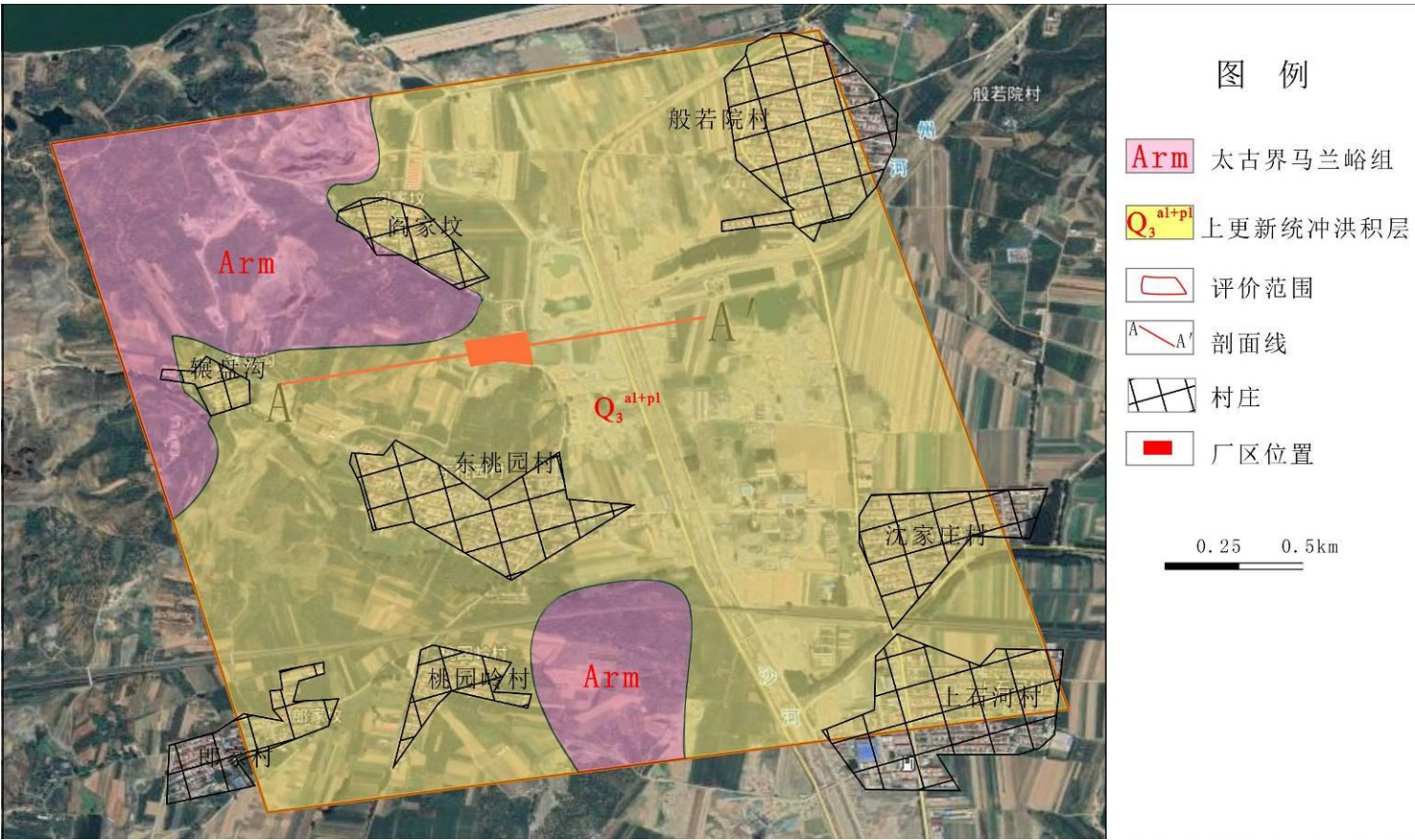
图 5.2-1 评价区地质图
