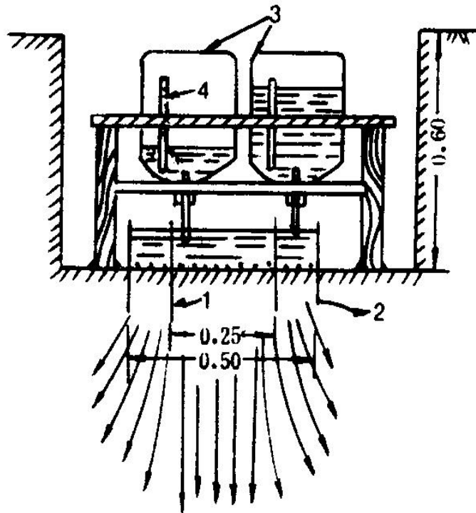
图5.2-13 双环渗水试验原理图
