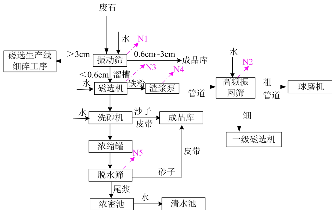
图 3.4-2 废石综合利用生产工艺流程及排污节点图
