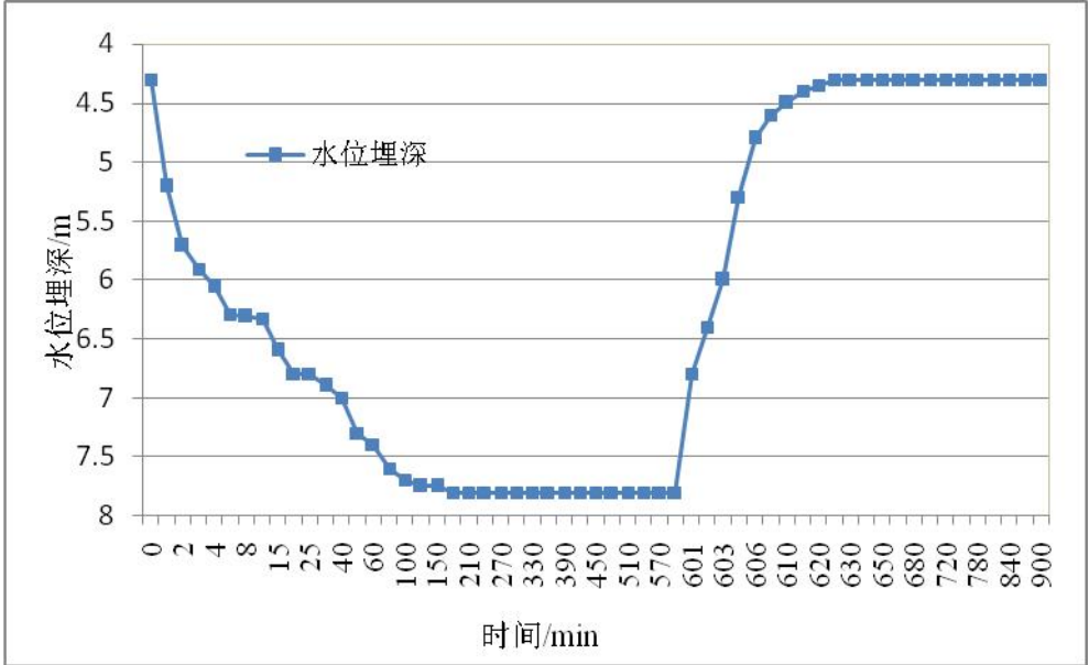
图5.2-8 般若院村抽水试验水位埋深-时间曲线
