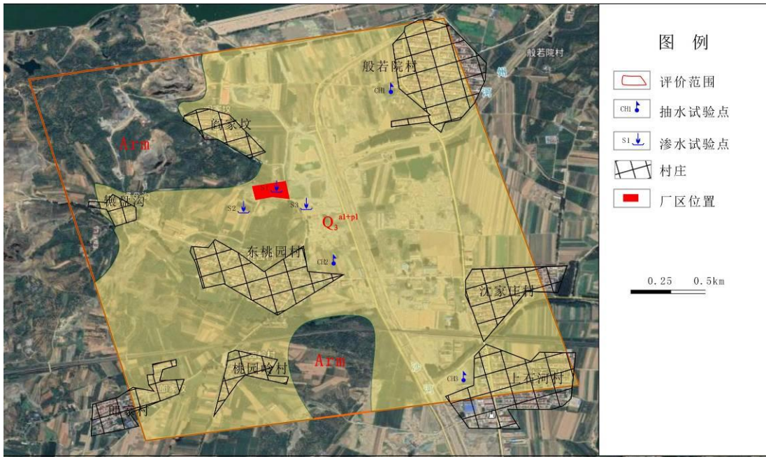
图 5.2-6 项目区抽水试验和渗水试验位置图
