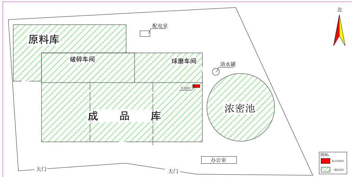
图5.2-19 厂区防渗分区图
