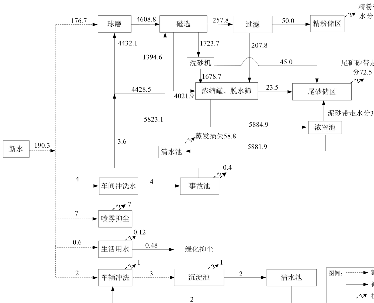
图 3.2-1 项目给排水平衡图 单位: m³/d
