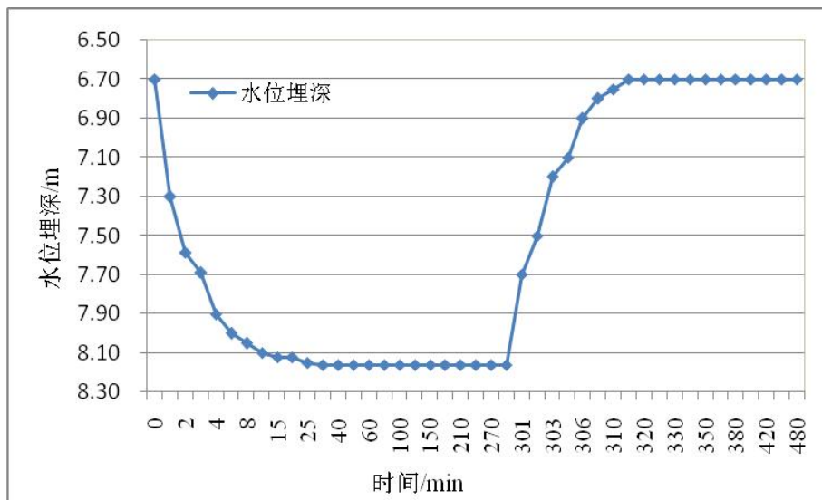
图5.2-12 上石河村抽水试验水位埋深-时间曲线
