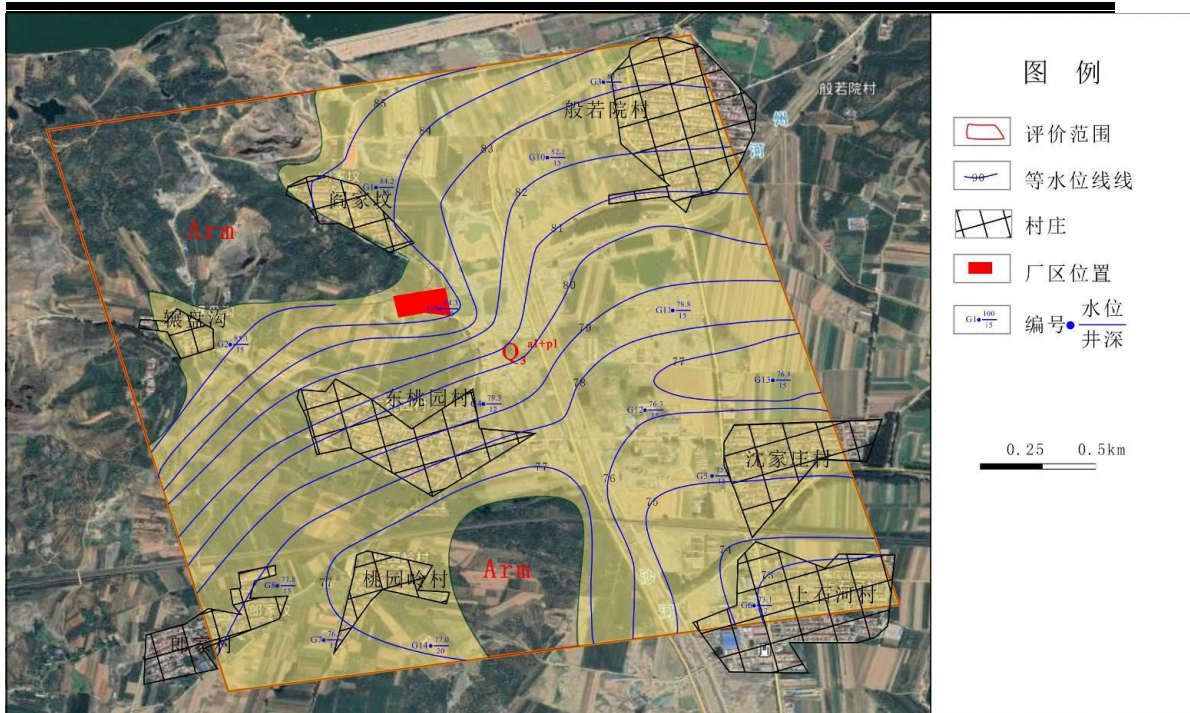
图 5.2-5 浅层地下水流场
