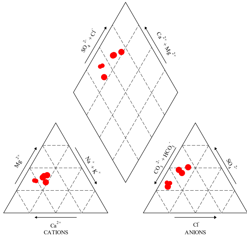
图 5.2-4 评价区水化学类型 piper 图
