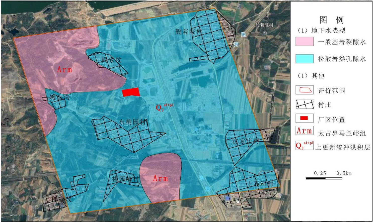
图 5.2-3 评价区水文地质图
