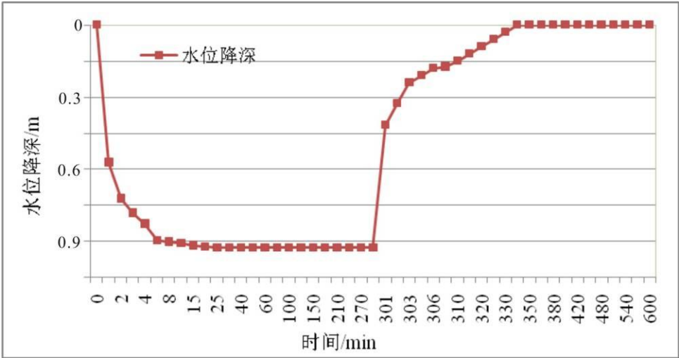
图5.2-7 项目厂区抽水试验降深-时间曲线
