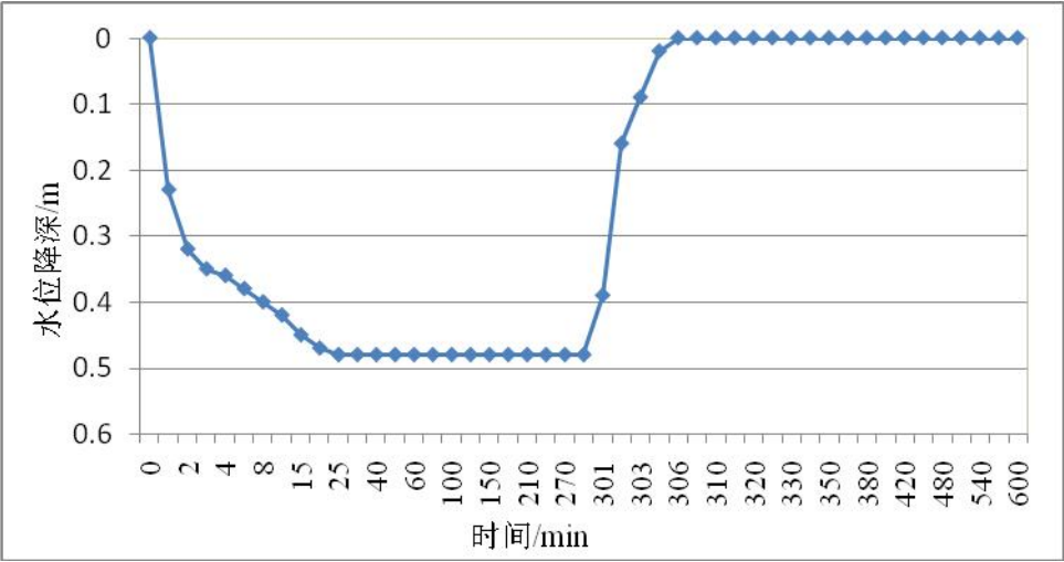
图5.2-9 北头山村抽水试验水位埋深-时间曲线
