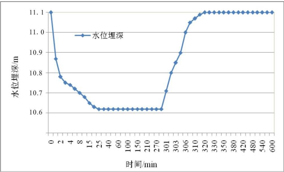
图5.2-10北头山村抽水试验水位降深-时间曲线
