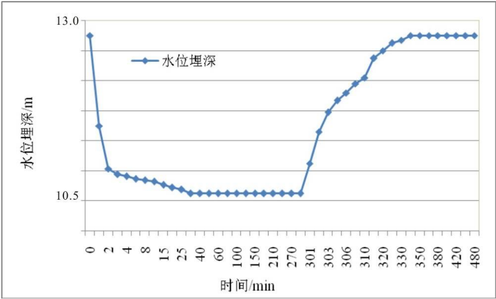
图5.2-11 力田庄村内抽水试验水位埋深-时间曲线
