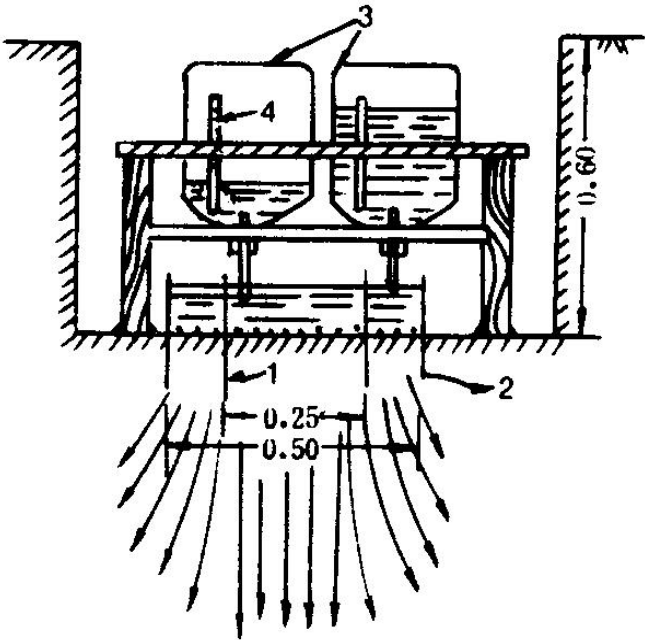
图5.2-13 双环渗水试验原理图
