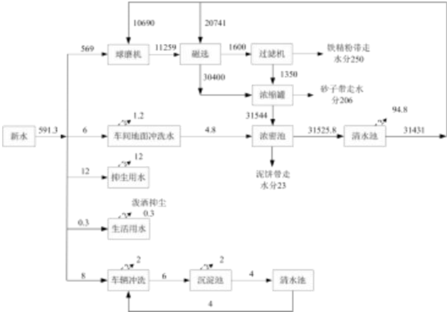
图 3.2-1 项目给排水平衡图 单位：m³/d
