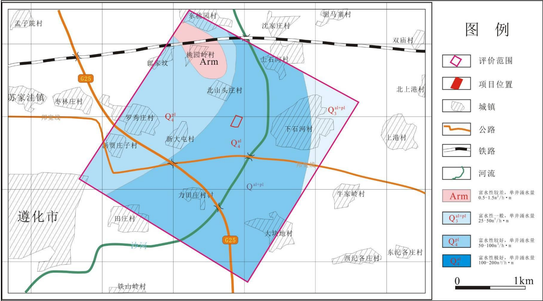
图 5.2-3 评价区水水文地质图
