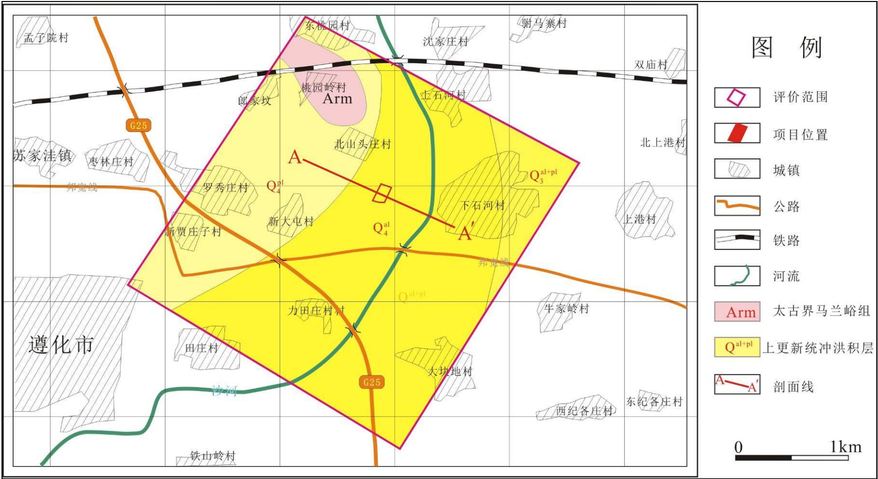
图 5.2-1 评价区地质图
