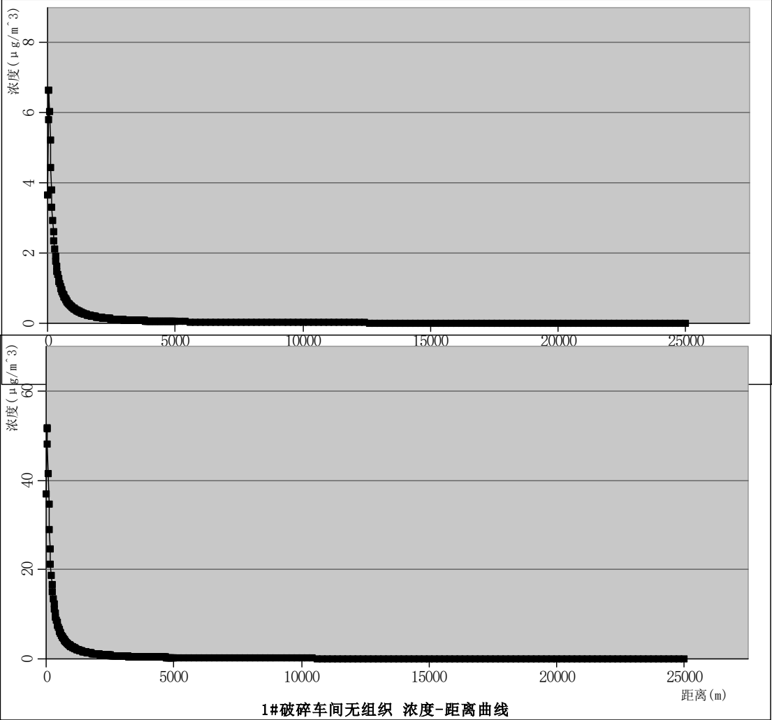
图 5.2-2 南厂区破碎线排气筒废气浓度距离曲线图 \mu\text{g}/\text{m}^3
