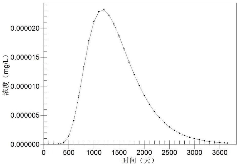
图 5.2-18 距离污染泄漏点 200 米处铁浓度时间变化过程线
