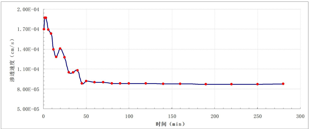
图 5.2-15 S-2 渗水试验成果图
