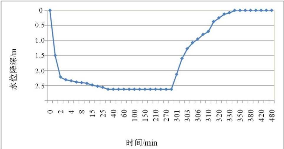
图5.2-12 力田庄村内抽水试验水位降深-时间曲线
