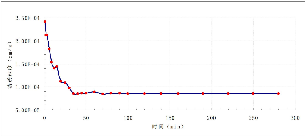
图 5.2-16 S-3 渗水试验成果图
