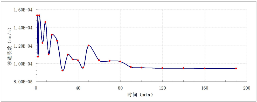
图 5.2-14 S-1 渗水试验成果图
