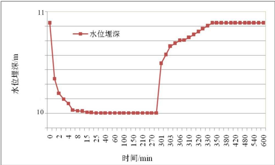
图5.2-8 项目厂区抽水试验水位埋深-时间曲线
