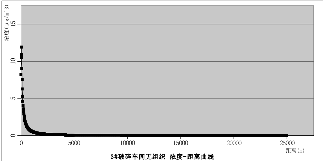
图 5.2-7 3#破碎车间无组织废气浓度距离曲线图 \mu\text{g}/\text{m}^3
