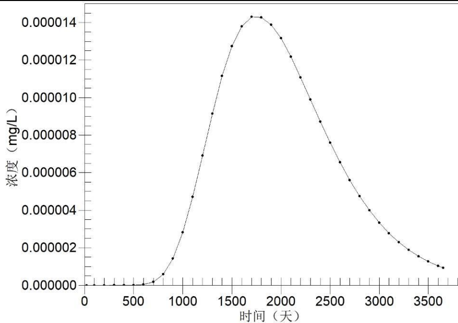
图 5.2-19 距离污染泄漏点 300 米处铁浓度时间变化过程线
