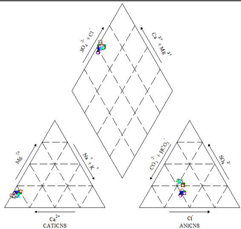
图 4.1-8 研究区水化学类型 piper 图
