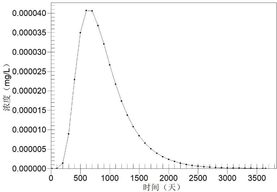
图 5.2-17 距离污染泄漏点 100 米处铁浓度时间变化过程线
