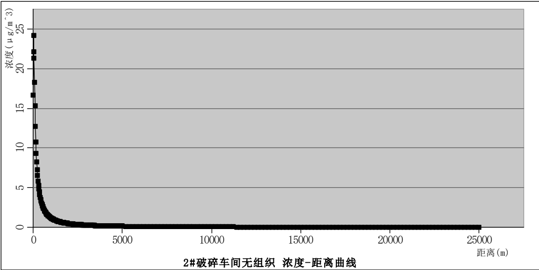
图 5.2-6 2#破碎车间无组织废气浓度距离曲线图 \mu\text{g}/\text{m}^3
