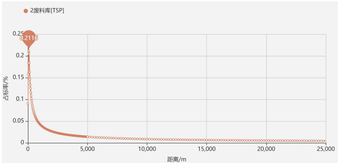
图 5.2-4 2#废料库（现有，尾矿砂、泥饼）无组织废气占标率距离曲线图
