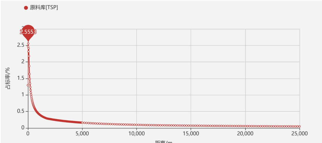
图 5.2-1 入料棚（本项目新增）无组织废气占标率距离曲线图
