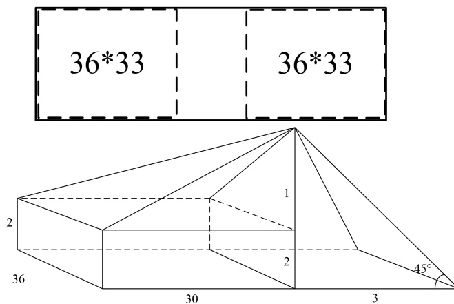
图 3.2-3 成品库堆存示意图
