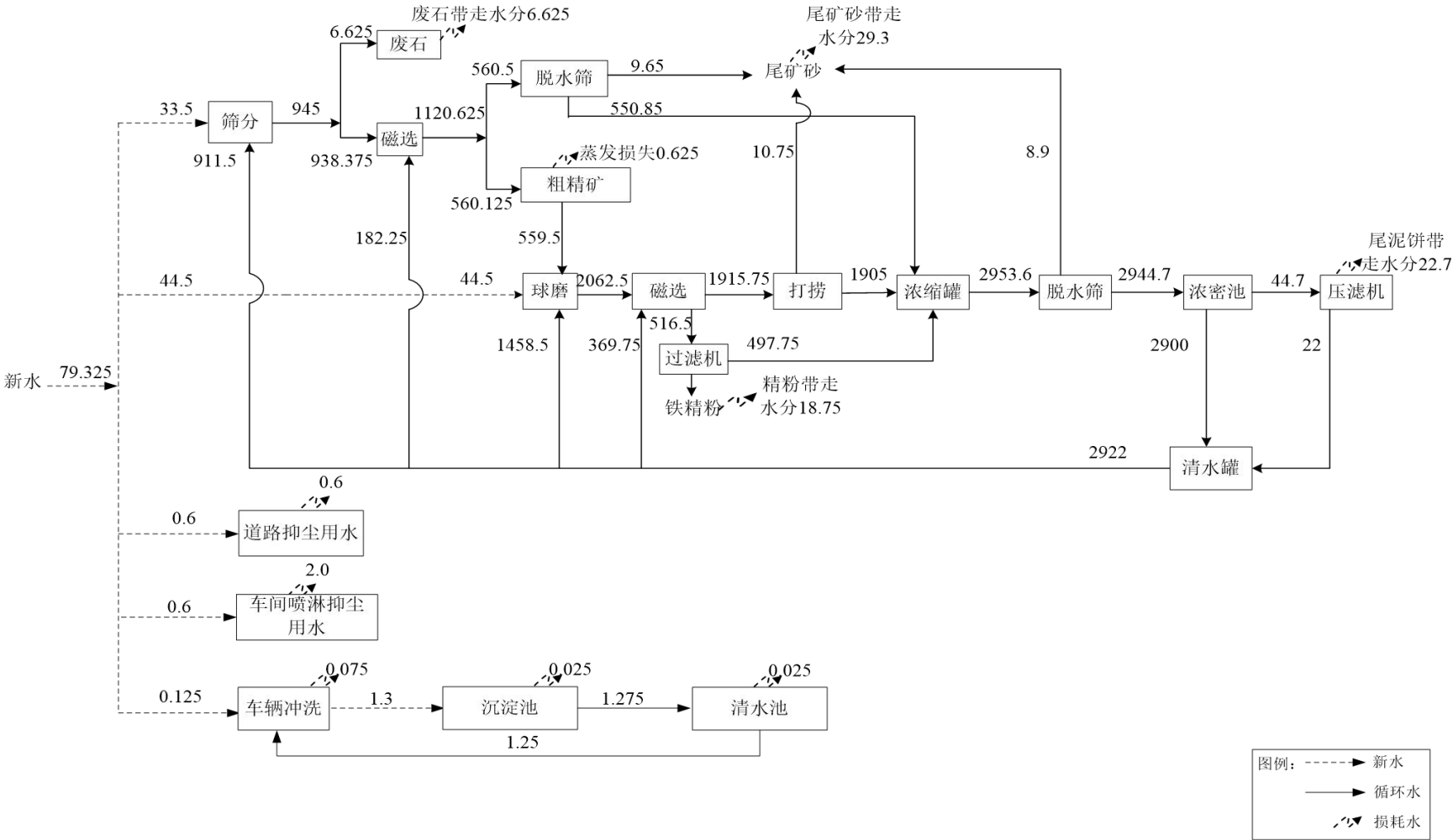
图 3.2-4 本项目新增用排水
