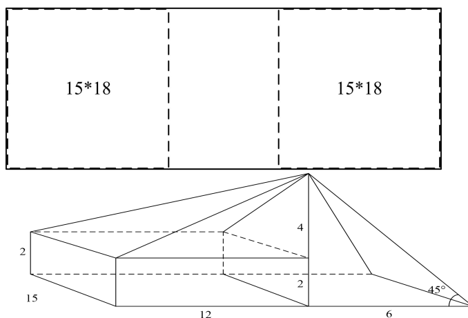
图 3.2-2 入料棚堆存示意图
