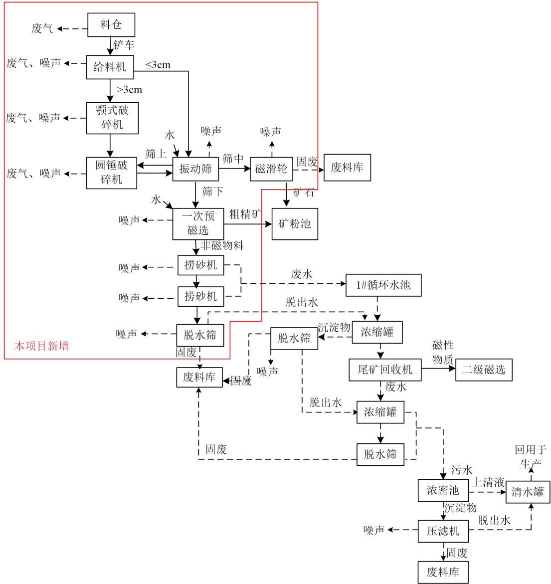
图3.3-1 粗破生产线生产工艺及生产排污节点图
