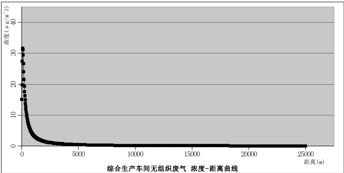
图 5.2-2 综合生产车间无组织废气浓度距离曲线图 \mu\text{g}/\text{m}^3
