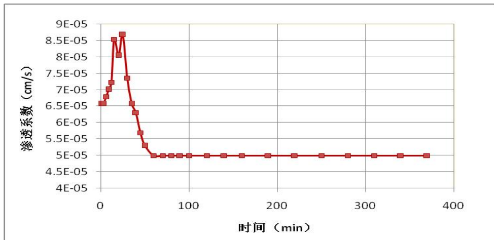
图 5.2-11 S-3 渗水试验成果图
