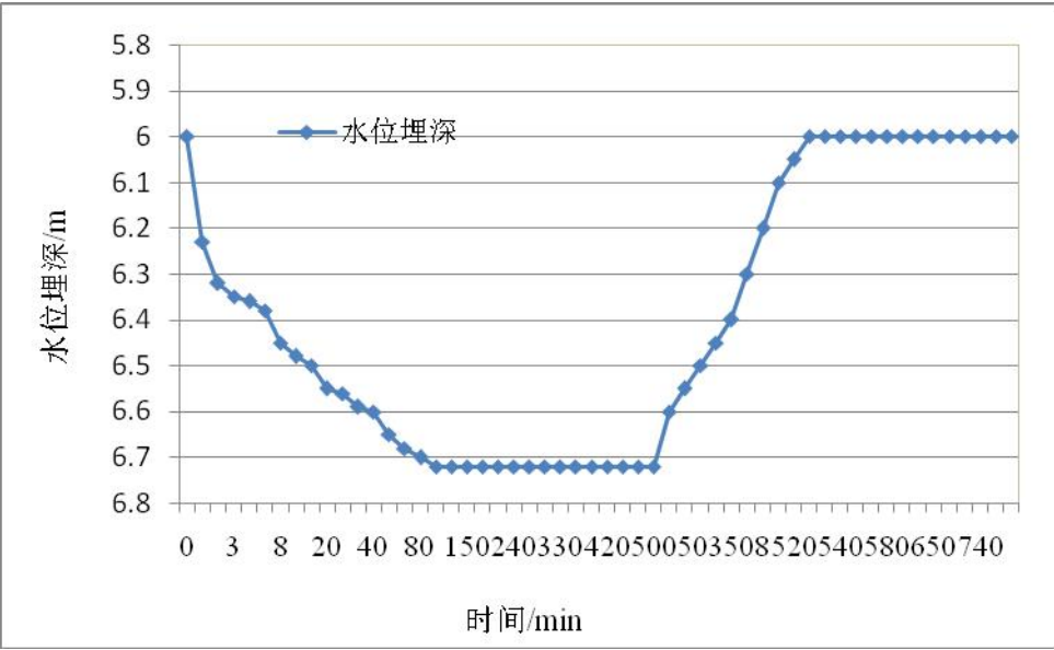
图5.2-5 东桃园村东抽水试验水位埋深-时间曲线
