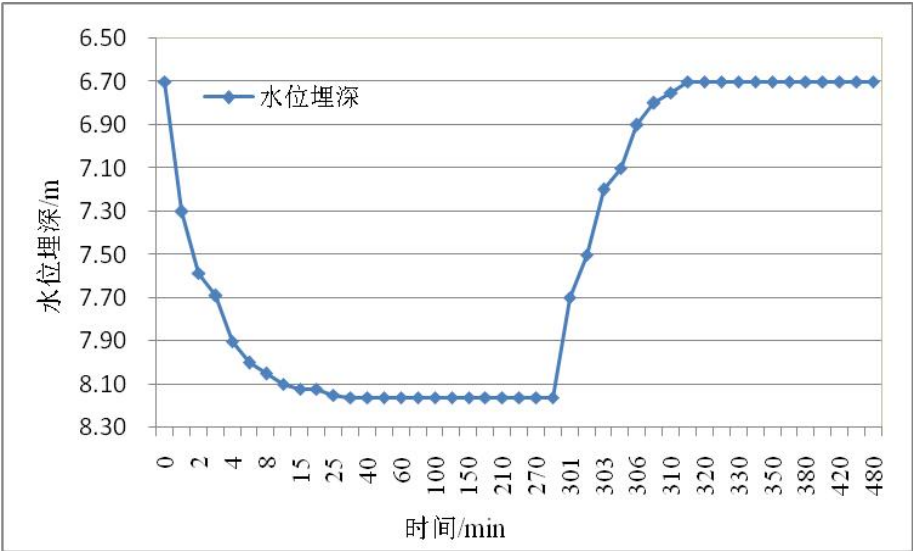
图5.2-7 上石河村抽水试验水位埋深-时间曲线
