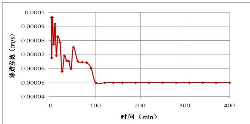
图 5.2-10 S-2 渗水试验成果图
