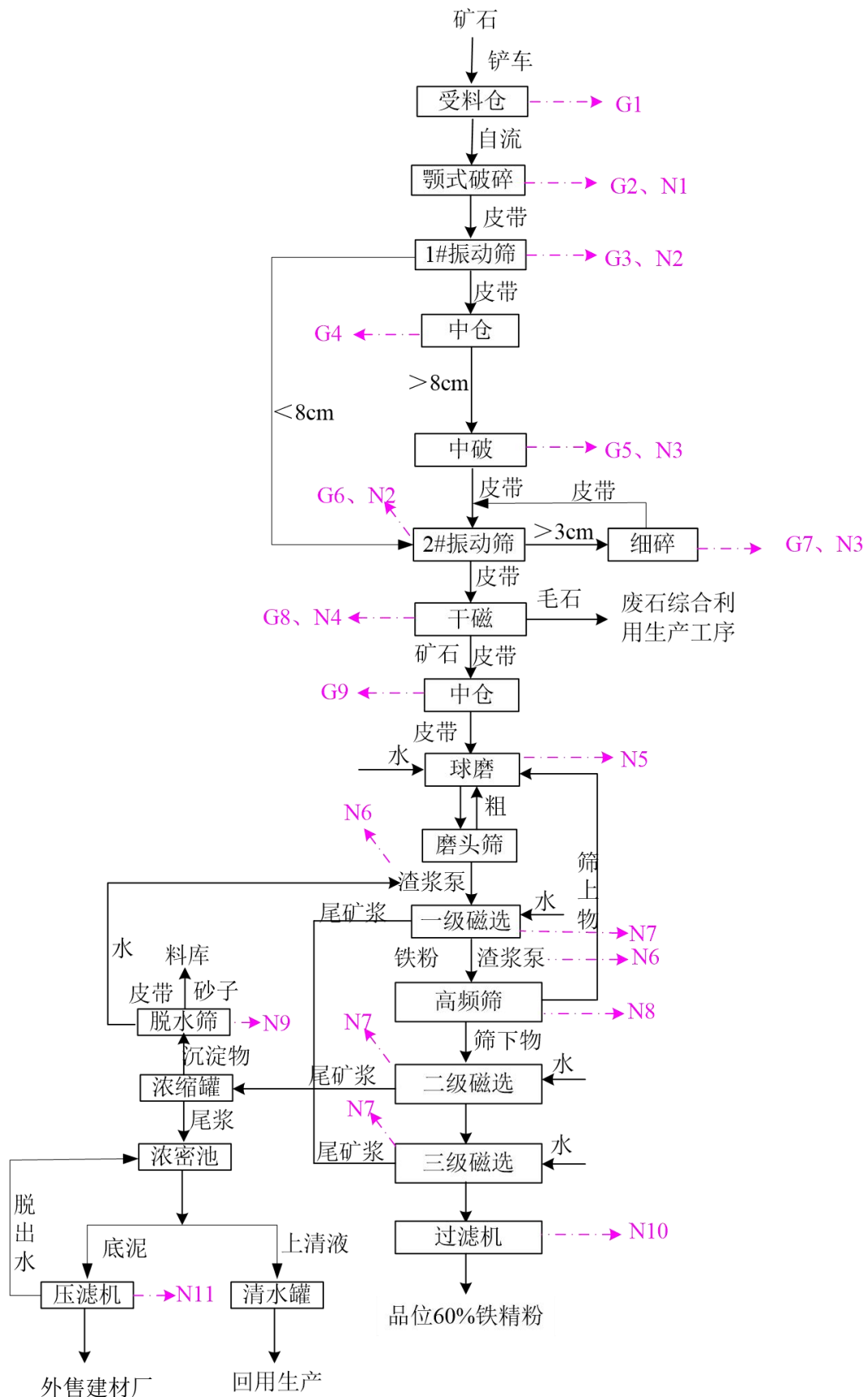
图 3.4-2 项目生产工艺流程及排污节点图
