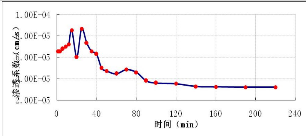
图 5.2-9 S-1 渗水试验成果图
