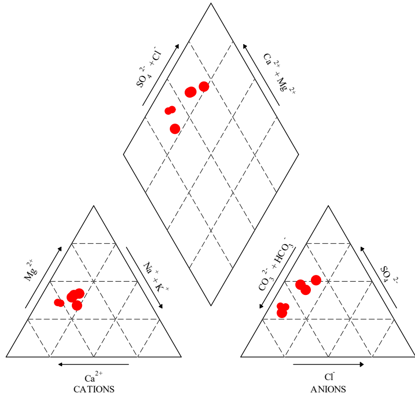
图 5.2-1 评价区水化学类型 piper 图
