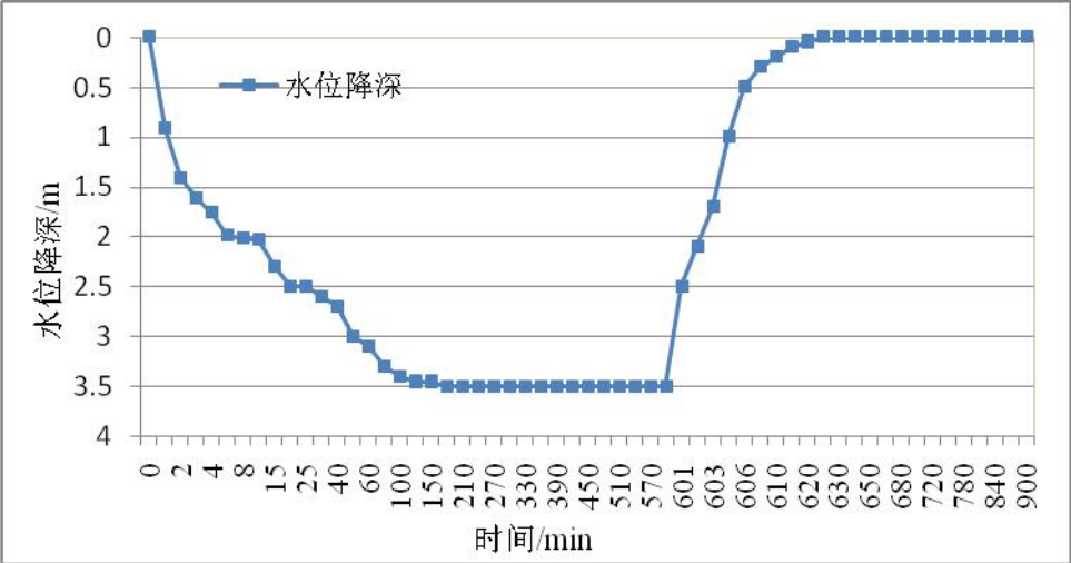
图5.2-2 般若院村抽水试验降深-时间曲线
