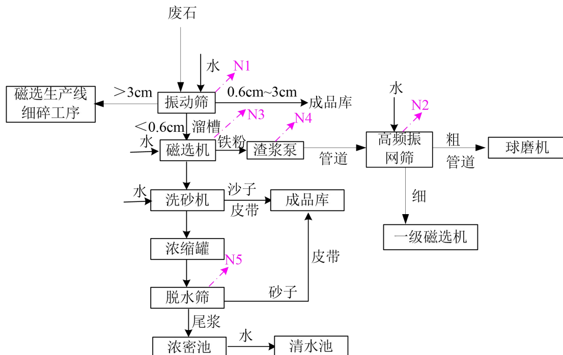
图 3.4-3 废石综合利用生产工艺流程及排污节点图
