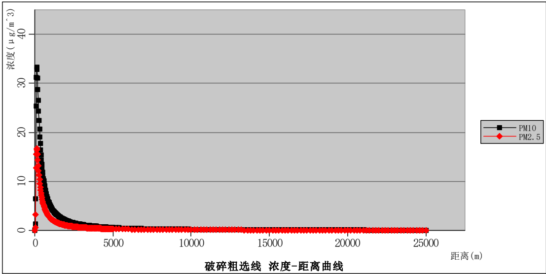
图 5.2-1 粗选生产线废气浓度距离曲线图 \mu\text{g}/\text{m}^3
