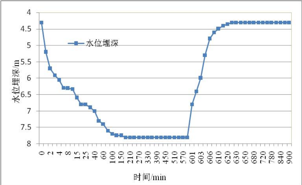
图5.2-3 般若院村抽水试验水位埋深-时间曲线
