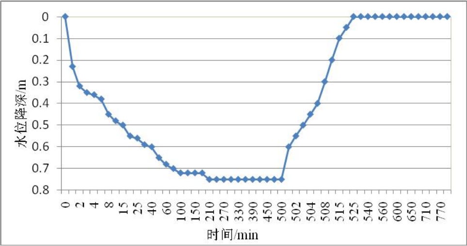
图5.2-4 东桃园村东抽水试验水位降深-时间曲线
