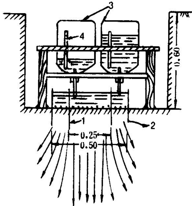
图5.2-8 双环渗水试验原理图
