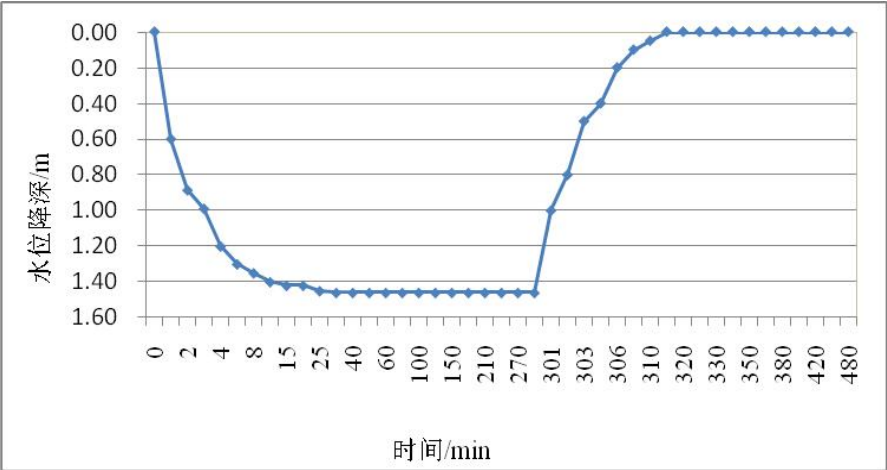
图5.2-6 上石河村抽水试验水位降深-时间曲线
