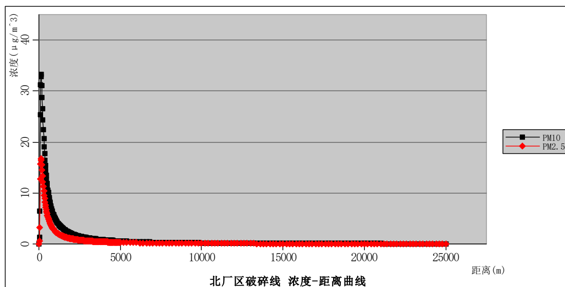
图 5.2-1 北厂区破碎线排气筒废气浓度距离曲线图 \mu\text{g}/\text{m}^3
