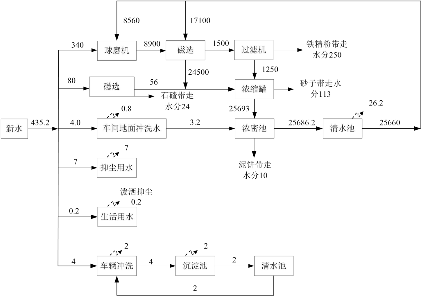
图 3.2-1 项目南厂区给排水平衡图 单位：m³/d
