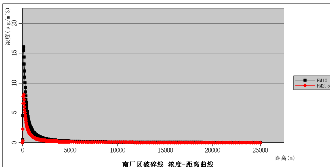
图 5.2-2 南厂区破碎线排气筒废气浓度距离曲线图 \mu\text{g}/\text{m}^3
