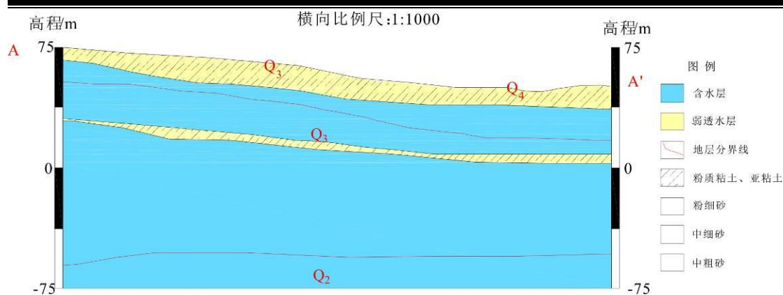
图 5.2-2 A-A'剖面图
