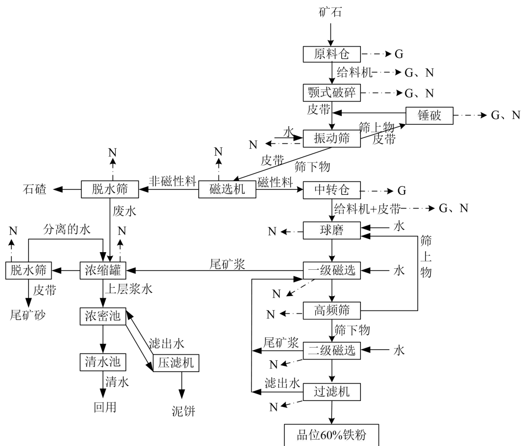
图 3.4-3 南厂区生产工艺流程及排污节点图
