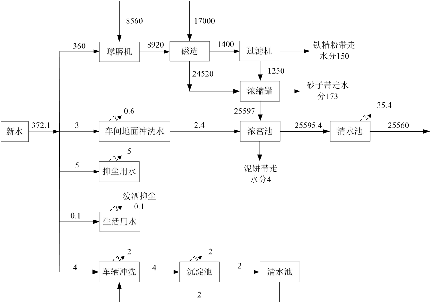
图 3.2-2 项目北厂区给排水平衡图 单位: m³/d
