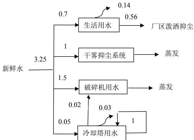
图 1 本项目生产给排水平衡图 单位： \text{m}^3/\text{d}
