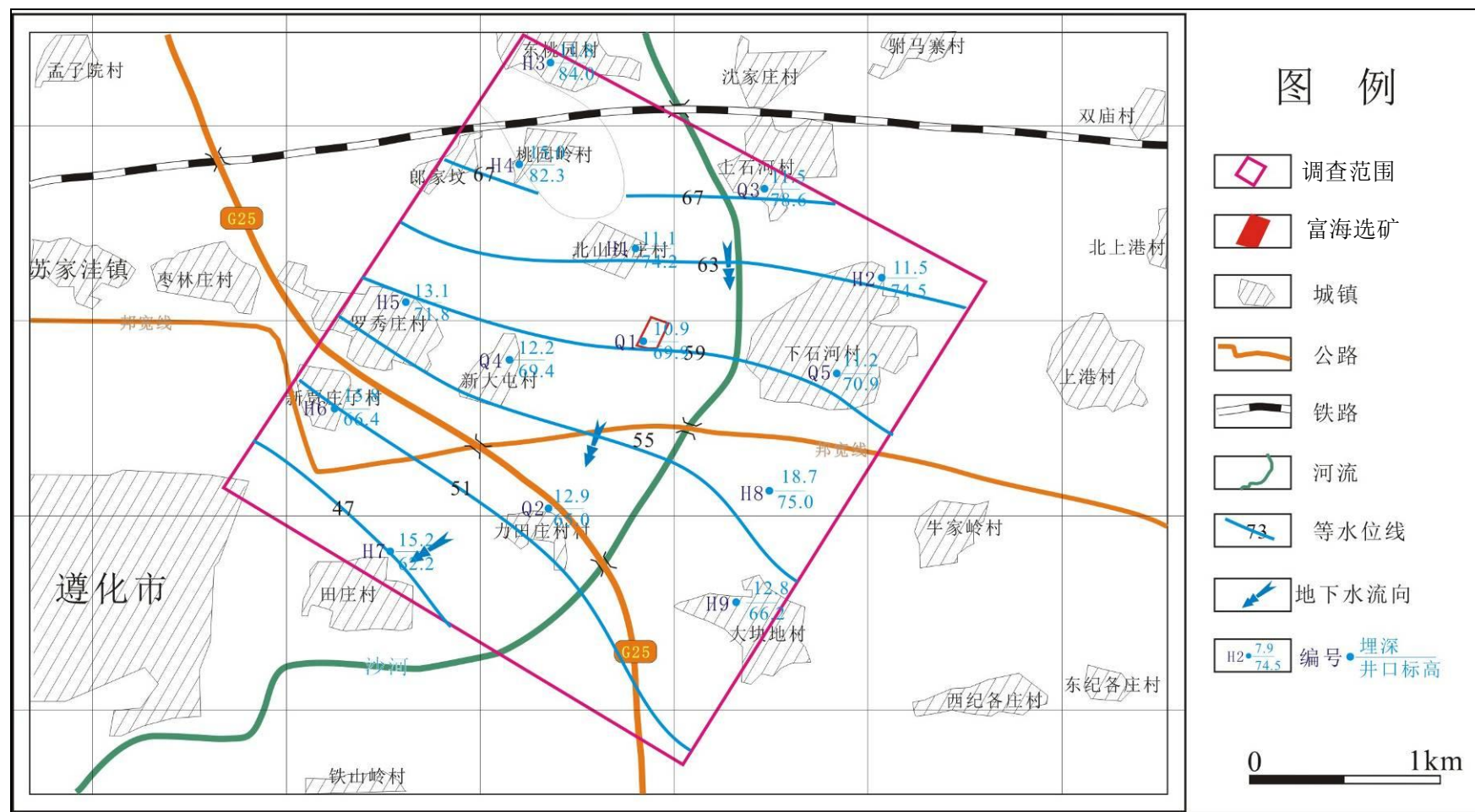
图 5.2-7 浅层地下水流场
