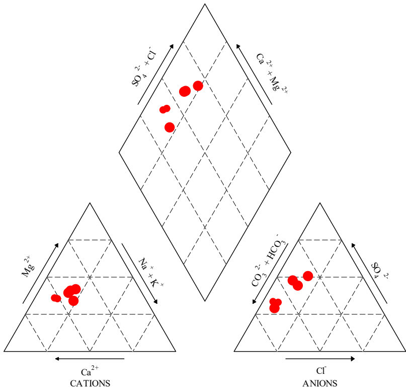
图 5.2-6 评价区水化学类型 piper 图
