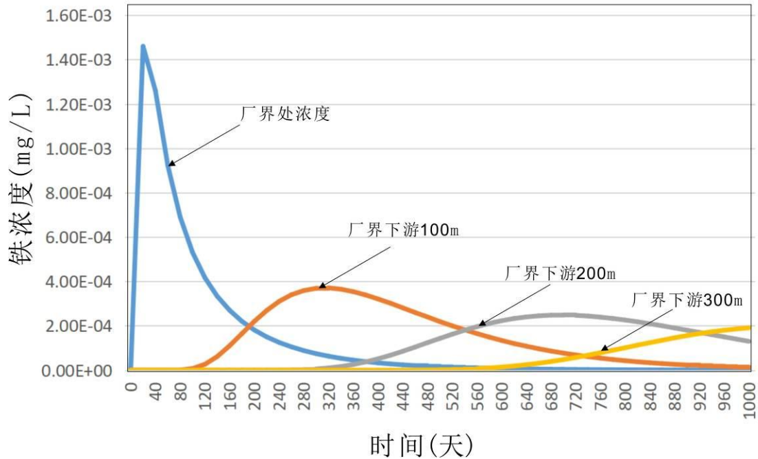
图 5.2-12 厂界、距厂界 100 米、200 米、300 米处铁浓度随时间变化过程线
