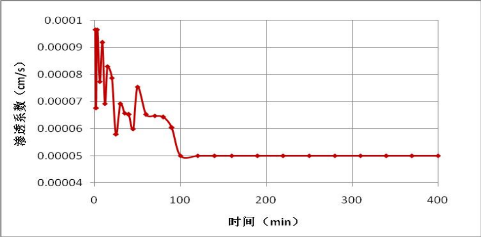
图 5.2-10 S-2 渗水试验成果图
