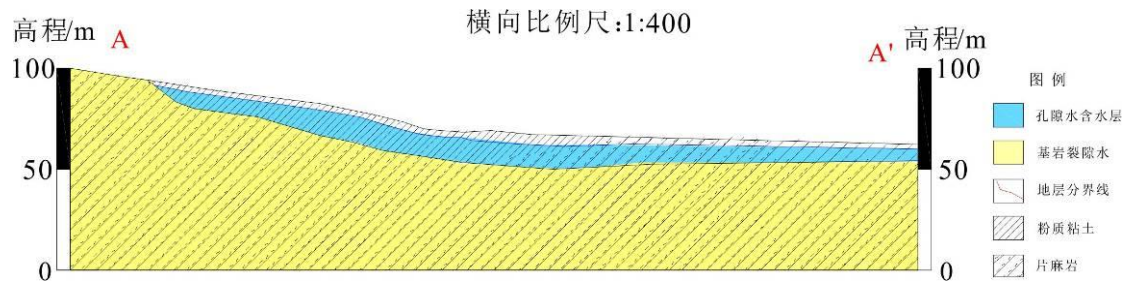
图 5.2-5 区域地质剖面图
