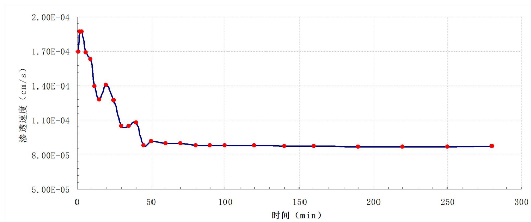
图 5.2-19 S-2 渗水试验成果图
