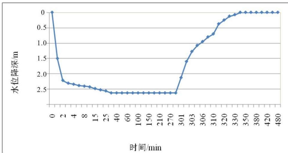
图5.2-16 力田庄村内抽水试验水位降深-时间曲线
