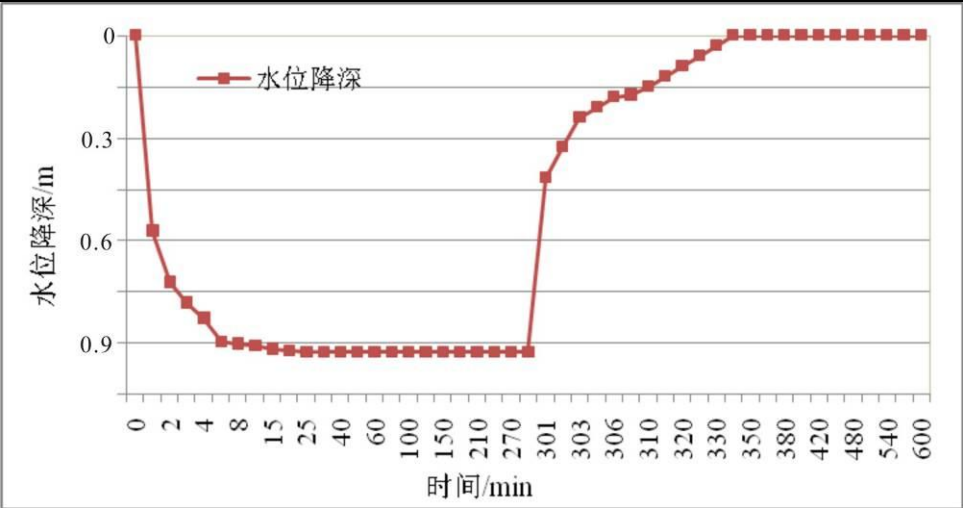
图5.2-11 项目厂区抽水试验降深-时间曲线
