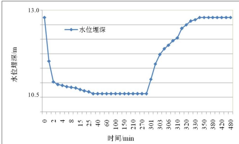
图5.2-15 力田庄村内抽水试验水位埋深-时间曲线
