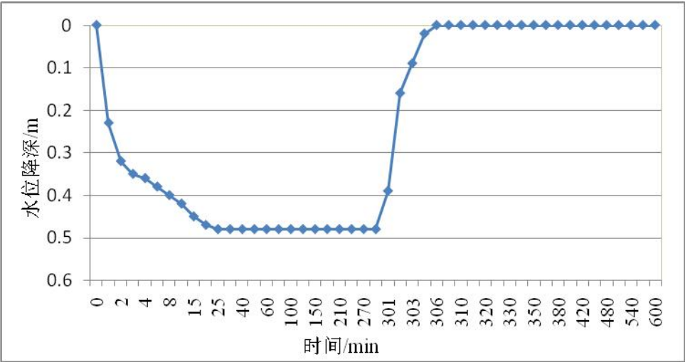
图5.2-13 北头山村抽水试验水位埋深-时间曲线
