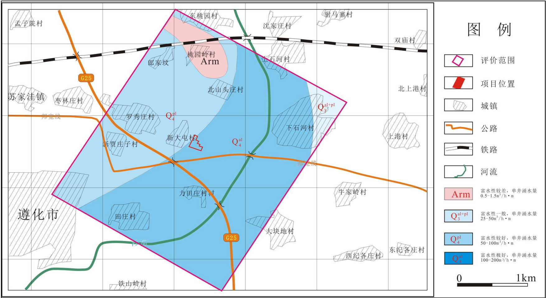
图 5.2-7 评价区水文地质图
