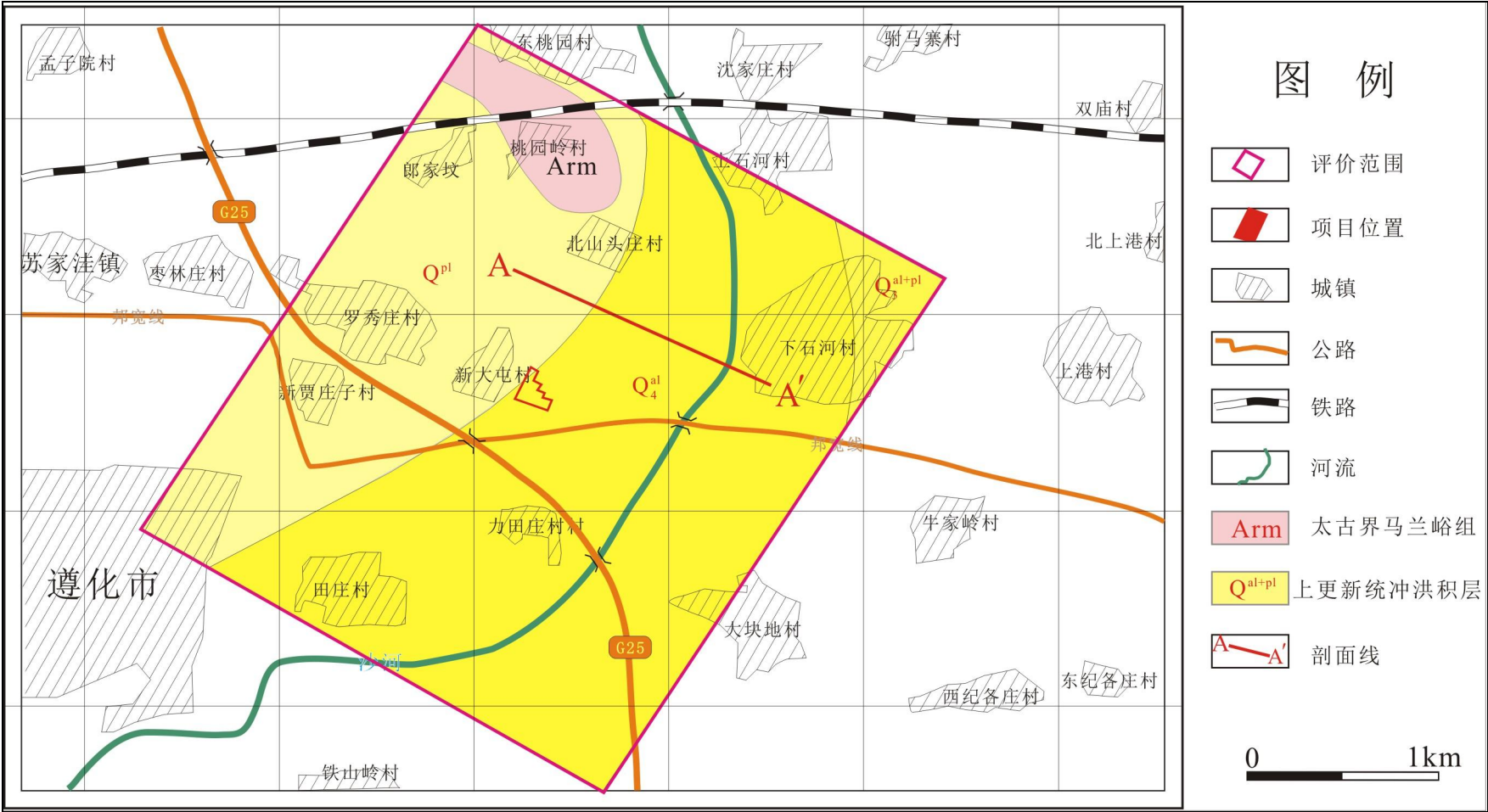
图 5.2-5 评价区地质图
