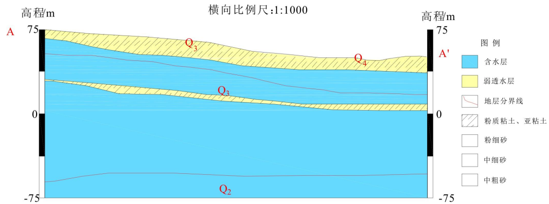
图 5.2-6 评价区地质图及剖面图
