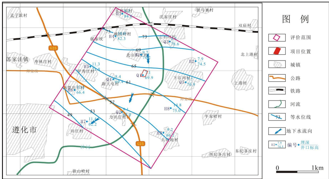
图 5.2-9 11 月 浅层地下水流场
