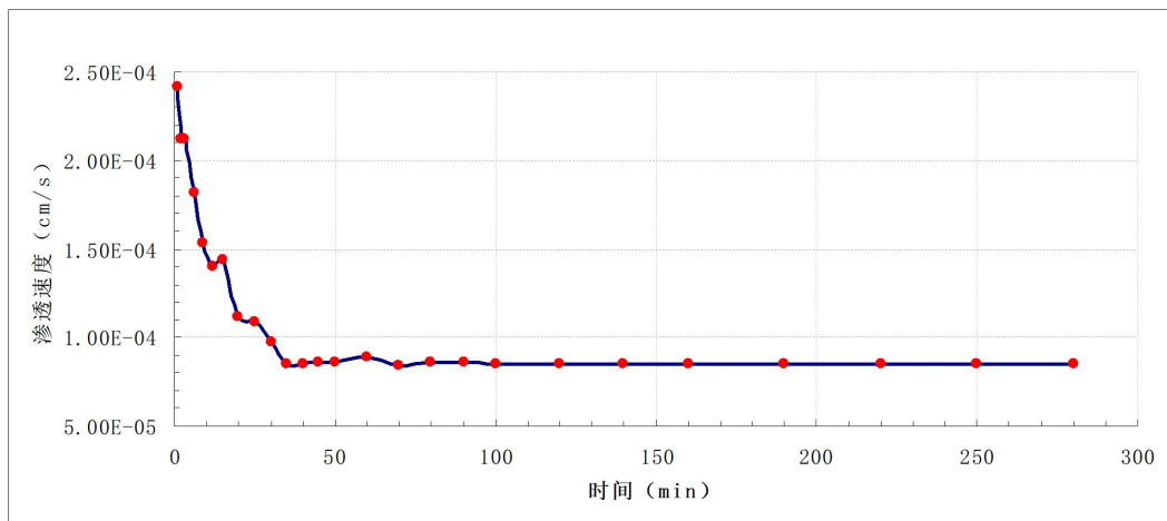
图 5.2-20 S-3 渗水试验成果图
