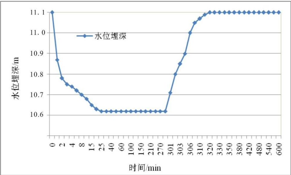
图5.2-14北头山村抽水试验水位降深-时间曲线
