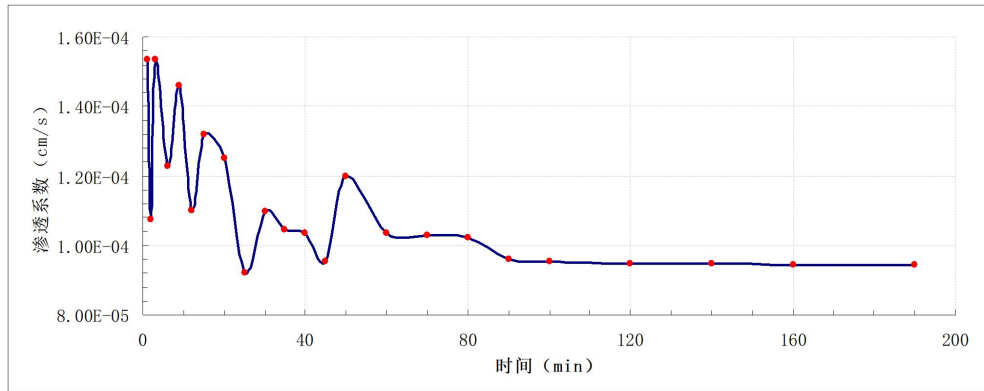
图 5.2-18 S-1 渗水试验成果图
