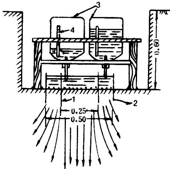
图5.2-17 双环渗水试验原理图
