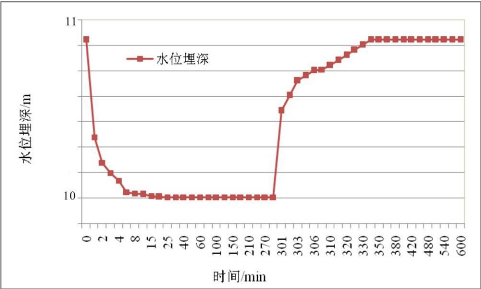
图5.2-12 项目厂区抽水试验水位埋深-时间曲线
