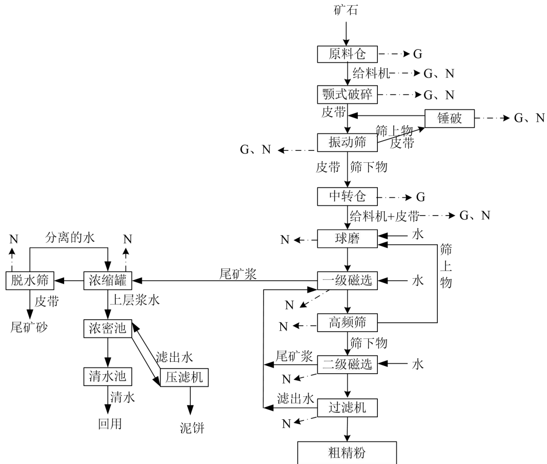
图 3.4-2 项目粗选生产工艺流程及排污节点图
