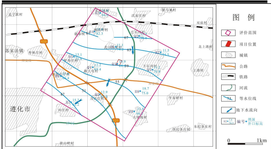
图 5.2-8 9 月浅层地下水流场
