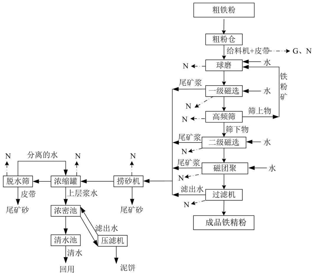
图 3.4-3 精选线工艺流程及排污节点图
