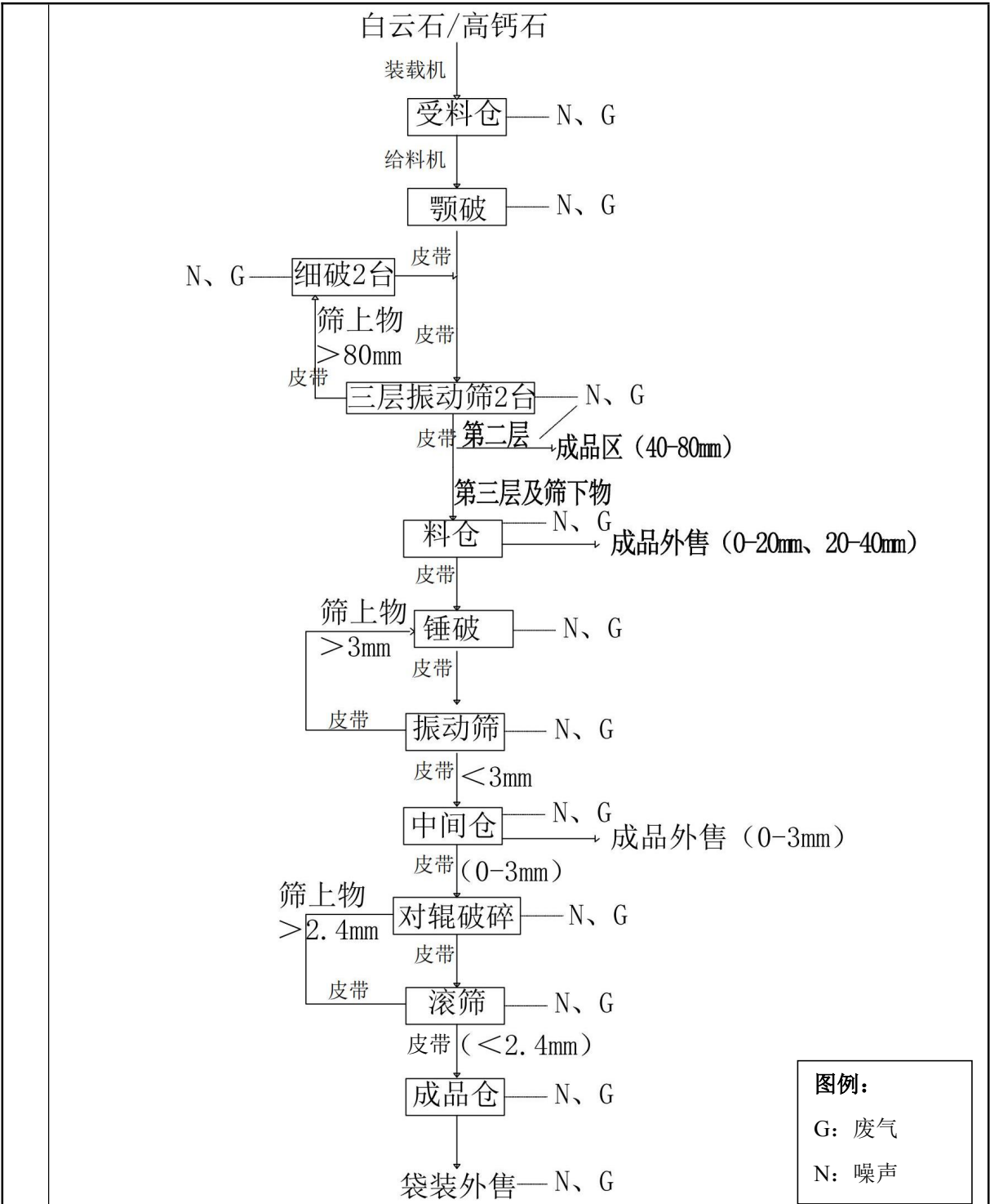
图 2-2 白云石及高钙石加工工艺流程及排污节点图
