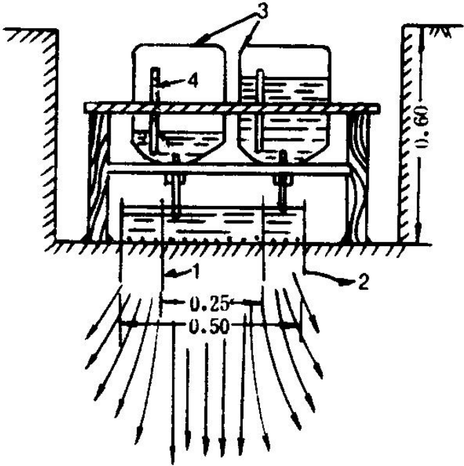
图5.2-14双环渗水试验原理图
