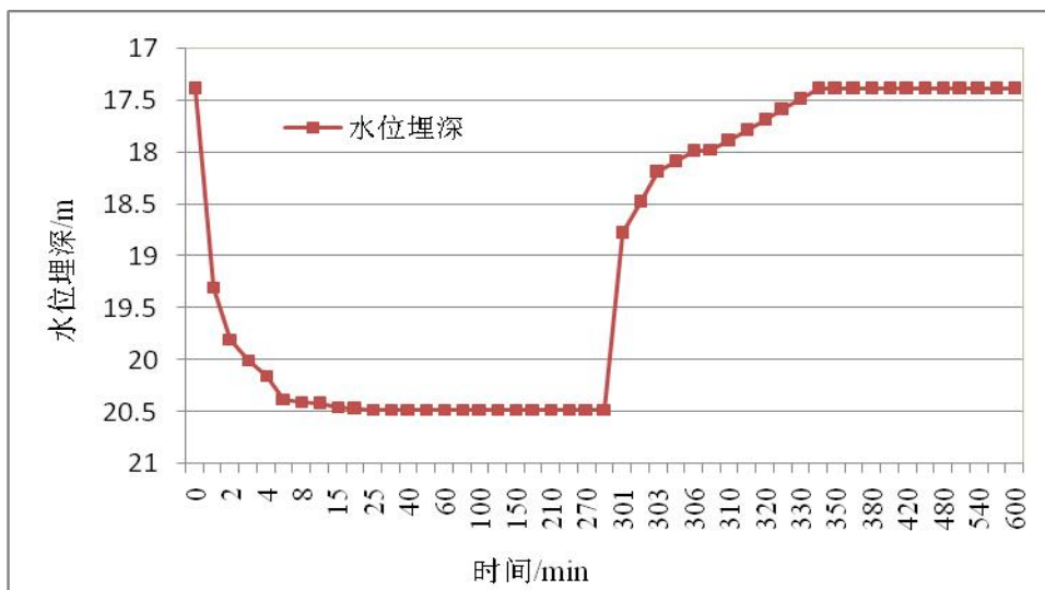
图5.2-9西新店子抽水试验水位埋深-时间曲线
