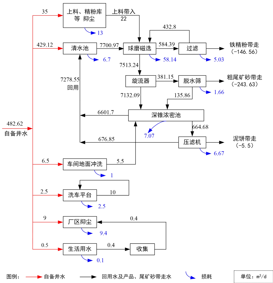
图 3.1-1 现有工程水平衡图
