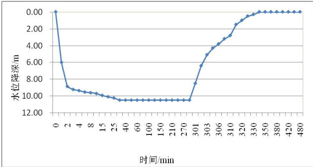
图5.2-13 大曹各寨村内抽水试验水位降深-时间曲线
