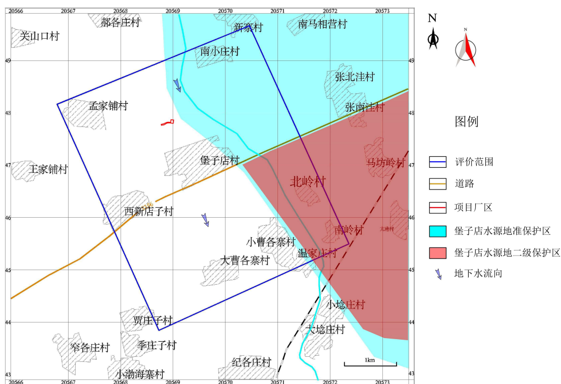
图 2.4-1 地下水评价范围图
