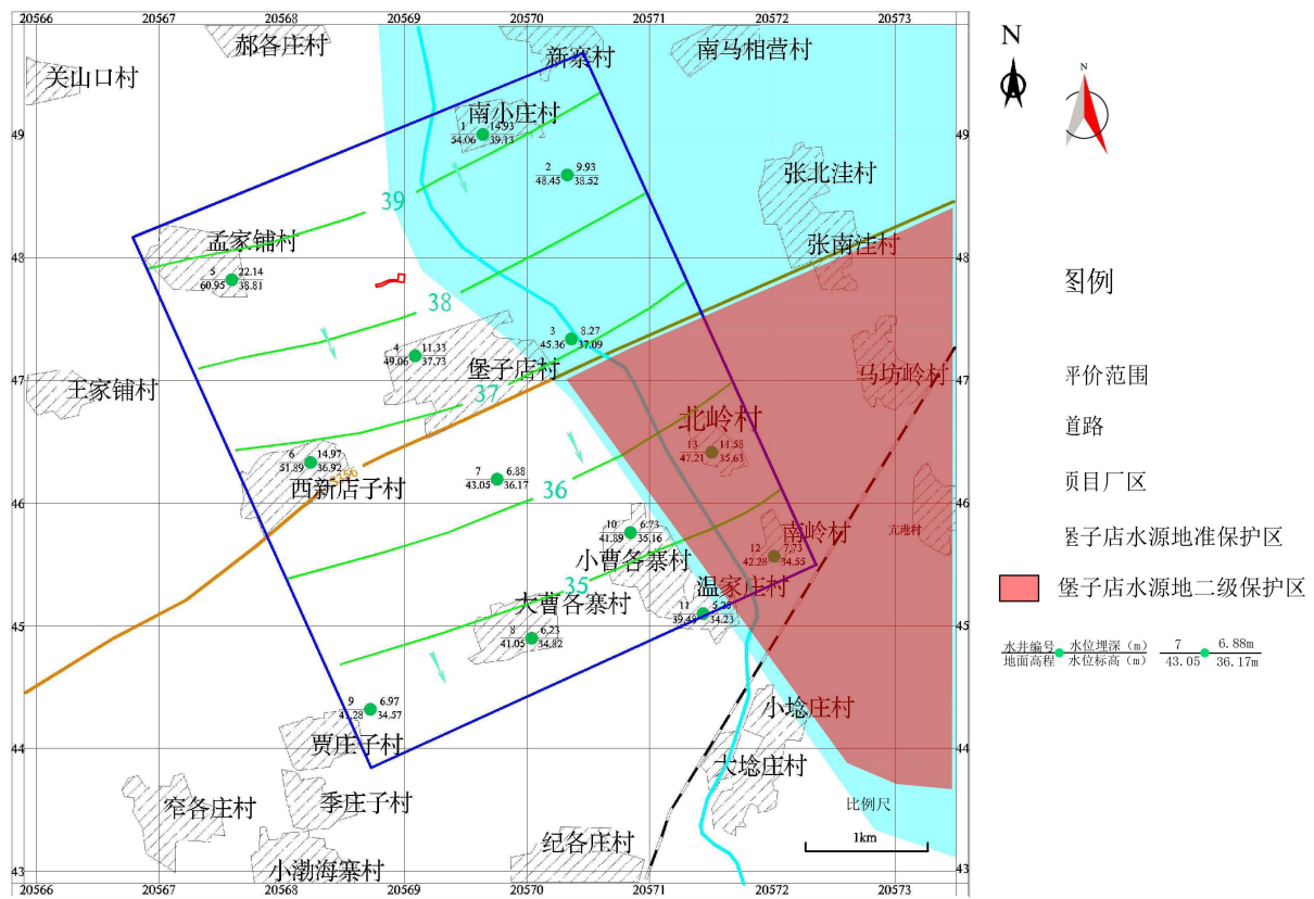
图 5.2-8 丰水期等水位线图
