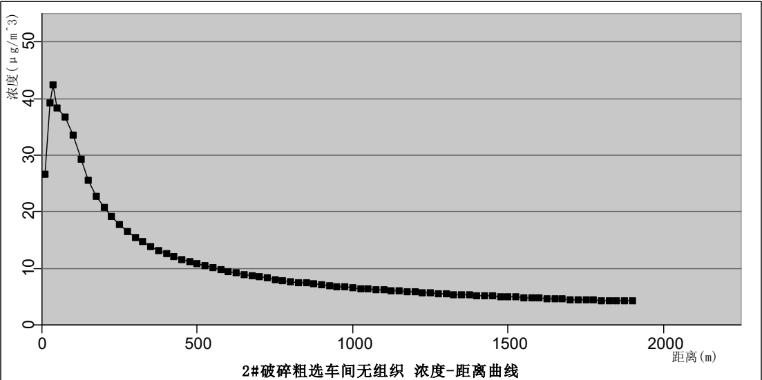
图 5.2-4 2#破碎粗选车间无组织废气浓度距离曲线图 \mu\text{g}/\text{m}^3
