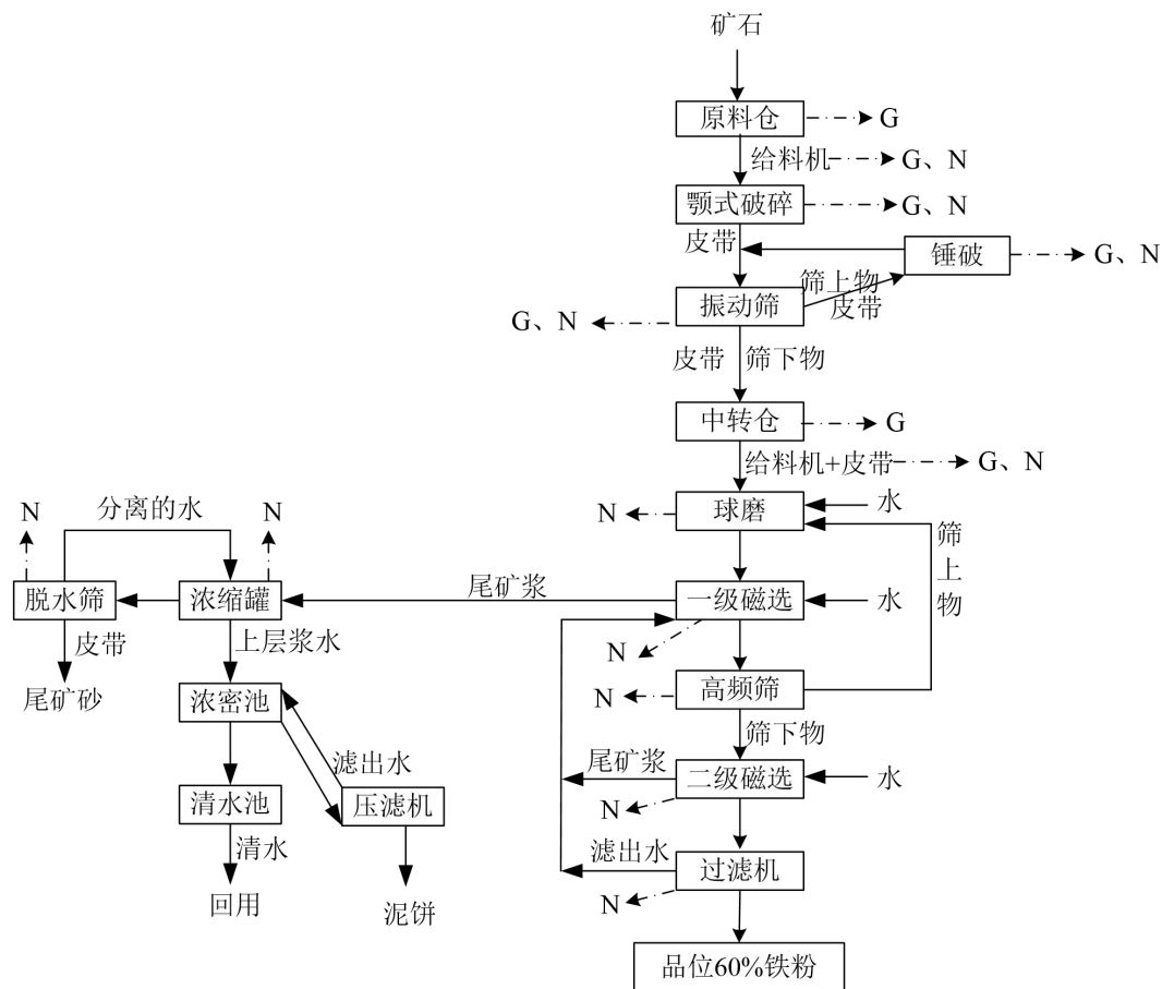
图 3.3-1 1#破碎粗选车间生产工艺流程及产排污环节分析
