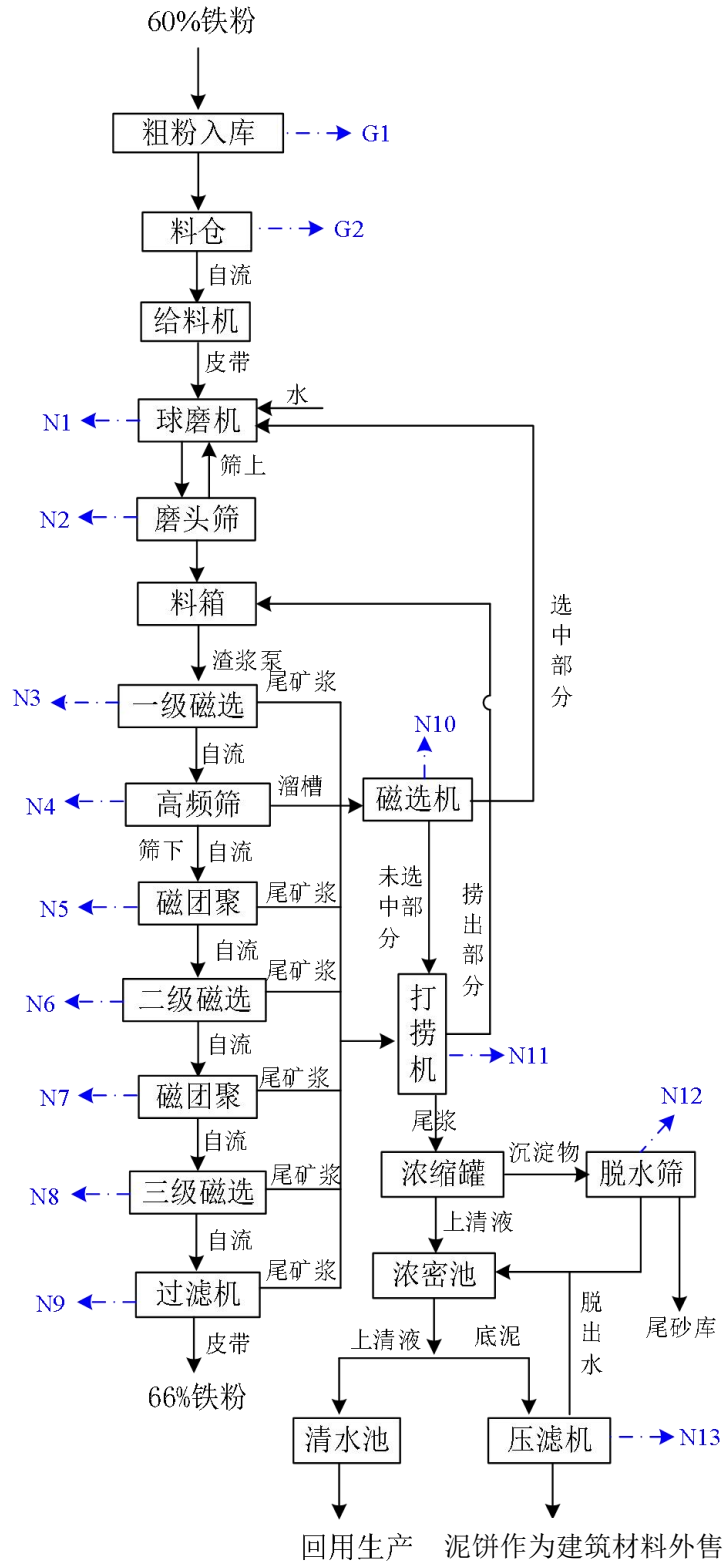
图 3.3-3 精选线生产工艺流程及产排污环节分析
