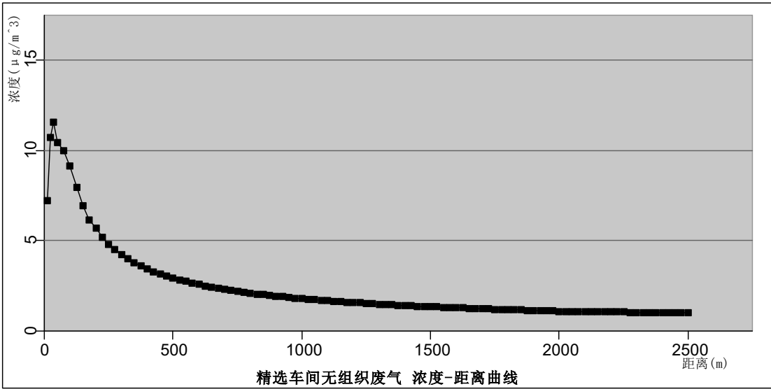
图 5.2-5 精选车间无组织废气浓度距离曲线图 \mu\text{g}/\text{m}^3
