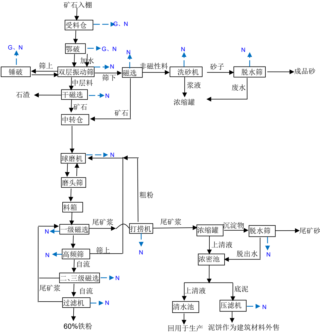
图 3.3-2 2#破碎粗选车间生产工艺流程及产排污环节分析
