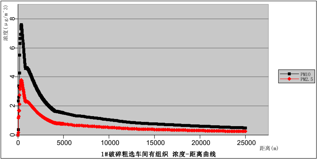
图 5.2-1 1#破碎粗选车间破碎线有组织废气浓度距离曲线图 \mu\text{g}/\text{m}^3
