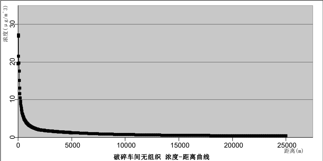
图 5.2-2 2#破碎粗选车间破碎线有组织废气浓度距离曲线图 \mu\text{g}/\text{m}^3
