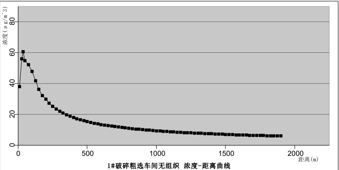
图 5.2-3 1#破碎粗选车间无组织废气浓度距离曲线图 \mu\text{g}/\text{m}^3
