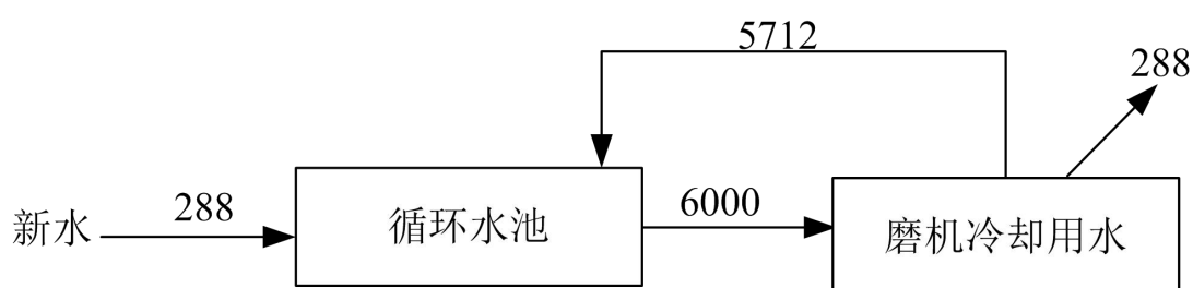
图3 本项目生产给排水平衡图 单位： \text{m}^3/\text{d}
