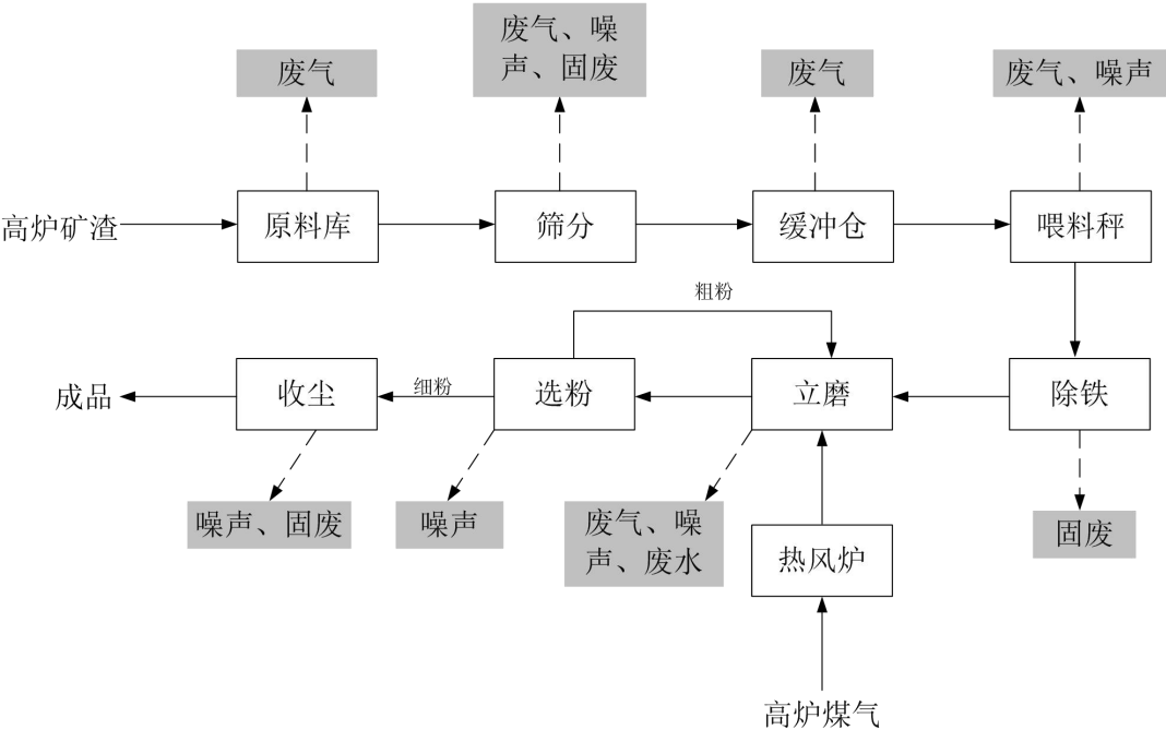
图 2 现有工程工艺流程及产排污节点图
