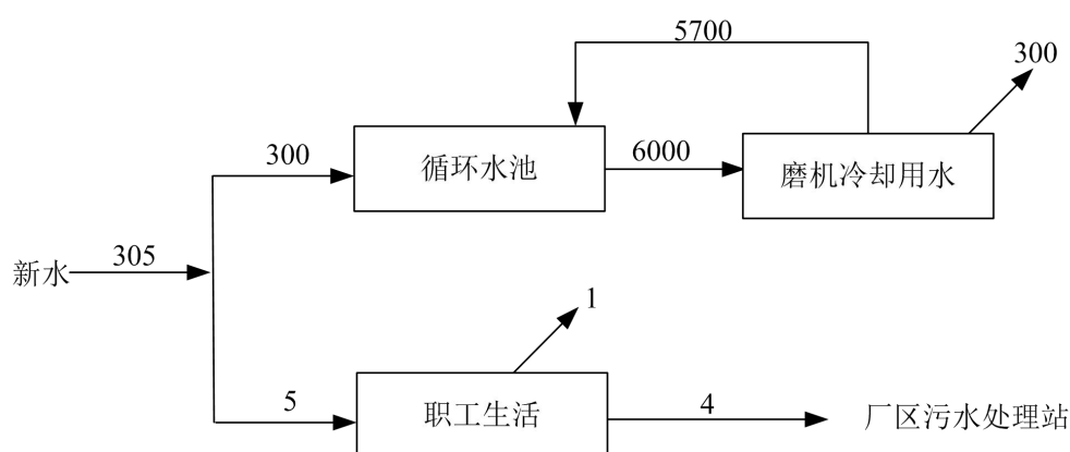
图 1 现有工程生产给排水平衡图 单位：m 3 /d
