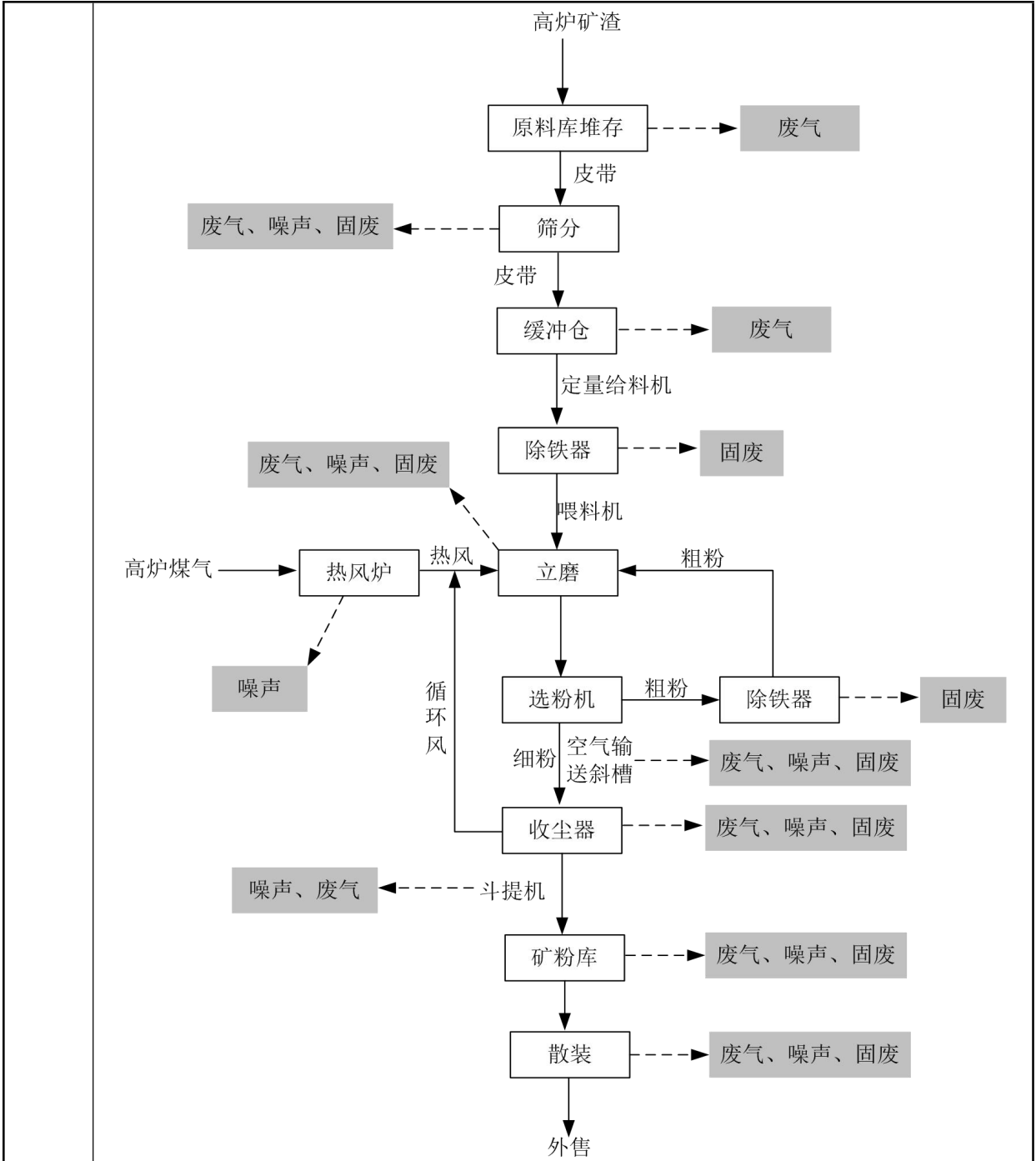
图 5 项目生产工艺及产排污节点图
