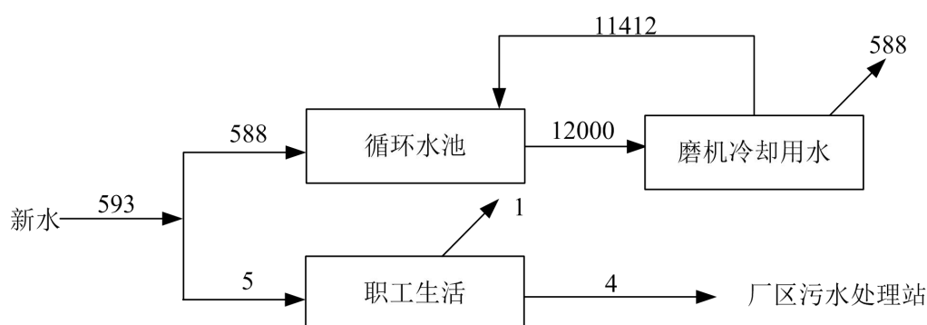
图4 项目建成后全厂矿渣微粉生产线水平衡图 单位： \text{m}^3/\text{d}
