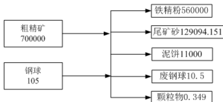
图 3.4-1 物料平衡图 (t/a)
