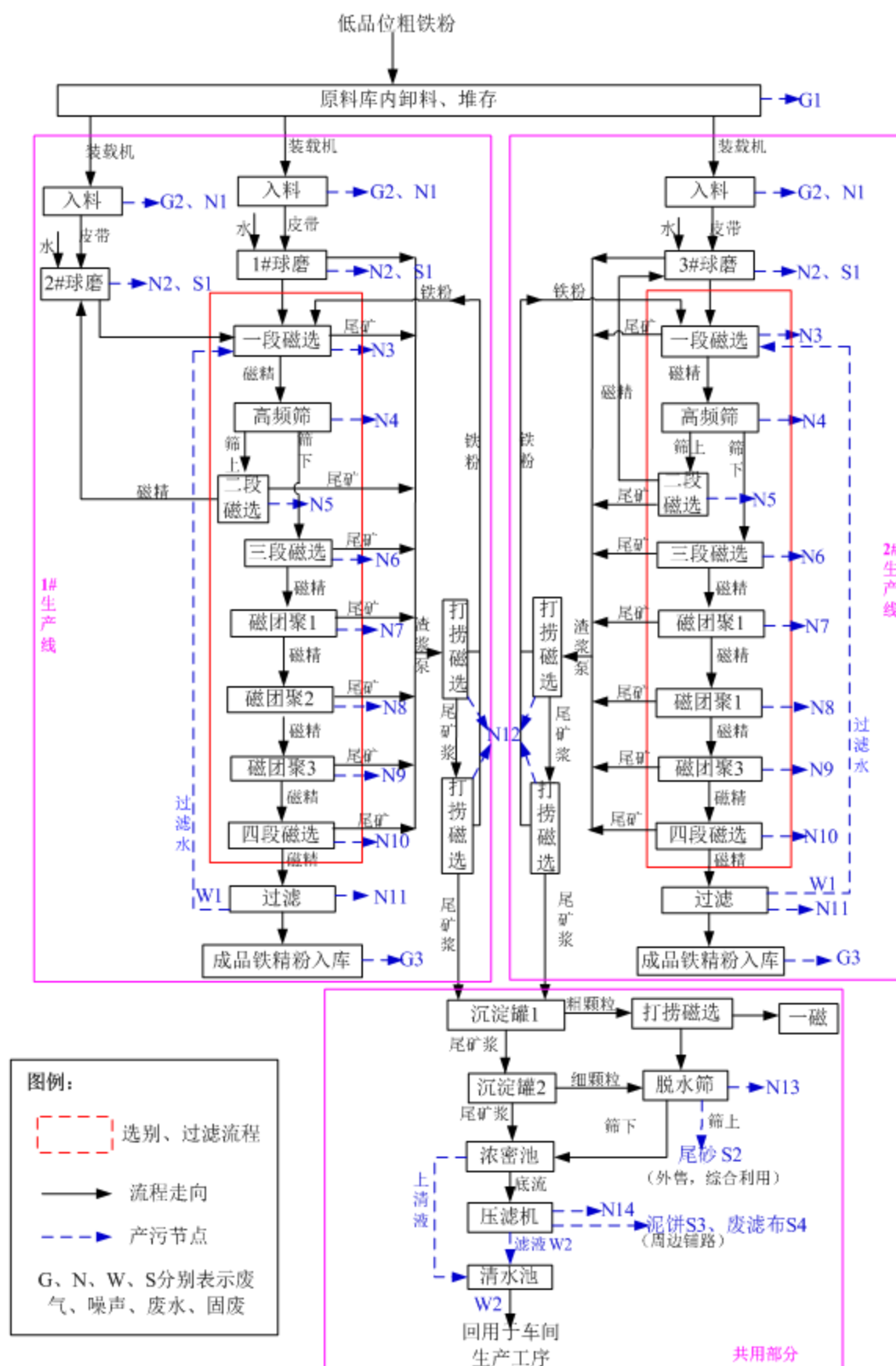
图 3.5-1 生产工艺流程及排污节点图
