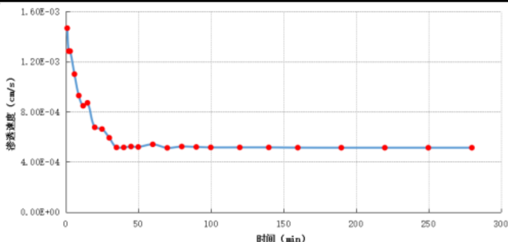
图 5.2-9 S2 渗水试验成果图
