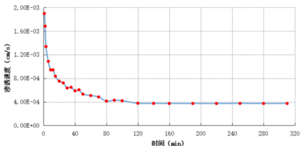
图 5.2-8 S1 渗水试验成果图
