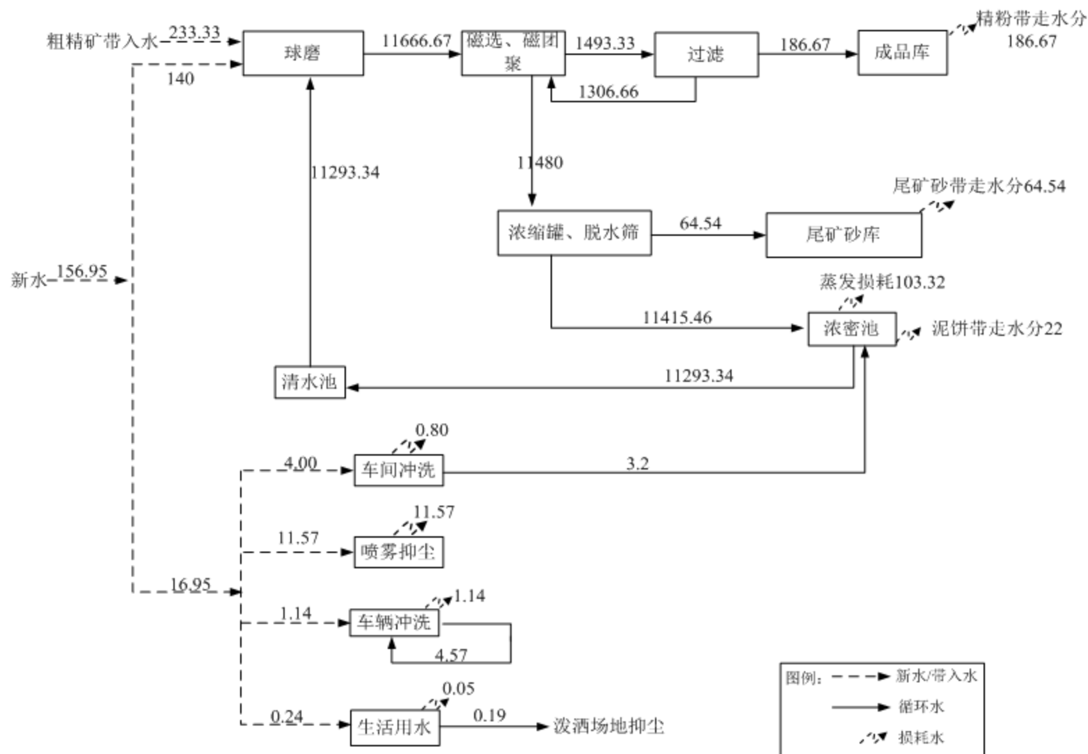
图 3.3-1 项目给排水平衡图 单位: \text{m}^3/\text{d}
