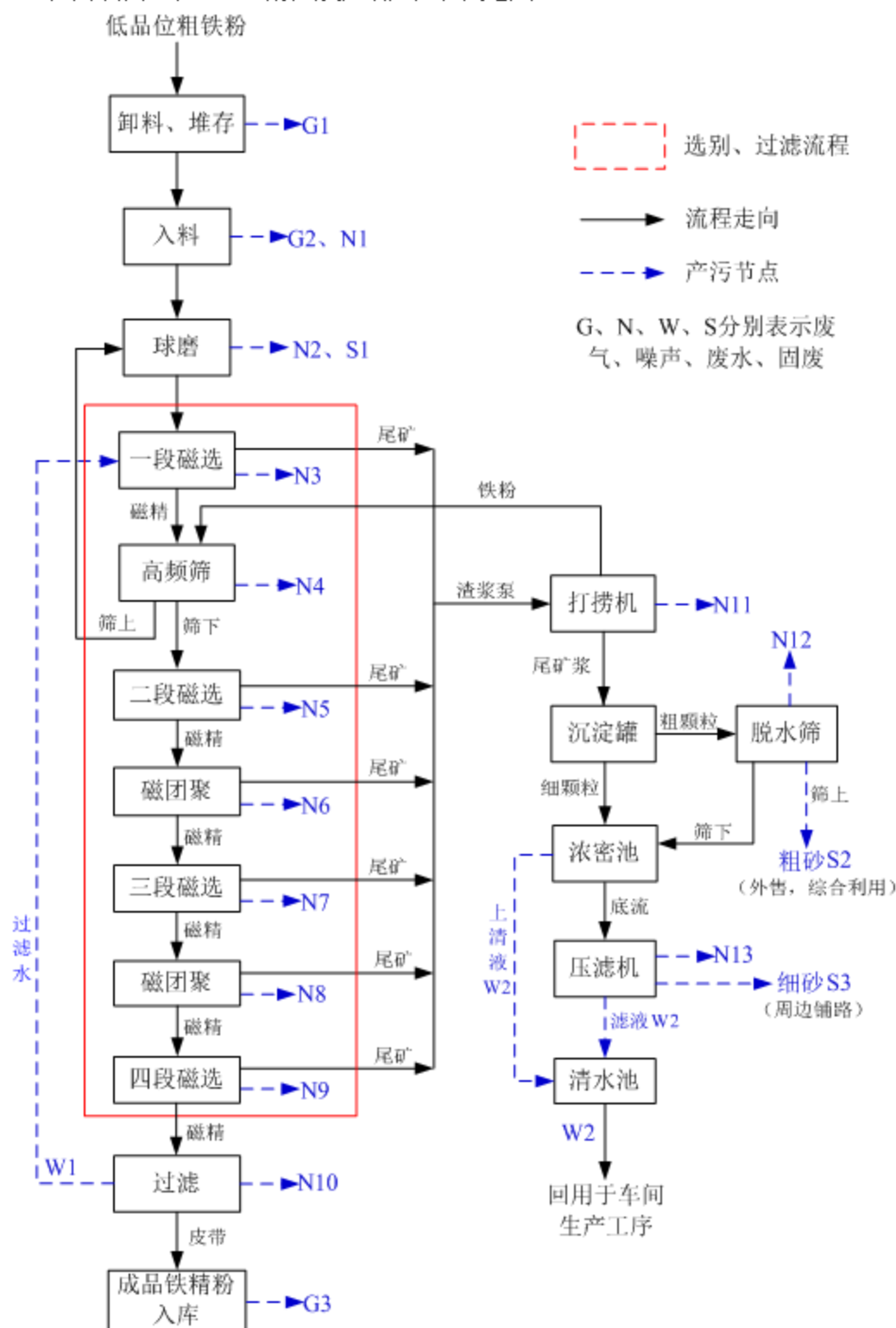
图 3.1-1 现有工程生产工艺流程及产排污环节分析
