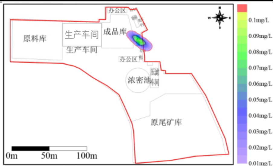
A. 10 天影响预测图
