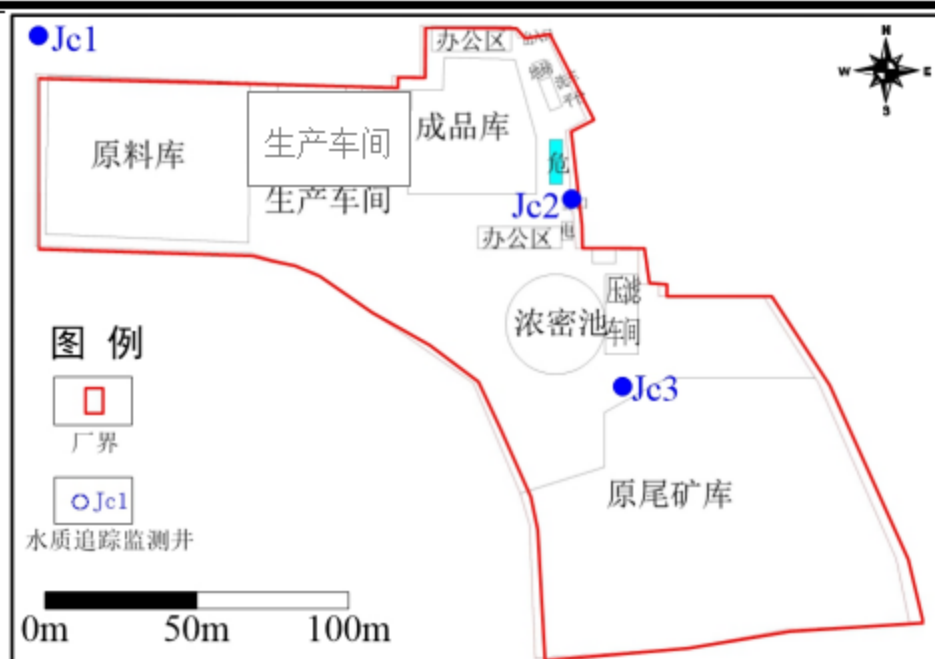
图 5.2-18 地下水监测点布置图
