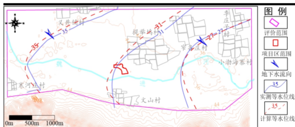
图 5.2-13 2024 年 10 月 26 日潜水等水位线拟合图
