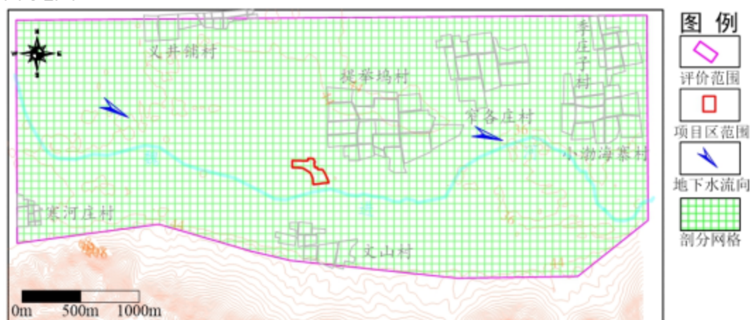
图 5.2-11 模拟区网格剖分图
