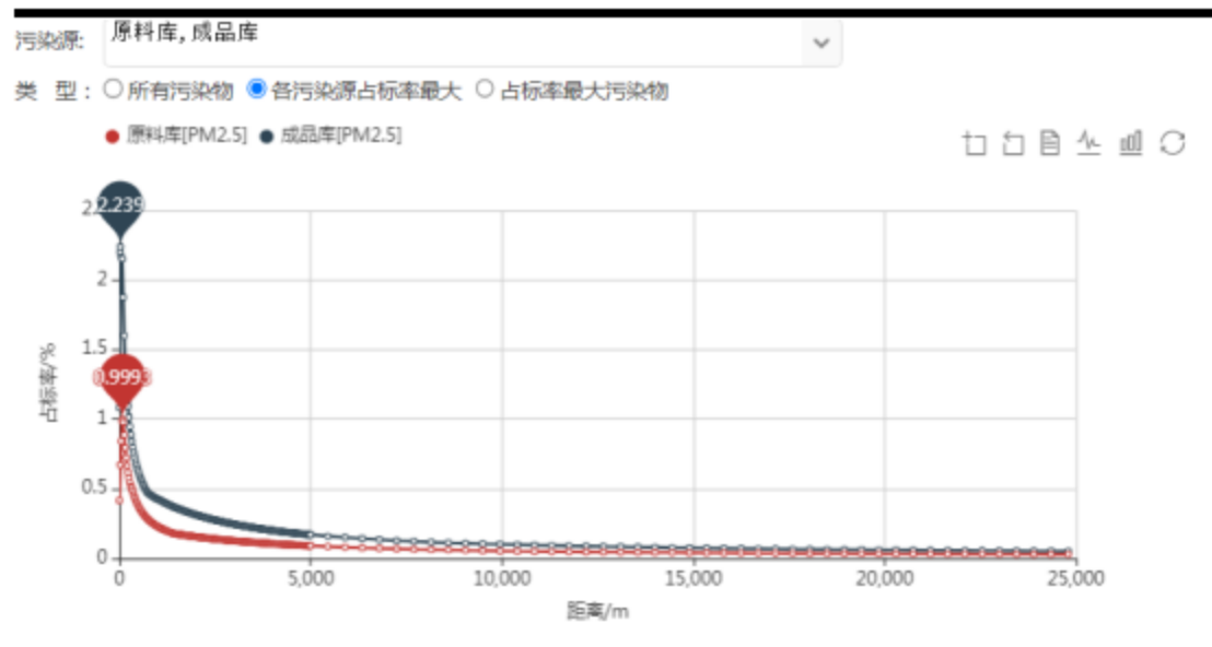
图 2.4.2 污染物最大占标率预测结果折线图
