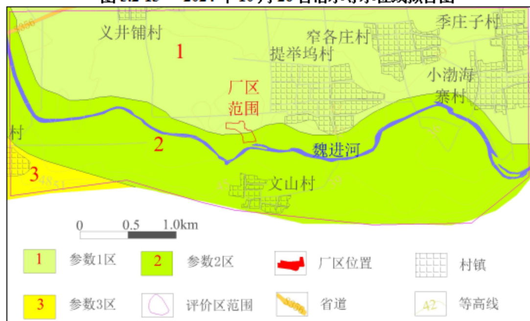
图 5.2-14 浅层含水层参数分区图
