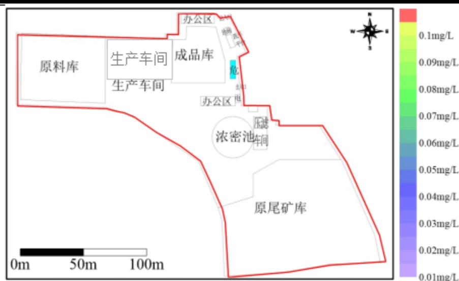
D. 150 天影响预测图
