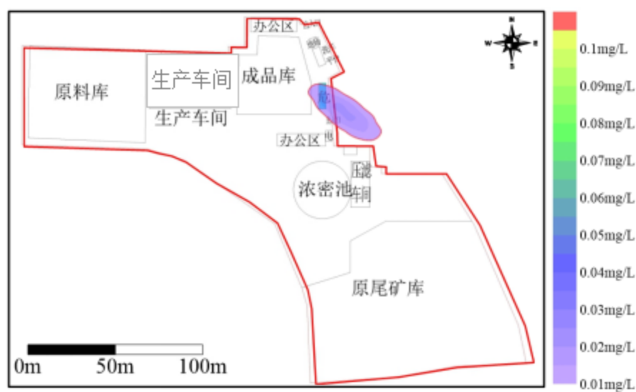
B. 50 天影响预测图
