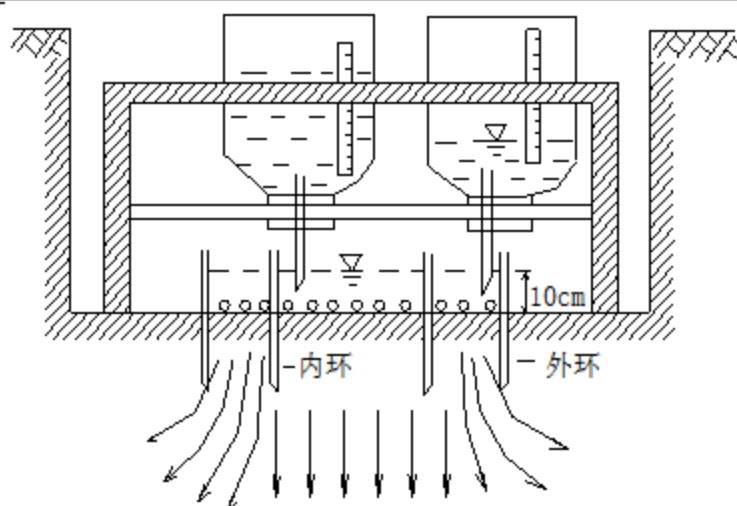
图 5.2-7 双环渗水试验原理图
