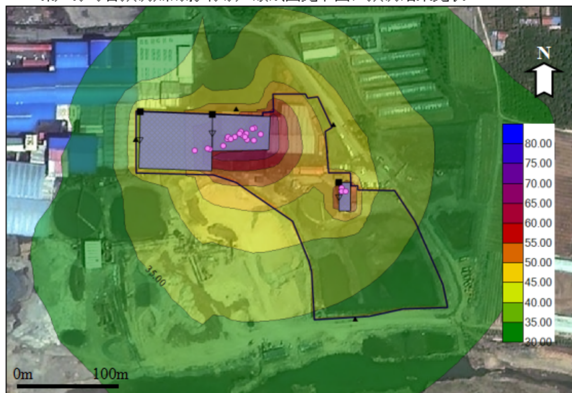
图 5.2-19 项目噪声预测等声级线图
