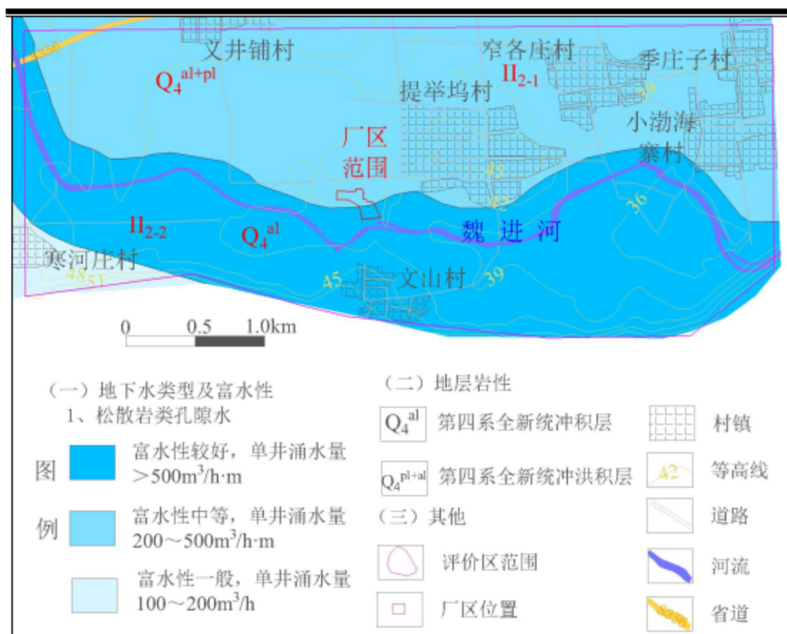
图 5.2-3 评价区水文地质图
