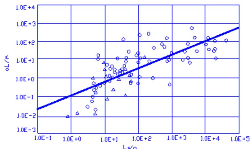
图 5.2-15 孔隙介质 2 维数值模型的 \lg \alpha_L - \lg L/n 图
