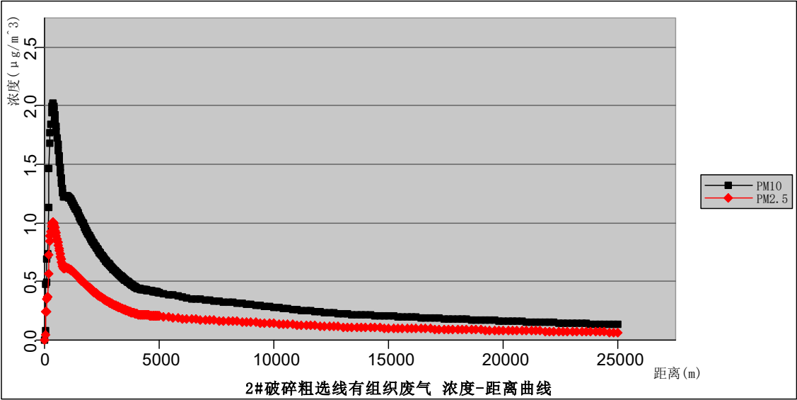
图 5.2-2 2#破碎粗选线有组织废气浓度距离曲线图 \mu\text{g}/\text{m}^3
