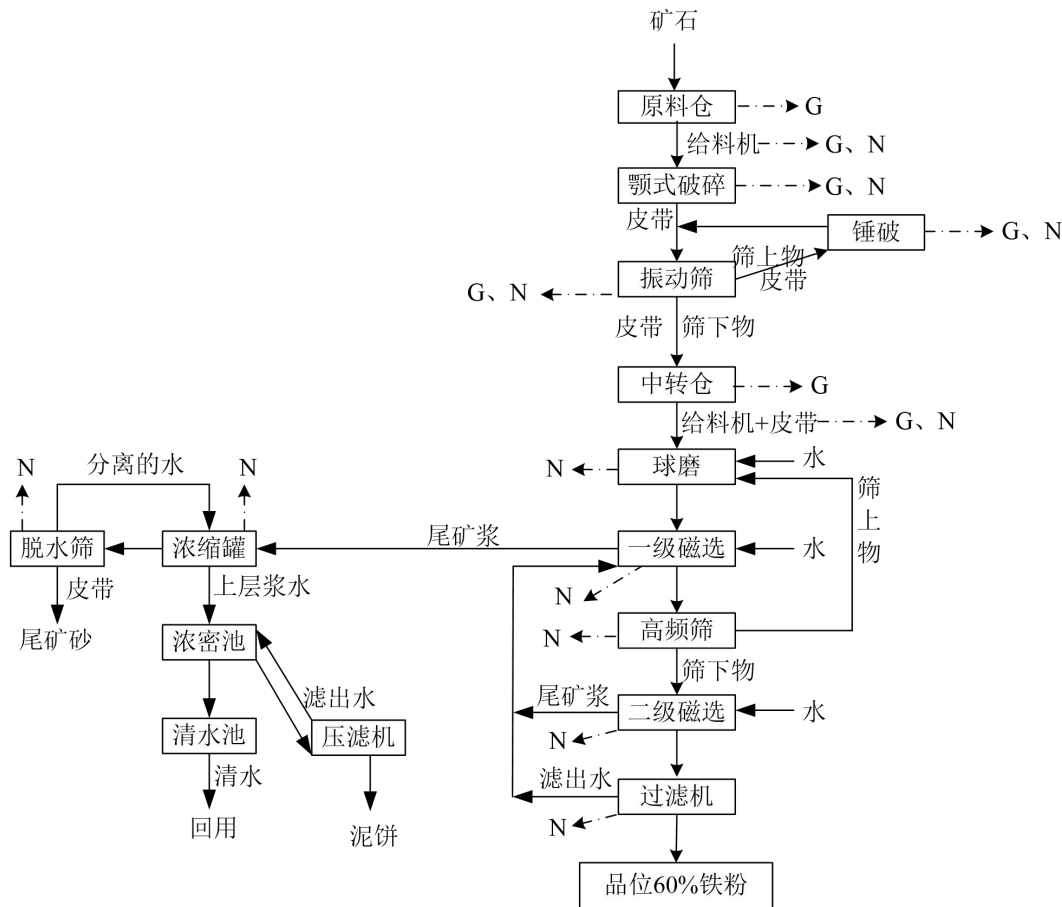
图 3.3-1 1#破碎粗选线生产工艺流程及产排污环节分析
