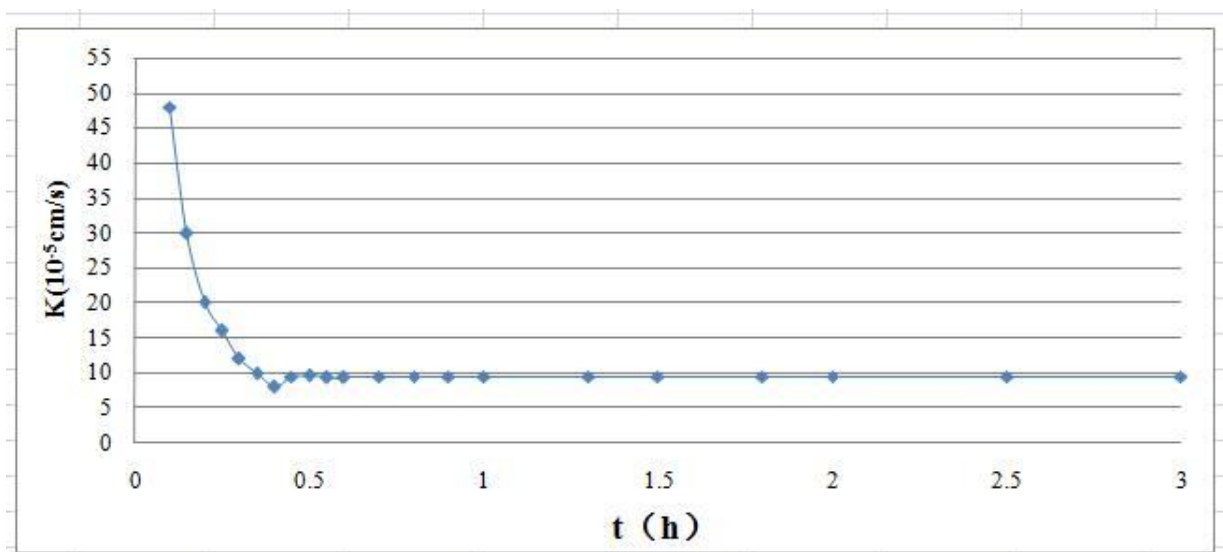
图 5.2-9 渗透系数与时间关系曲线图
