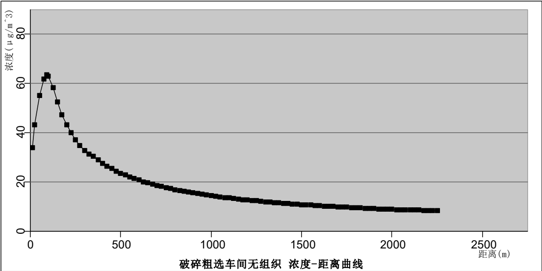
图 5.2-3 破碎粗选车间无组织废气浓度距离曲线图 \mu\text{g}/\text{m}^3
