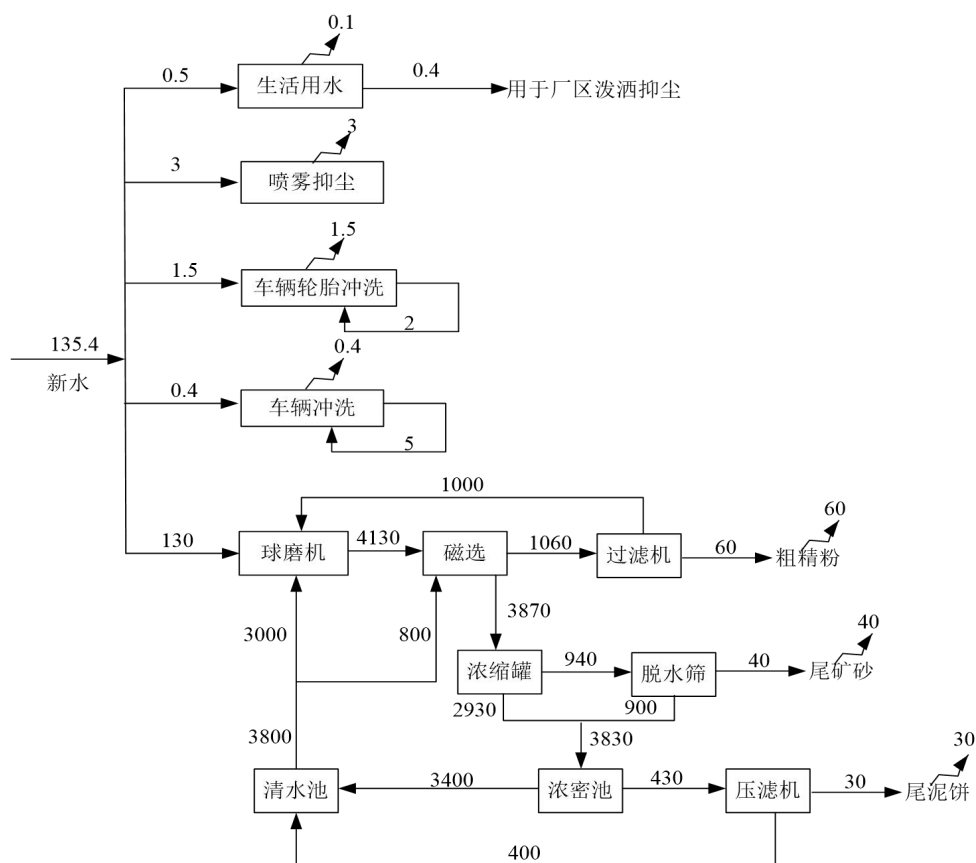
图 3.1-1 现有工程水平衡图
