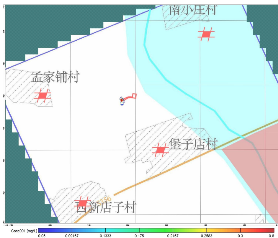
图 5.2-14 铁运移 100 天迁移范围图
