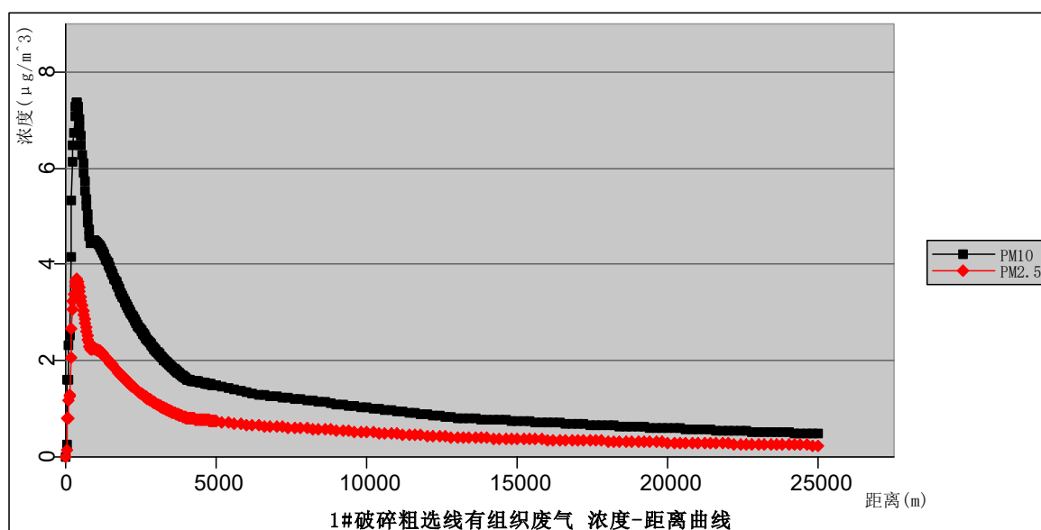
图 5.2-1 1#破碎粗线有组织废气浓度距离曲线图 \mu\text{g}/\text{m}^3
