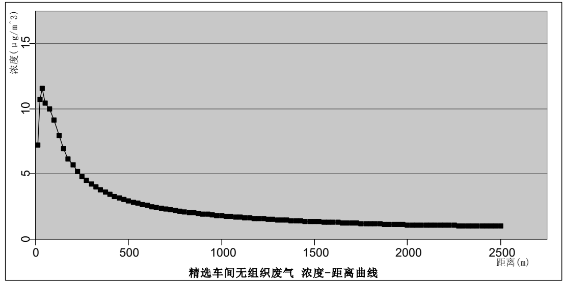
图 5.2-4 精选车间无组织废气浓度距离曲线图 \mu\text{g}/\text{m}^3
