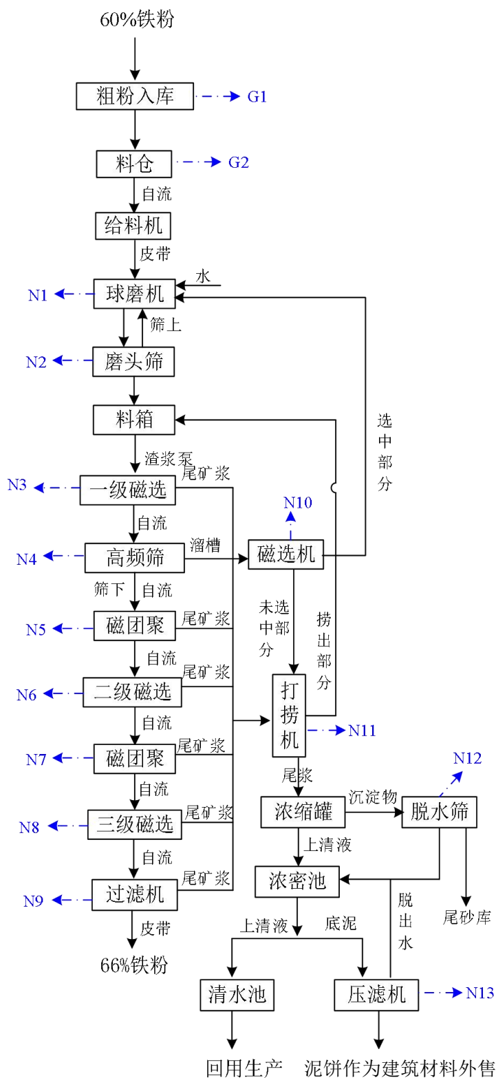
图 3.3-3 精选线生产工艺流程及产排污环节分析
