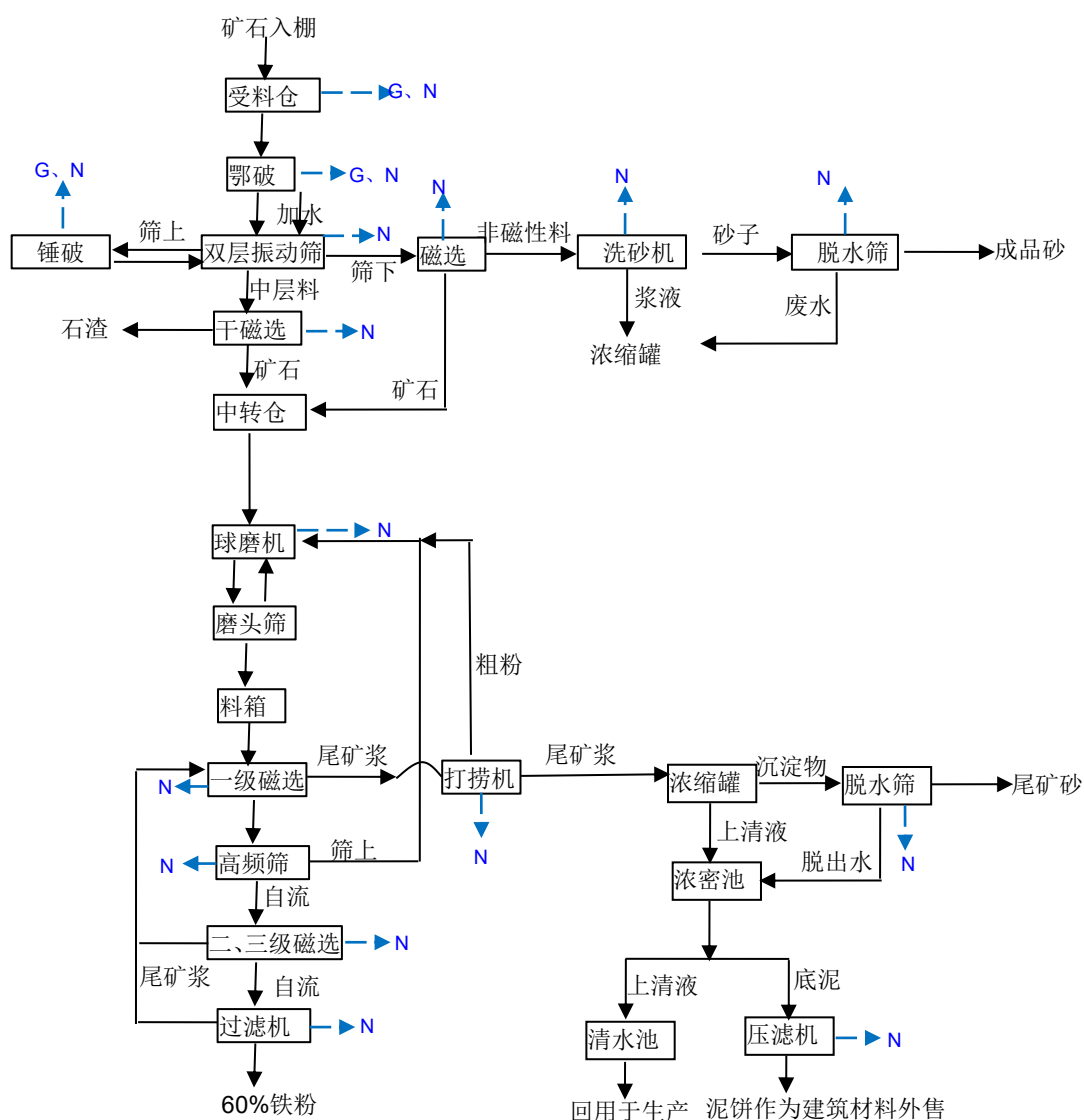
图 3.3-2 2#破碎粗选线生产工艺流程及产排污环节分析
