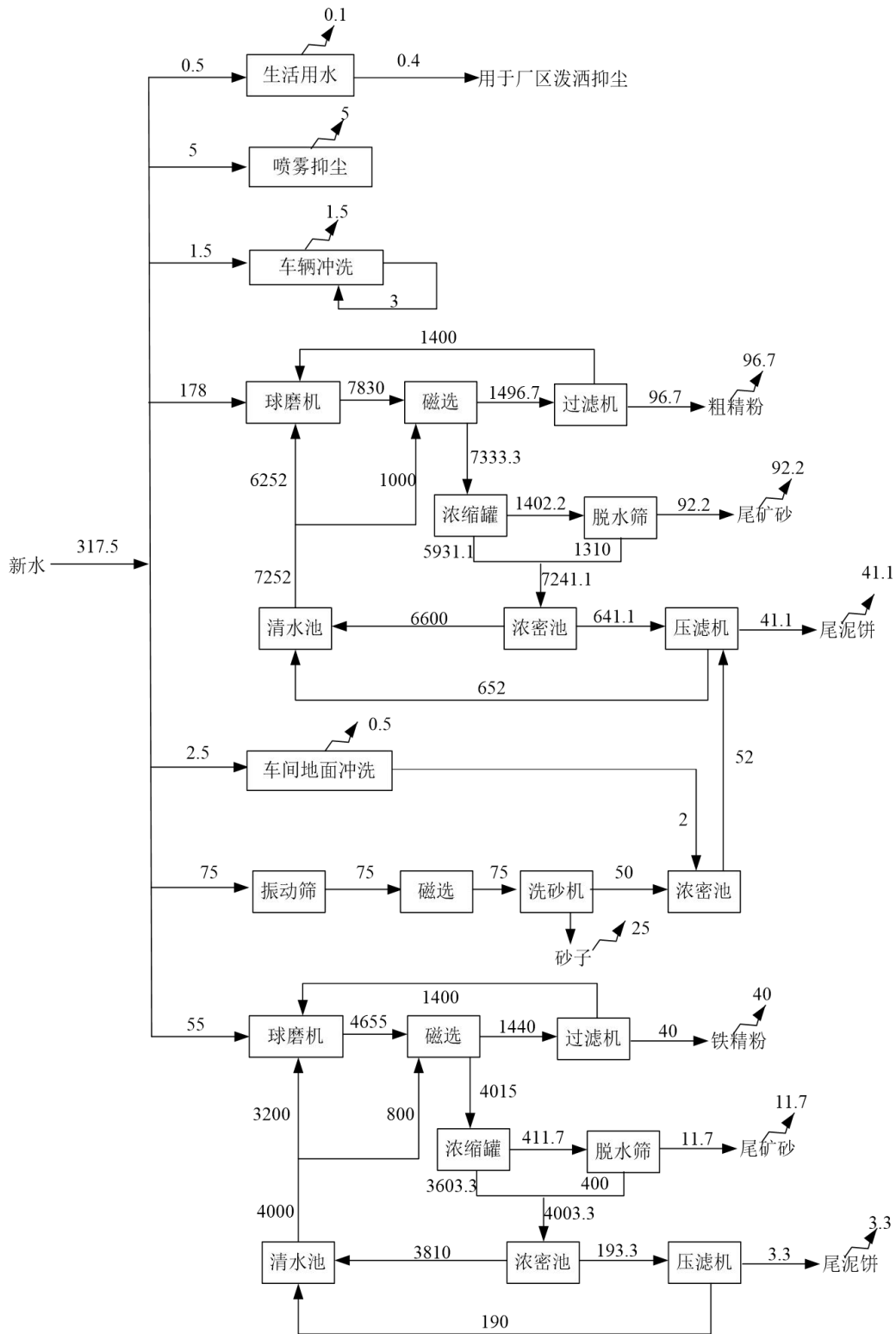
图 3.2-1 改扩建项目实施后全厂水平衡图 m³/d
