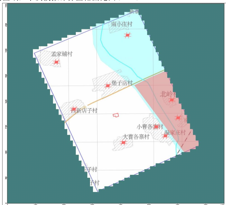
图 5.2-10 模拟计算区范围示意图
