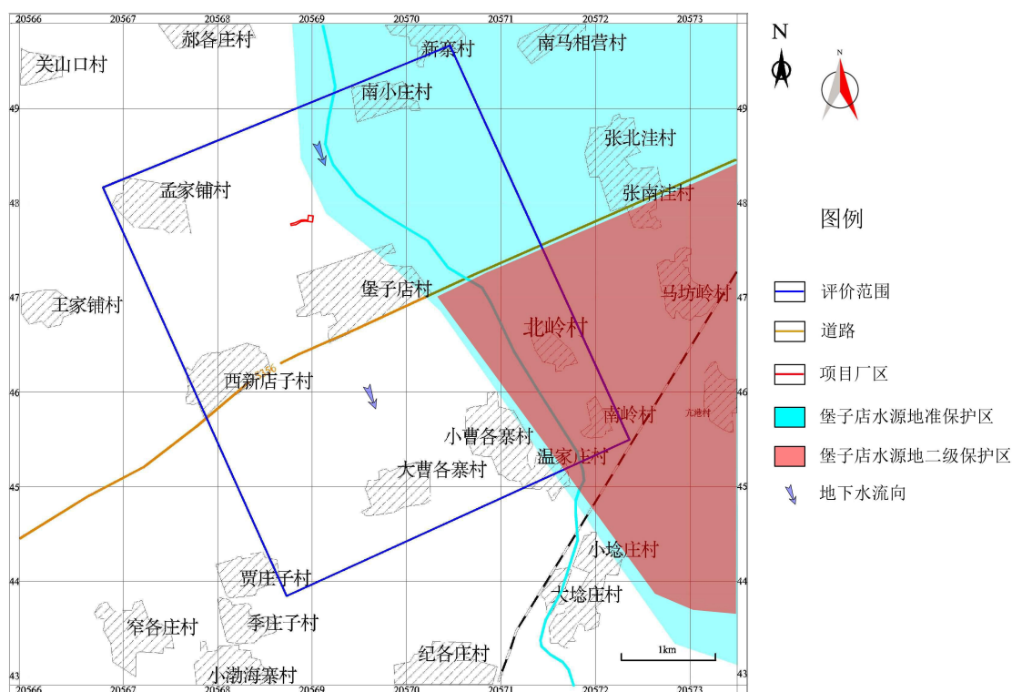
图 2.4-1 地下水评价范围图
