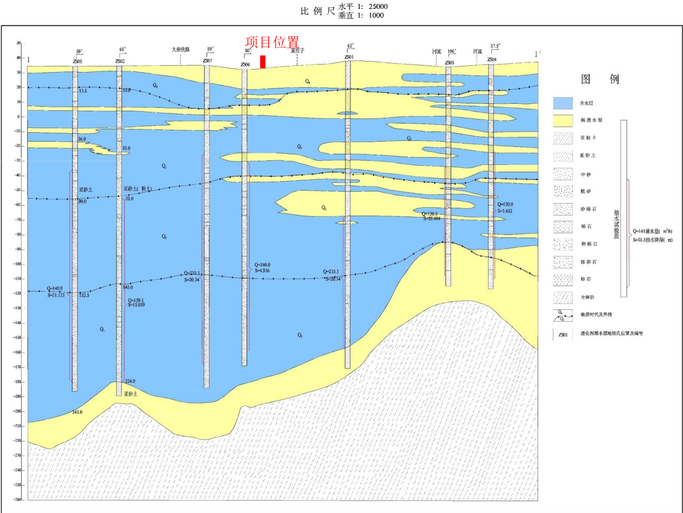
图 5.2-6 评价区水文地质剖面图
