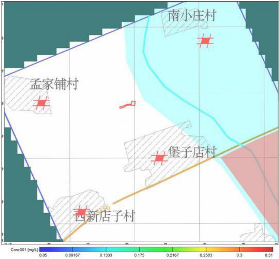
图 5.2-16 铁运移 1000 天迁移范围图
