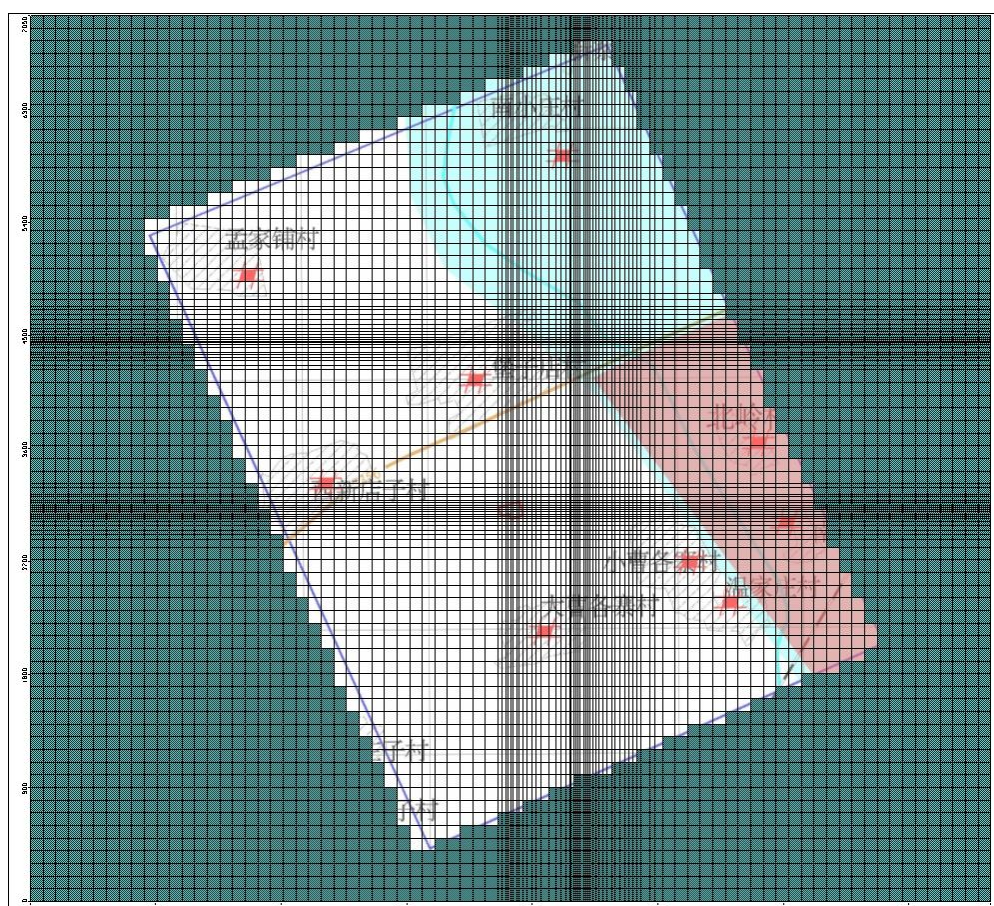
图 5.2-11 模拟区域网格平面图
