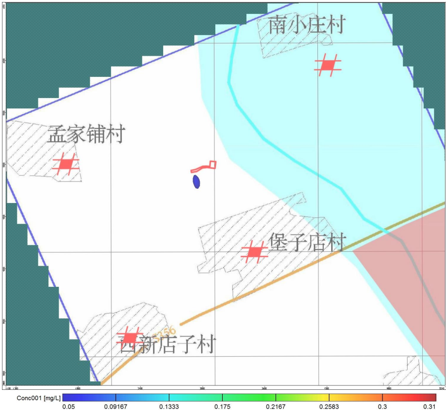
图 5.2-15 铁运移 500 天迁移范围图
