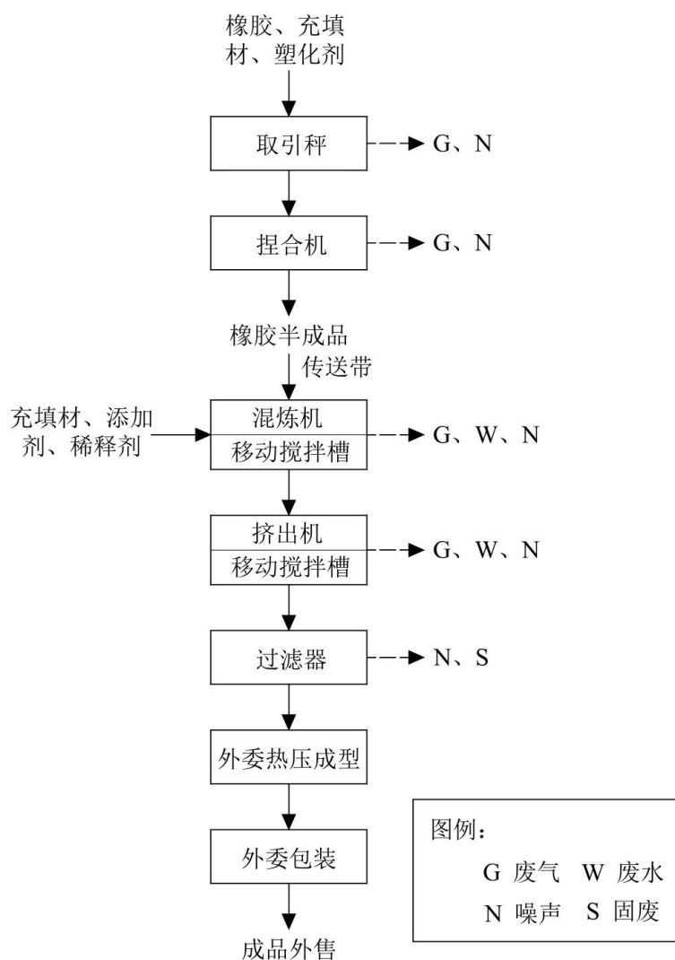
图 14 填充材生产工艺流程及排污节点图
