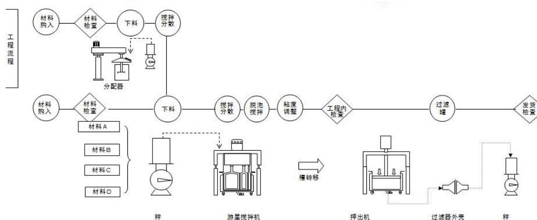
图9 制振材搅拌混合装置示意图
