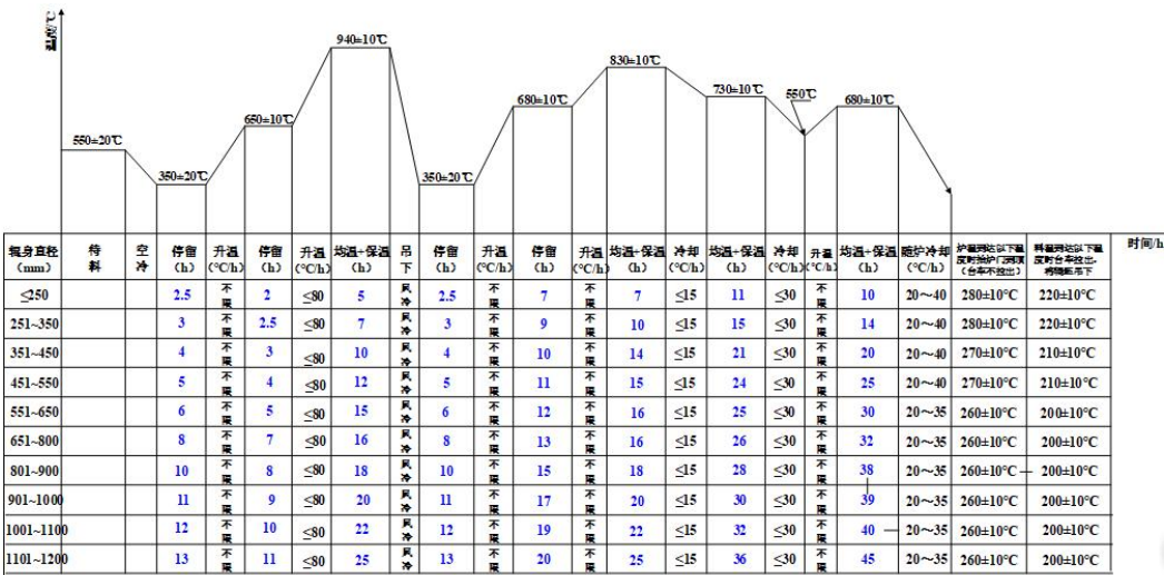
图 2-5 项目锻压车间热处理工艺曲线图
