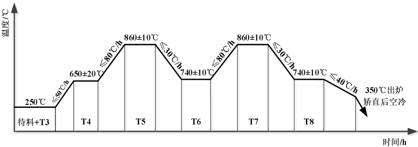
图 2-3 项目不同规格锻件退火工艺曲线图
