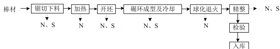
图2-6 盾构机刀圈延链配套产线工艺流程及排污节点图
