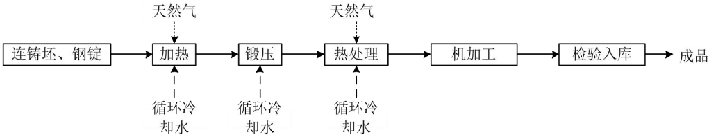
图 2-7 现有工程生产工艺流程图（2 万吨高性能合金钢锻件项目）
