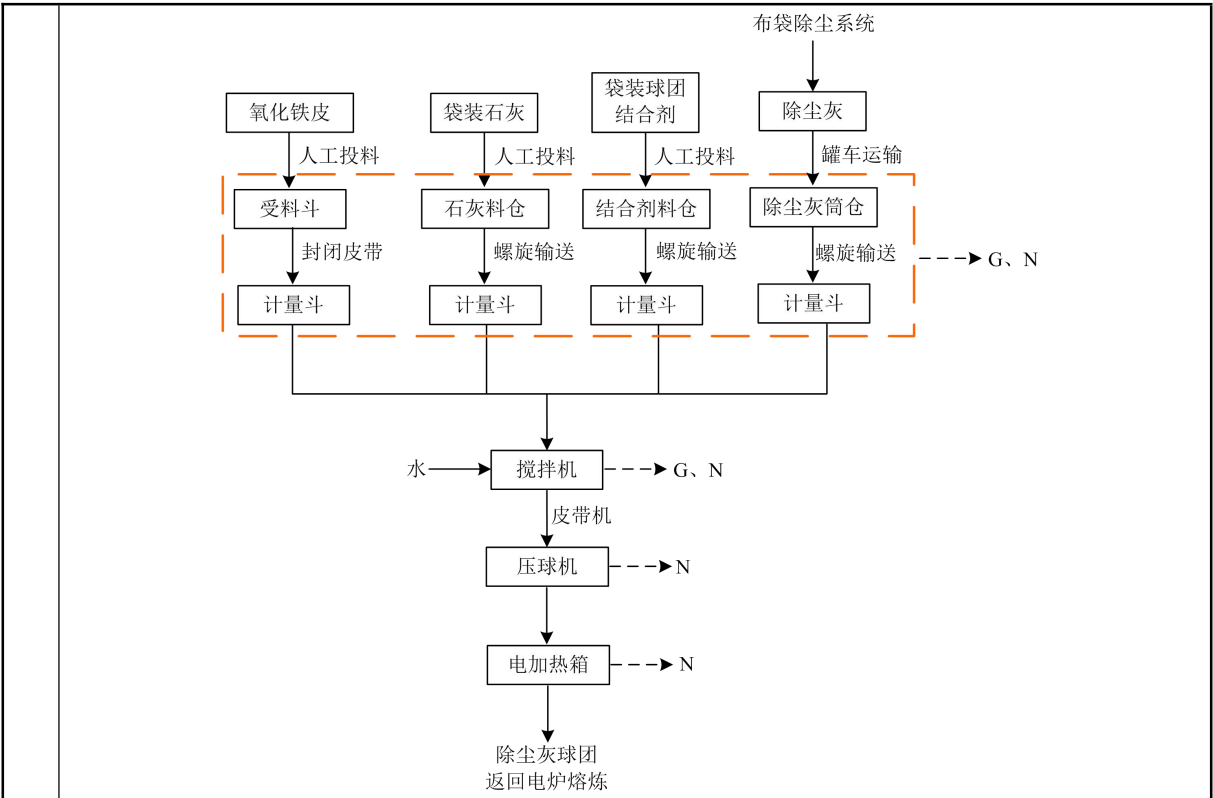
图 2-11 除尘压球生产工艺流程及排污节点图
