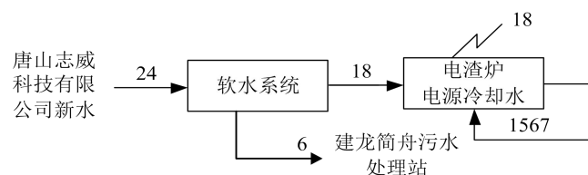
图 2-1 本项目志威科技厂区给排水平衡图 单位： \text{m}^3/\text{d}
