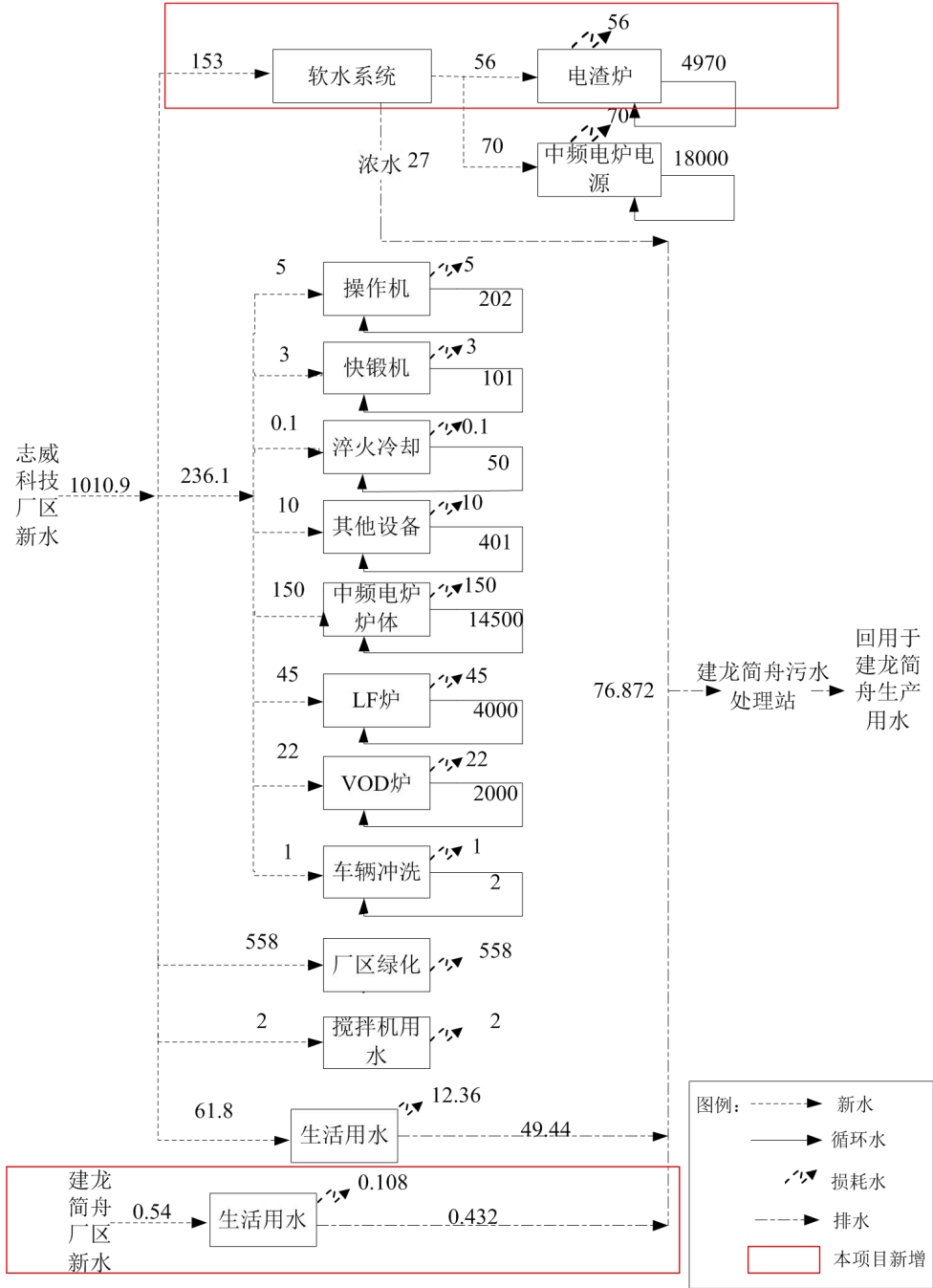
图 2-3 本项目建成后全厂给排水平衡图 单位：m³/d
