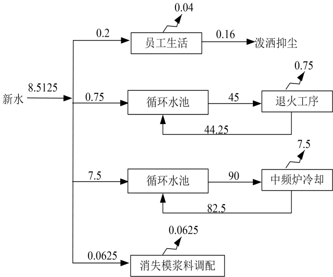
图 4 项目水平衡图 单位 m 3 /d
