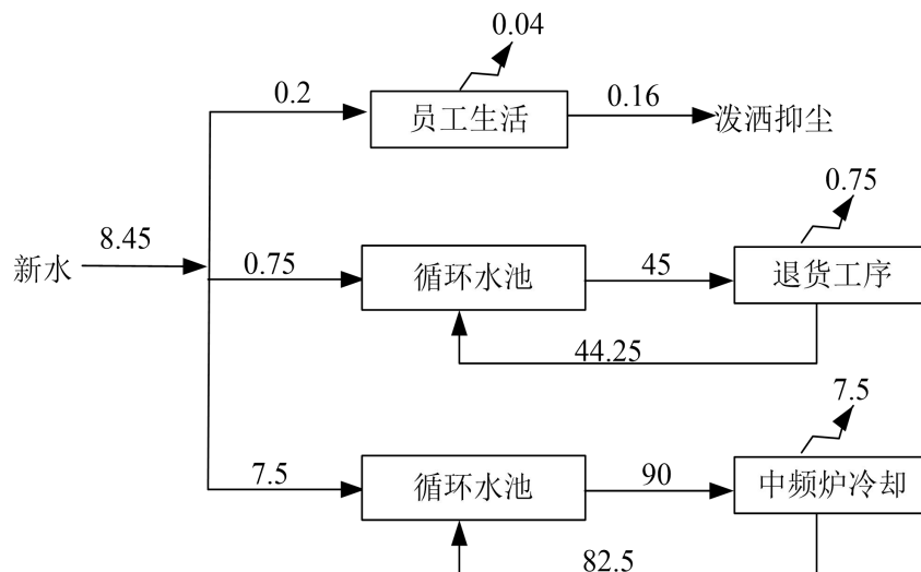
图1 项目水平衡图 单位 m³/d
