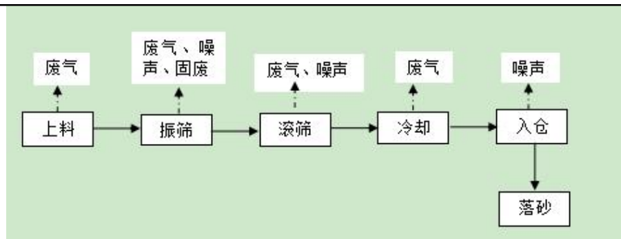
图3 砂处理工艺流程及排污节点图
