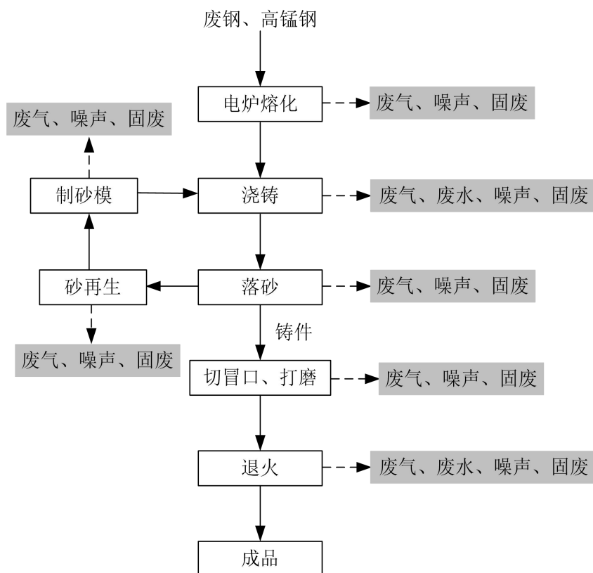
图2 铸造生产工艺流程及排污节点图
