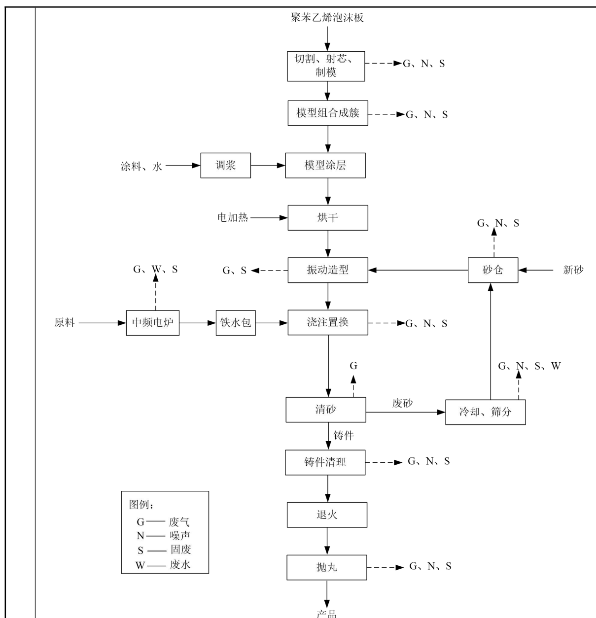
图 5 消失模铸造生产工艺及产排污节点图
