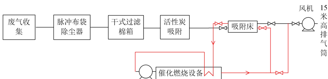
图6 有机废气处理工艺流程图
