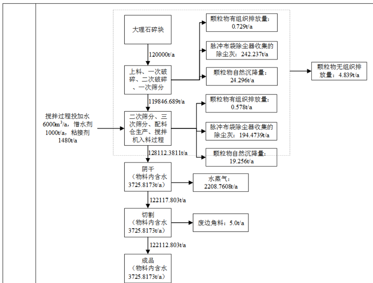
图1 本项目物料平衡图
