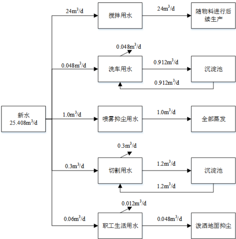
图2 本项目水量平衡图
