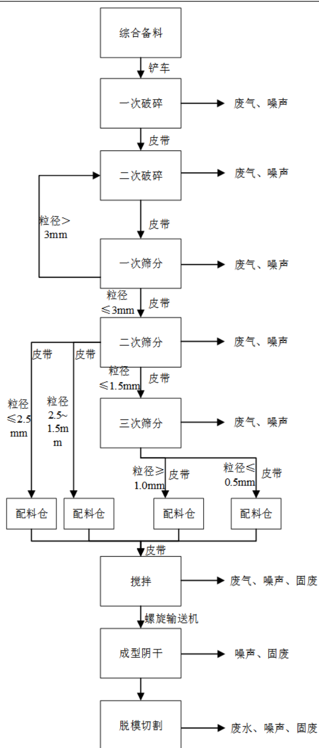
图3 生产工艺流程及产污节点图
