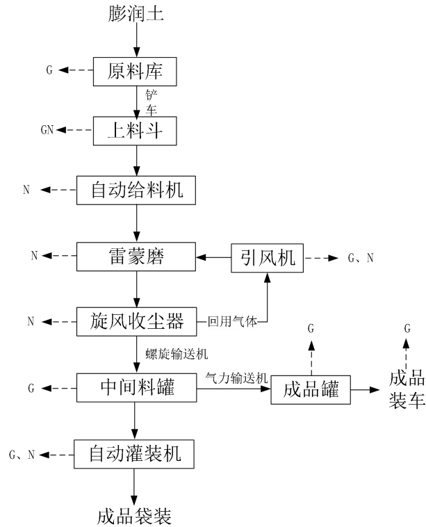
图 2-1 项目生产工艺流程及排污节点图
