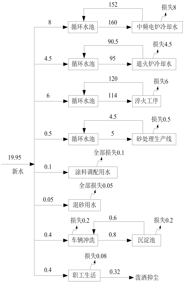
图 2-1 项目水平衡图 单位：m 3 /d
