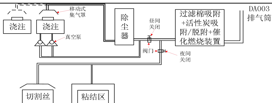
图 4-2 浇注废气收集治理示意图
