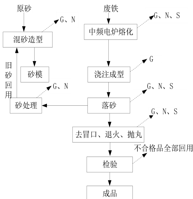
图 2-3 现有工程生产工艺流程及排污节点
