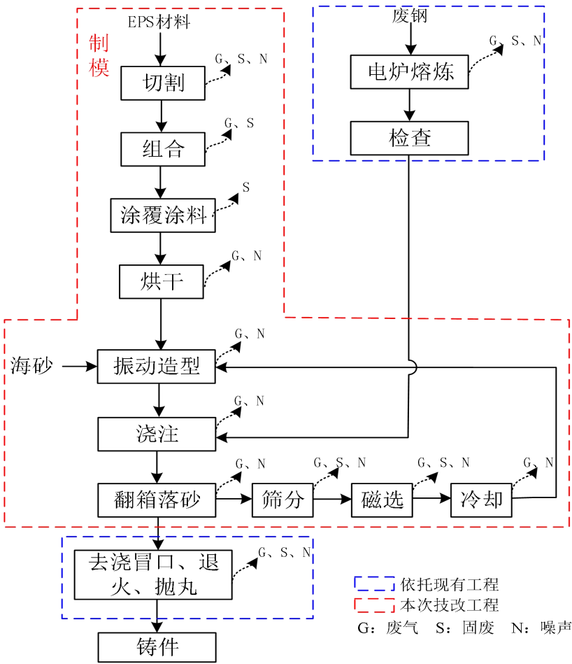
图 2-2 项目工艺流程及排污节点图
