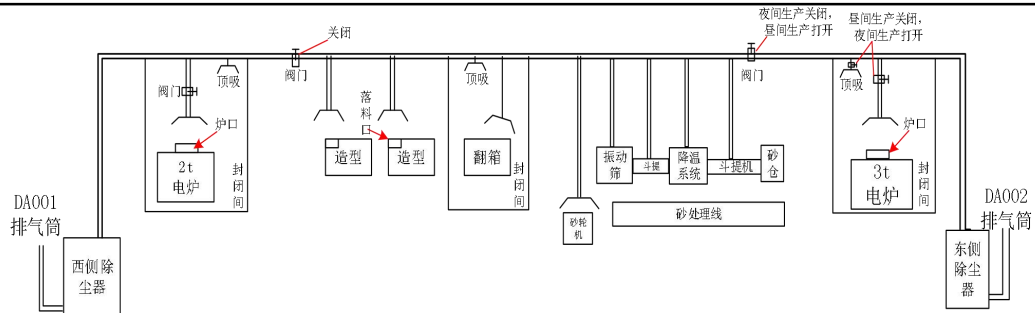
图 4-1 熔炼、造型、落砂/砂处理和去除浇冒口废气收集治理示意图
