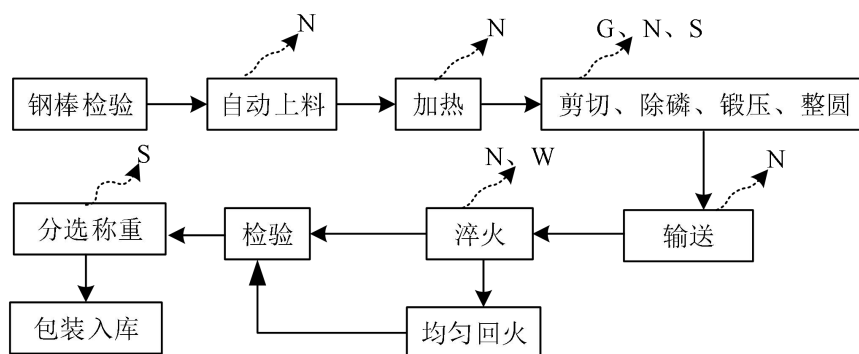
图 2-4 锻压工艺流程及排污节点图
