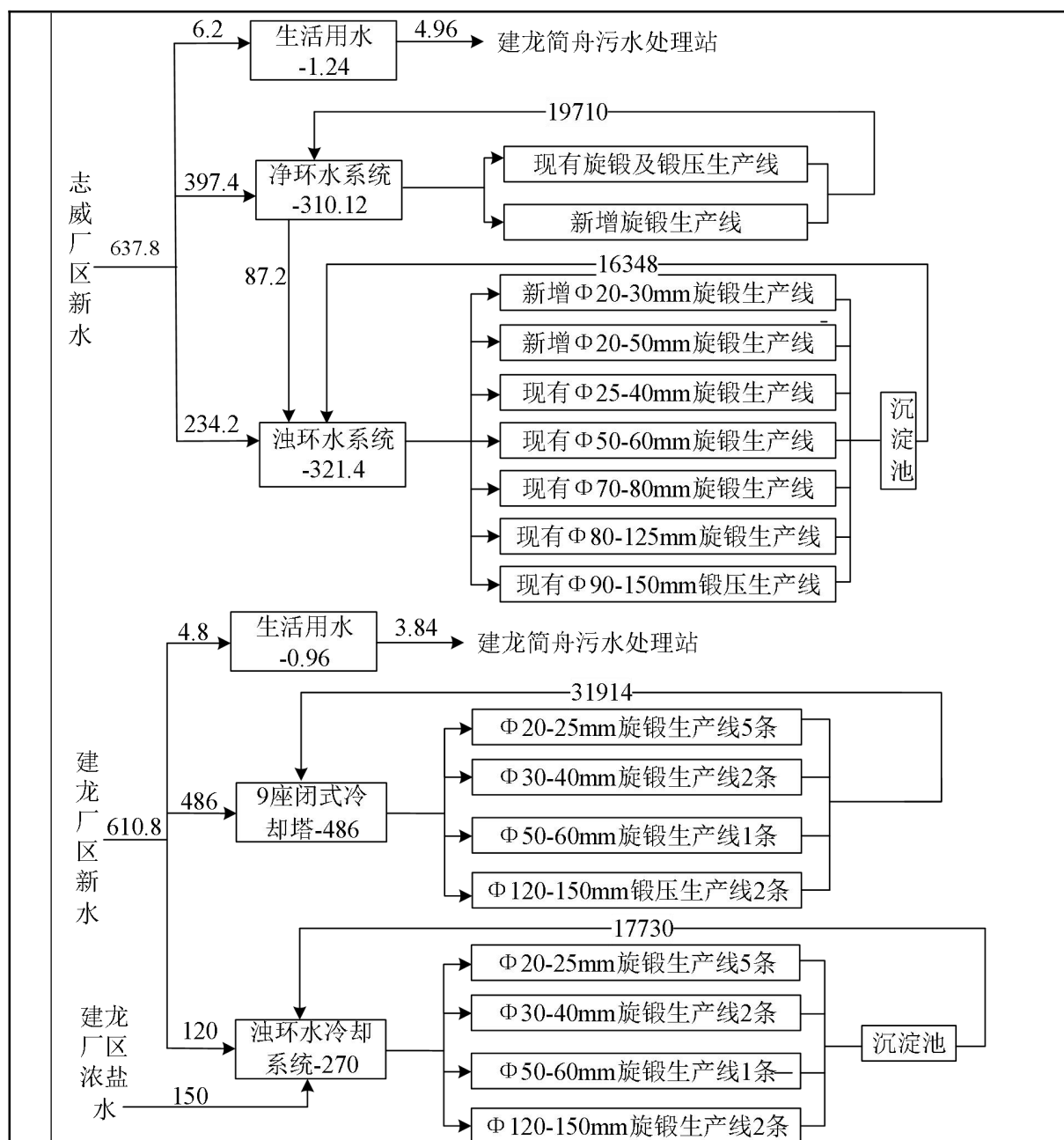
图 2-3 本项目建成后全厂给排水平衡图 单位: \text{m}^3/\text{d}
