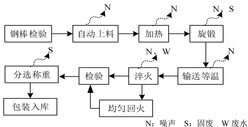
图 2-3 旋锻生产工艺流程及排污节点图
