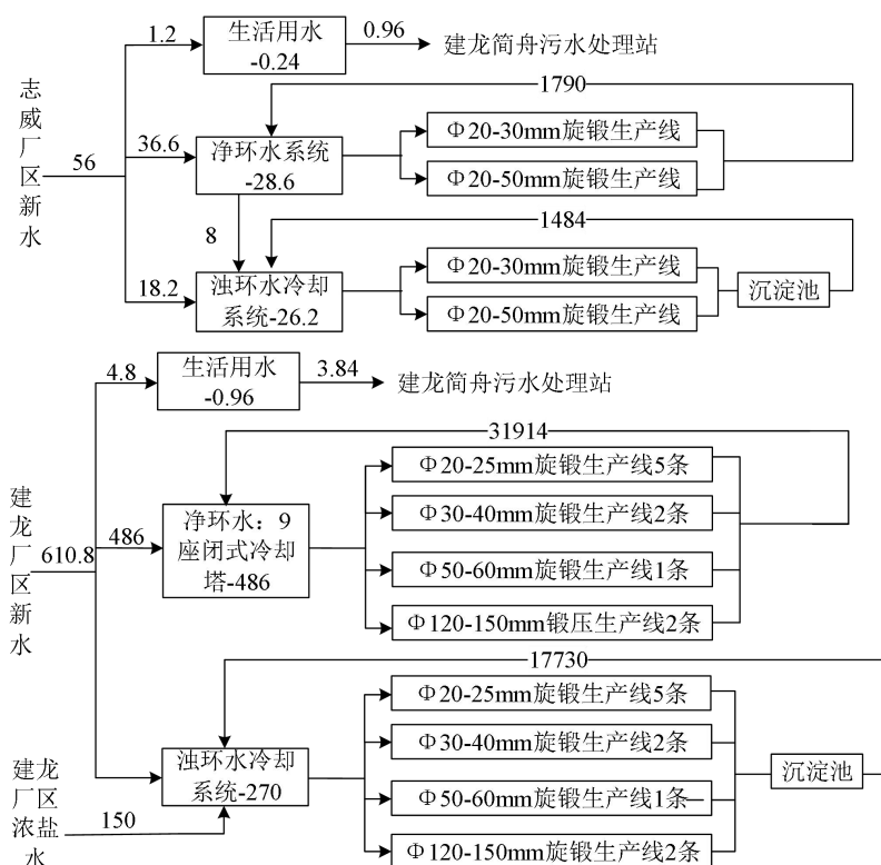
图 2-1 本项目给排水平衡图 单位：m 3 /d
