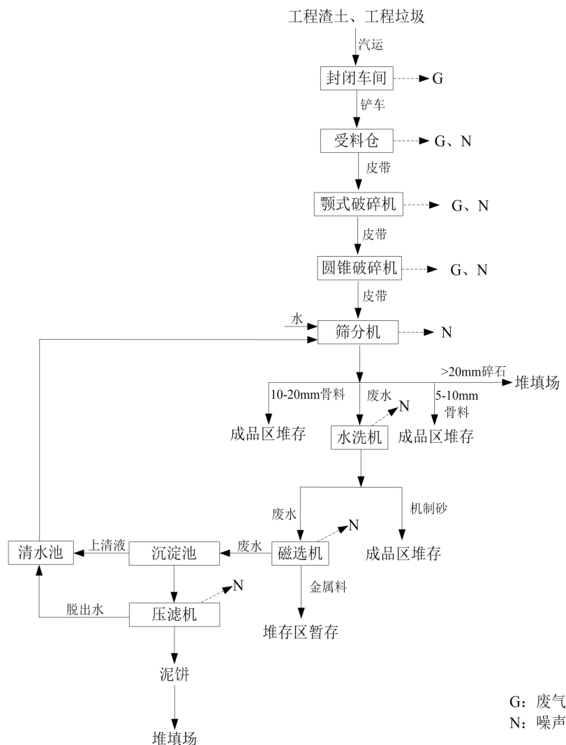
图 2-3 1#生产线工艺流程及排污节点图
